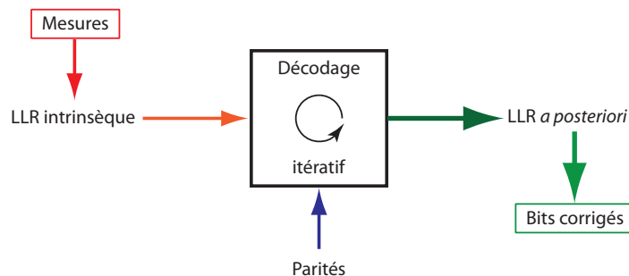
Figure 7.3 : Schéma de principe d'un décodeur mou.
