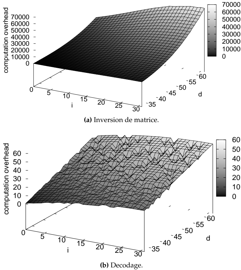
Figure A.9: Computation overhead pour la reconstruction pour RC(32, 32, d, i) .
