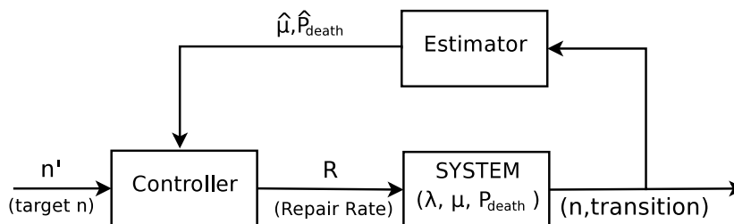
Figure A.11: Le schéma de contrôle adaptatif
