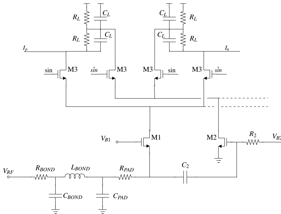
Figure 9: Schéma du BLIXER conçu [2].
