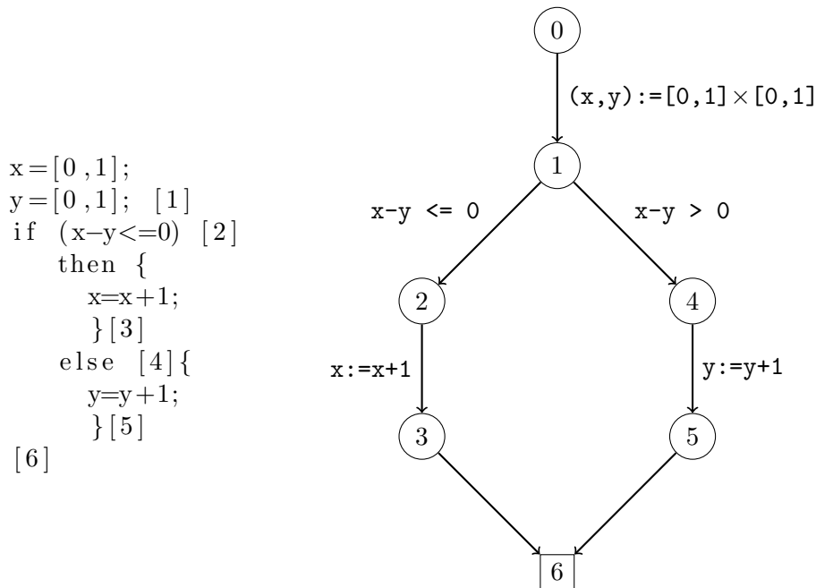
Figure 2.4 – Un programme avec un branchement conditionnel à gauche et son graphe de flot de contrôle
