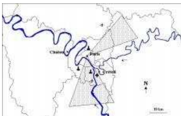
Figure II.11 : Origine des masses d'air sur le site de Paris du 09/12/96 au 19/12/96
