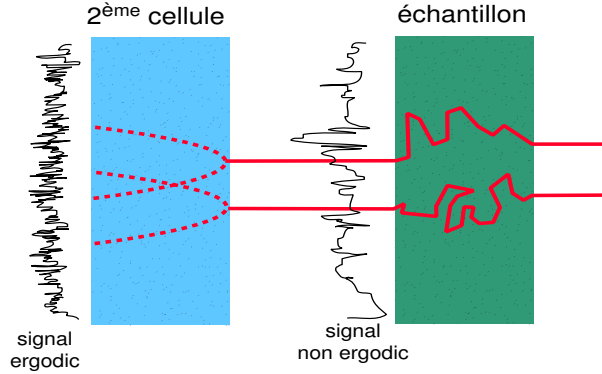
Fig. 2.11: Représentation schématique du principe de double cellule. Le signal non ergodique émergeant de l'échantillon traverse la deuxième cellule. Les traits pointillés représentent l'enveloppe de la lumière entrant en C ou D et diffusant dans la deuxième cellule (approximation DWS). Dans la zone de recouvrement des deux paraboles les lumières des points C et D interfèrent conduisant à une moyenne spatiale du signal non ergodique.
