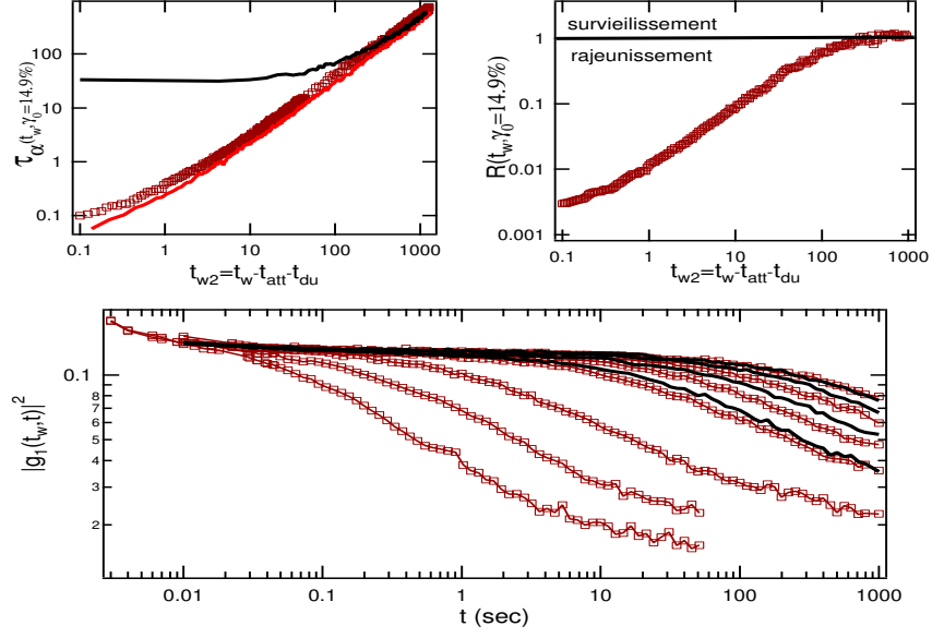
Fig. 3.11: a) Temps caractéristique de décroissance après un cisaillement de 14.9% pendant 100s en fonction de t_{w2} : trait plein noir: \gamma = 0\% :trait grisé, \gamma = 14.9\% : \square b) Rapport R en fonction de t_{w2} . c) Faisceau des fonctions de corrélation après le cisaillement ( \square ) pour des t_{w2} = 0.13s, 1.25s, 5s, 60s, 165s, 467s, 1212s ; et pour un cisaillement nul (trait plein) pour des temps t_{w2} = 1s, 180s, 500s, 1212s .
