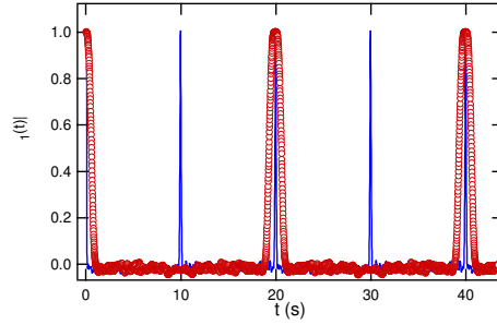
Fig. 9.3: Fonctions de corrélation sous cisaillement pour un gel de gélatine avec traceurs. La fréquence utilisée est 0.1Hz. Pour une phase \bar{\phi} = \frac{\pi}{2} (○), on voit que la fonction présente un écho toutes les périodes. Pour une phase \bar{\phi} = 0 (trait plein), il y a doublement de la fréquence. Notons aussi que la forme et la largeur des échos dépendent considérablement de \bar{\phi} .
