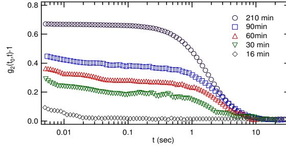
Fig. 2.9: Fonctions de corrélation non normalisées obtenues avec la caméra après la trempe d'un gel de gélatine de 60°C à 20°C. Remarquez la croissance de l'intercept indiquant la présence d'une décorrélation aux temps courts.
