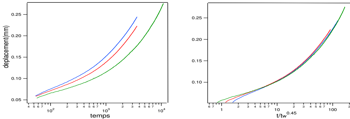
Fig. 5.7: a) Vieillissement de la complaisance pour des âges t_w = 30min\ 60min\ 180min b) remise à l'échelle des courbes par le facteur \frac{t}{t_w^{0.45}} . La température est T=30^\circ C .
