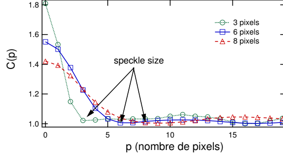
Fig. 2.4: Mesure de C(p) pour différentes ouvertures du diaphragme. La taille du grain speckle correspond au premier minima de la fonction C(p) [56]
