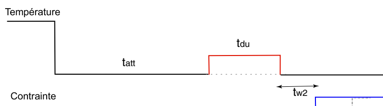
Fig. 5.1: Principe du protocole appliqué aux polymères vitreux. En haut: histoire de la température; en bas: histoire de la contrainte.
