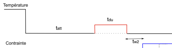
Fig. 5.5: Principe du protocole appliqué aux polymères vitreux. En haut histoire de la température, en bas histoire de la contrainte.
