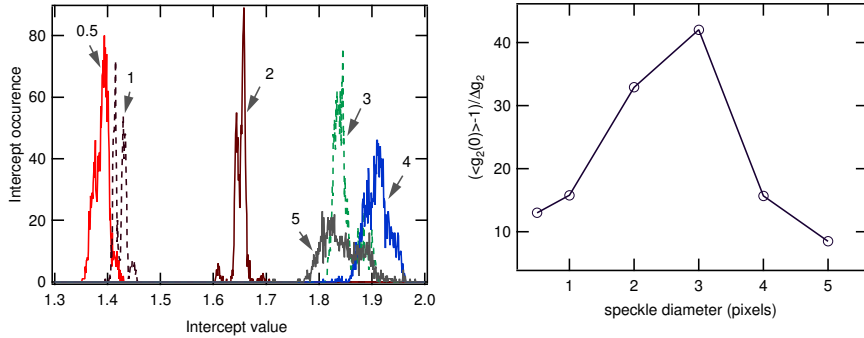
Fig. 2.5: (a) Histogramme des intercepts pour différentes tailles de speckle (0.5, 1, 2, 3, 4, 5 pixels) comme indiqués sur la figure. L'intercept théorique est 2. Notez la croissance de la valeur de l'intercept avec la taille (meilleur contraste) ainsi que celle de la dispersion (moins bonne statistique). (b) rapport "signal sur bruit" \langle(g_2(0,0) - 1)\rangle/\Delta g_2 montrant que le meilleur compromis est obtenu pour une taille de 3 pixels.[56]
