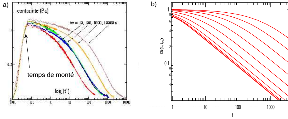
Fig. 8.2: a) Module de relaxation mesuré sur une solution concentrée de billes de silice. Remarque le temps de monter de l'appareil aux temps courts. b) Module de relaxation calculé à partir du modèle SGR. L'axe des temps a volontairement été tronqué à t_{min} = 1s . On a alors l'impression d'une dérive de la valeur du module à l'origine. Cette dérive est un simple effet d'une gamme de temps d'observation finis.
