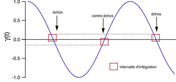
Fig. 9.13: Représentation schématic de l'effet de disymétrie généré par le temps fini d'intégration de la caméra. La fréquence d'acquisition CCD doit être un multiple de la fréquence de cisaillement pour minimiser cet effet tant sur l'échos que sur le contre échos.
