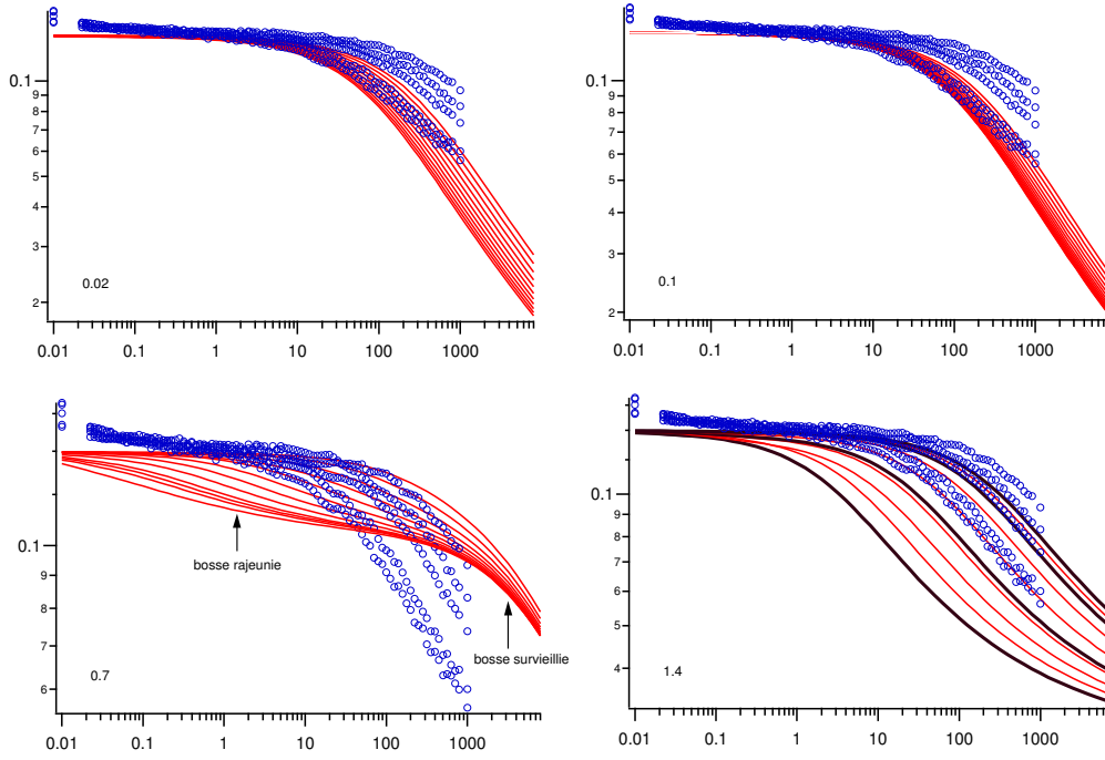
Fig. 7.2: Différents essais de fit pour un cisaillement de 2.9%. Les différentes amplitudes de cisaillement théoriques sont \gamma_0^2 = 0.02, 0.1, 0.7, 1.4 . La présence d'une double bosse dans la fonction de distribution semble ne pas convenir quantitativement au changement de forme de la fonction de corrélation.
