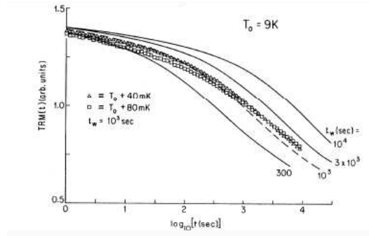
Fig. 4.6: Illustration de l'effet de survieissement sur un verre de spin [13]. Les courbes en trait plein et pointillé sont les courbes de vieillissement simple. Les courbes en symbole sont les fonctions de relaxation suivant la petite marche en température positive. La courbe pour \Delta T = 80mK montre clairement une décroissance plus rapide à temps court et plus lente à temps longs.
