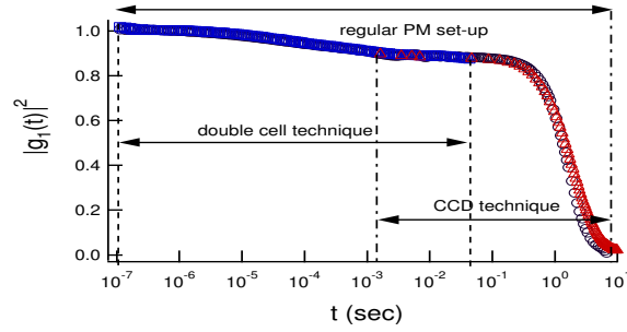
Fig. 2.16: Superposition des fonctions de corrélation obtenues par les trois techniques (PM seul (o), Double cellule ( \square ), caméra ( \triangle ) sur un gel de gélatine pour t_w = 300 min. La légère différence observée aux temps longs est attribuée à un temps de mesure trop faible pour la technique PM seul (3600s). Le temps d'acquisition des données est de 100 s pour la double cellule et de 10s pour la caméra.
