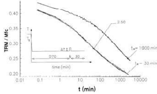
Fig. 4.5: Effet de rajeunissement mesuré sur les courbes de relaxation TRM (ref) pour une marche positive en température. La courbe mesurée 30 minutes après la marche thermique se superpose avec la courbe mesurée 30 minutes après la trempe. Il y a donc rajeunissement total.[6]
