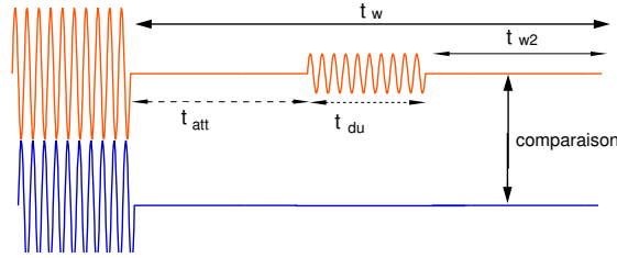
Fig. 3.9: Illustration du protocole expérimental. La schéma du haut représente le protocole de perturbation et le schéma du bas le protocole de référence. Les différents temps sont définis sur la figure.
