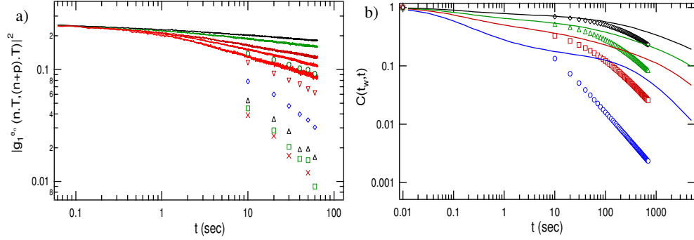
Fig. 9.10: a) Comparaison des fonctions g_1^{en}(n.T, (n+p).T) (symboles) et des fonctions de décroissance spontanée (trait continu). Les cycles de référence sont les cycles numéro 2 ( \times ), 4 ( \square ), 6 ( \triangle ), 10 ( \diamond ), 30 ( \nabla ), 100 (O) de bas en haut pour les fonctions en traits pleins. L'amplitude du cisaillement est de 5.5%. La dynamique spontanée est systématiquement plus lente que la dynamique forcée. b) Même courbes calculées à partir du modèle SGR. L'amplitude du cisaillement est \gamma_0^2 = 20 . Les cycles de référence sont les cycles numéro 1 (O), 10 ( \square ), 30 ( \triangle ), 100 ( \diamond ). On observe un bon accord qualitatif.
