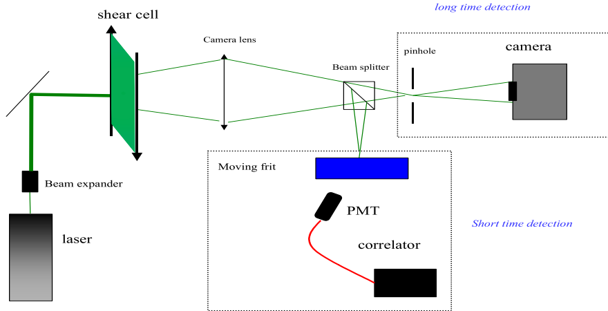
Fig. 2.12: Montage expérimental de l'acquisition temps courts/temps longs.
