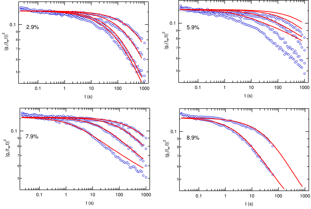
Fig. 7.3: Superposition Des faisceaux de courbes pour différentes amplitudes de cisaillement (2.9%, 5.9%, 7.9%, 8.9%) fittés par les courbes théoriques calculées pour un \Delta T de resp 0.1, 3, 4.5, 6.2. Pour toutes les valeurs du cisaillement sauf pour 5.9% les fits semblent acceptables, pourtant le temps écoulé entre chaque courbes théoriques ne correspond pas au temps écoulé entre chaque courbes expérimentale. Le fit est donc forcé.
