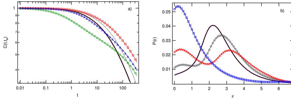
Fig. 6.15: a) Fonction de corrélation C après cisaillement \gamma_0^2 = 6.2 (symboles) et de référence (trait plein) et pour des temps t_{w2} = 0 ( \circ ) (resp trait gras), 6 ( \triangle ), 50 ( \square ) (resp trait fin). Le fort croisement des courbes pour les petits t_{w2} correspond à une forte surpondération des temps courts qui s'équilibrent vite pour ne plus laisser apparaître que la surpondération aux temps longs. b) Distributions P pour différentes amplitudes de cisaillements \gamma_0^2 = 0 (trait plein) 2.9 \circ , 6.2 \triangle , 20.25 \square . Toutes les courbes sont calculées pour t_{w2} = 0 . On remarque séparation en deux bosses de la distribution.
