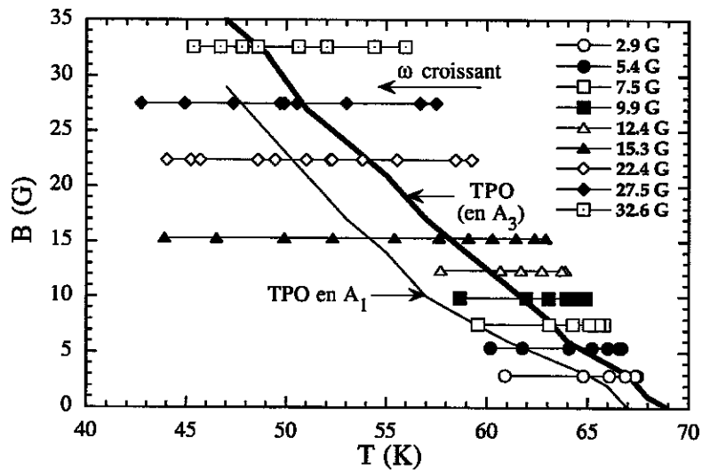
FIG. 4.22 – Localisation des points de mesure de r_w dans le diagramme de phase ( B, T ) des échantillons étudiés. La TPO repérée par MOD au point A_3 est indiquée par la ligne en gras, une ligne simple repère la TPO en A_1 (voir fig. 4.14). Les points dans le liquide de vortex vérifient \langle \cos \phi_{n,n+1} \rangle < 0.5 , en accord avec le saut de \langle \cos \phi_{n,n+1} \rangle de 0.7 à 0.3, observé à la TPO par d'autres auteurs [51, 52]. Pour un champ donné, la fréquence JPR des points de mesure augmente quand la température diminue (flèche " \omega croissant").
