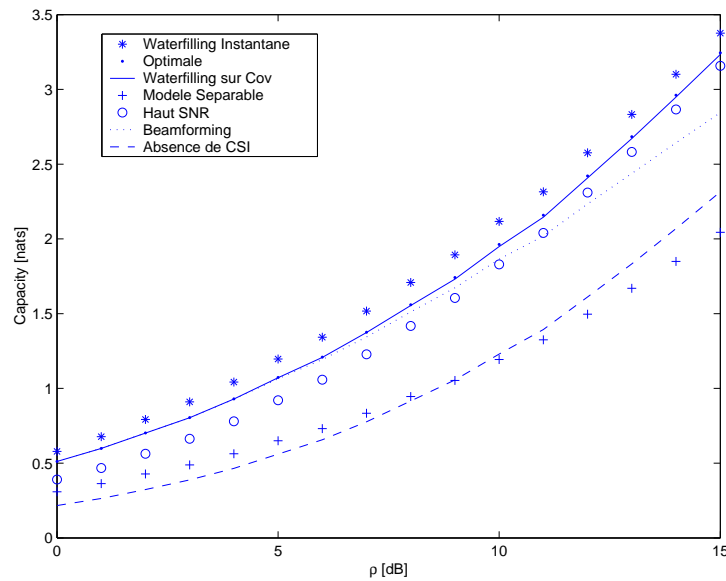
Figure 7.22: Modèle à chemins, N_{tx} = N_{rx} = 4 , L_p = 2 .
