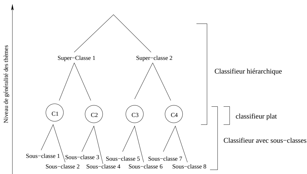
FIG. 5.1 – Opposition entre classifieurs hiérarchiques et classifieurs avec sous-classes. Les catégories à discriminer sont les ensembles C1 , C2 , ..., C4 . Un classifieur “plat” n’utilise que cette information pour faire la classification. Un classifieur hiérarchique utilise des regroupements de classes en ensemble plus généraux alors qu’un classifieur avec sous-classes détermine des sous-ensembles plus précis de chaque classe.
