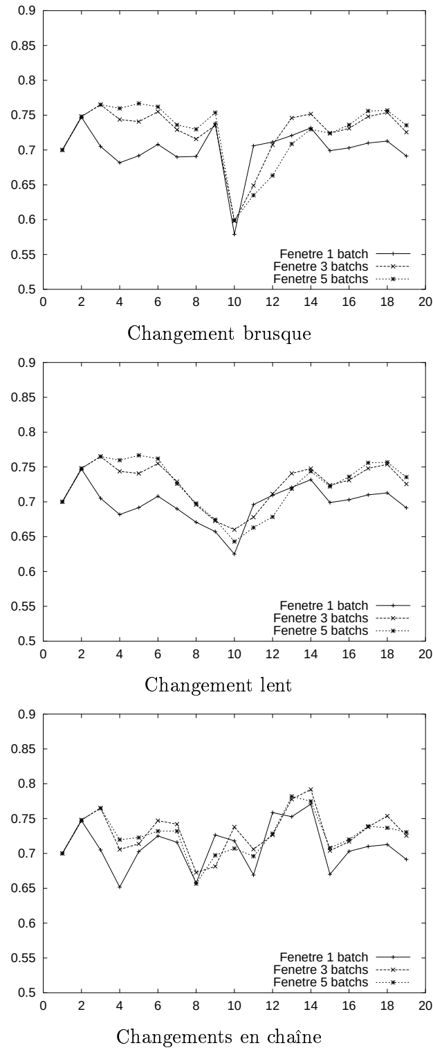
FIG. 6.4 – Comportement de Rocchio en fonction de la taille de la fenêtre pour les trois types de changements.
