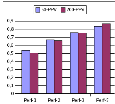
FIG. 4.5 – Expériences supplémentaires avec k-PPV
