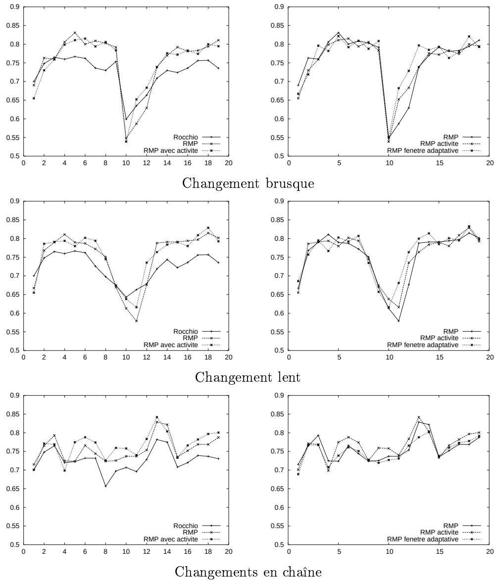
FIG. 6.5 – Comparaison entre Rocchio, RMP, RMP avec taux d'activité et RMP avec fenêtre adaptative.
