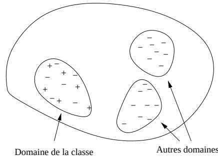
FIG. 2.2 – Interprétation géométrique du Query Zoning . Seuls les éléments négatifs du domaine doivent être pris en compte.
