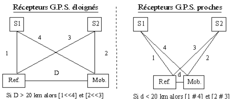
Figure 3 : correction différentielle
