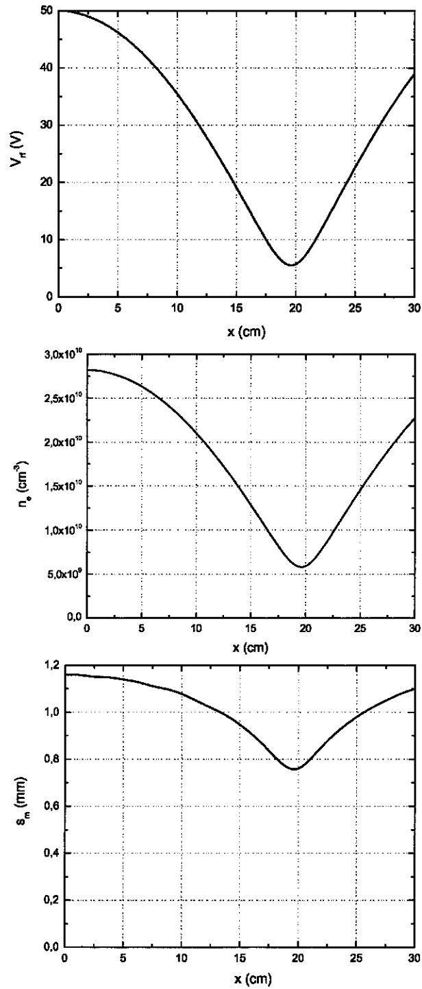
FIG. 3.10 – Profils radiaux de potentiel, de densité et de taille de gaine calculés par le modèle ligne de transmission (150 mTorr, V_0 = 200 V, gap 3 cm, 81.36 MHz)
