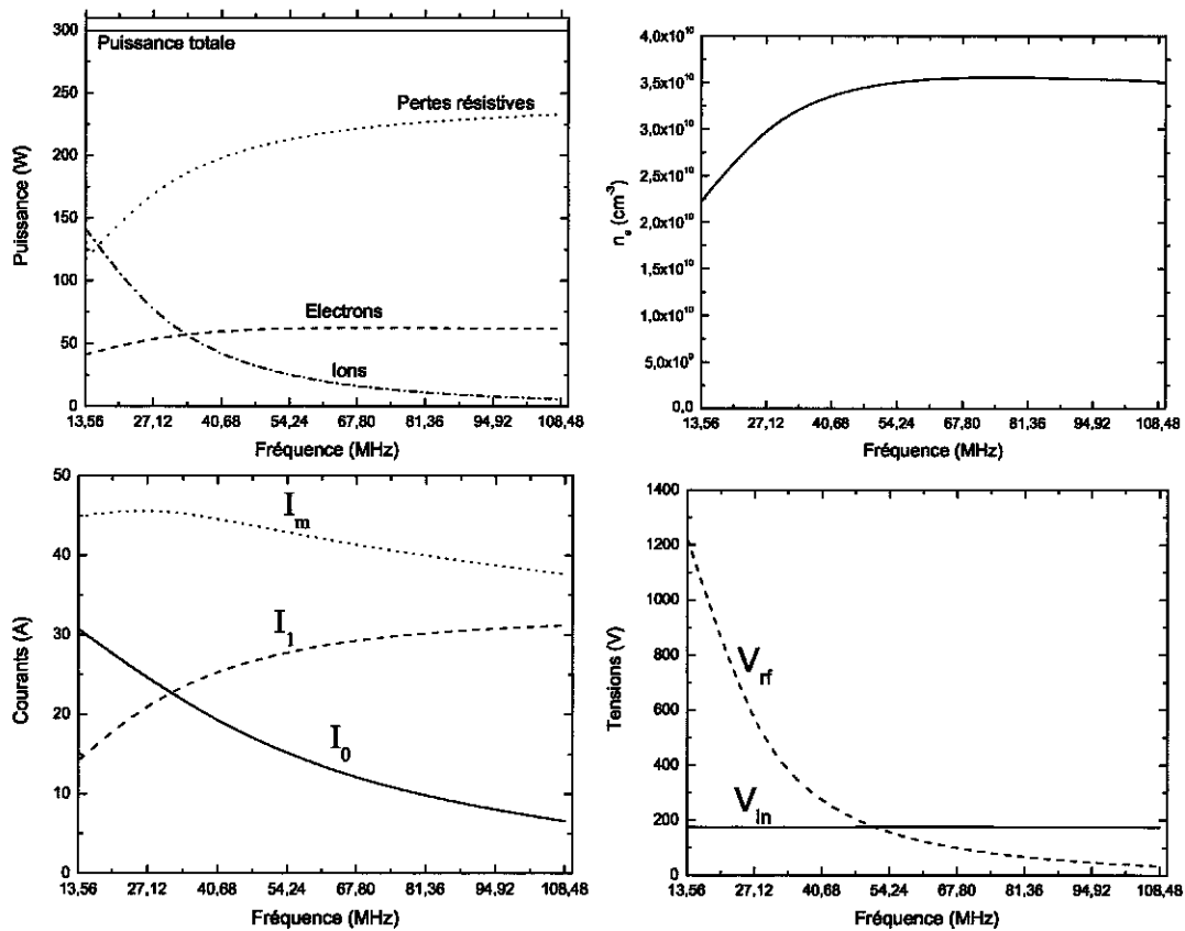
FIG. 2.11 – Puissances dissipées, densité d'électrons, courants et tensions en fonction de la fréquence pour P_{in} = 300 \text{ W} , R_m = f(\sqrt{\omega}) , 150 mTorr, gap 3 cm
