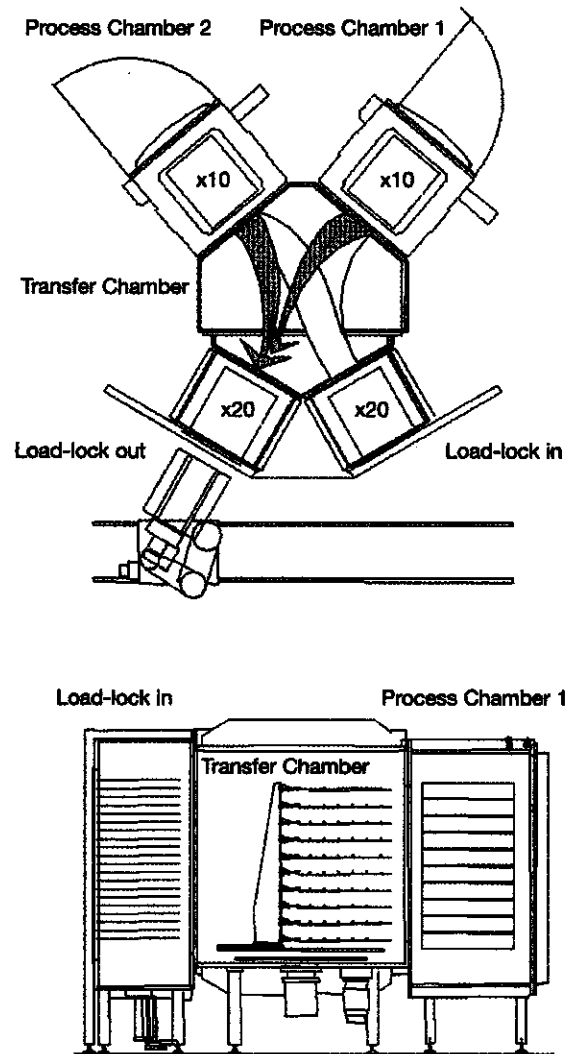
FIG. 4.4 – Vue de dessus et vue de côté d'un système industriel avec réacteurs en parallèle (source : Unaxis)
