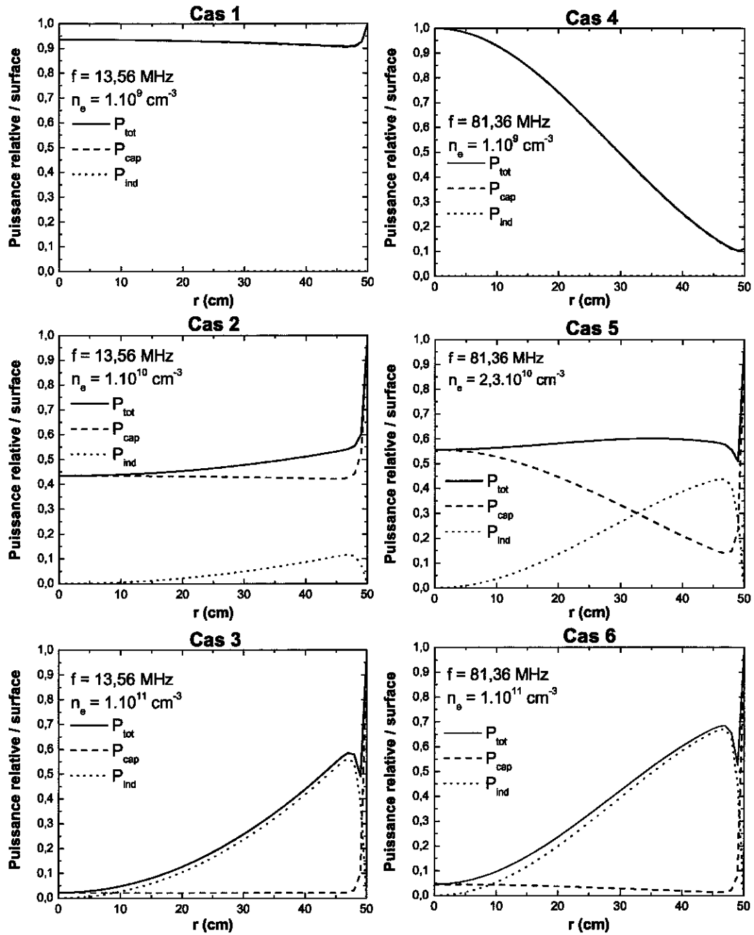
FIG. 3.6 – Profil du dépôt de puissance radiale pour différentes conditions de décharge (décharge cylindrique, rayon 50 cm, gap 3 cm, 150 mTorr) s_m = 8 mm. r = 0 correspond au centre des électrodes.
