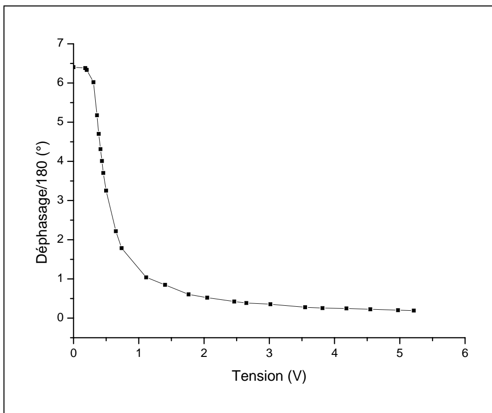
Figure 3.8 : Déphasage en fonction de la tension appliquée aux contrôleurs pour un cristal liquide nématique Jenoptik PLM 220 mm ( \lambda = 632.8 \text{ nm} ).
