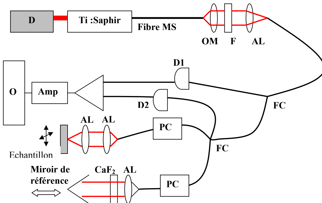
Figure 1.2 : OCT à fibres du MIT, USA.
