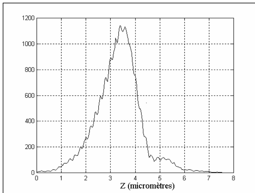
Figure 1.13 : Enveloppe des franges d'interférences ( \sqrt{S_{\text{int}}} ) en fonction de la position axiale Z sur la lame en verre inclinée. La largeur à mi-hauteur vaut 1,4 \mu\text{m} .
