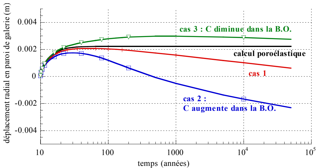
Figure VI-30 : Evolution au cours du temps du déplacement radial en parement de galerie (massif élastoviscoplastique).
