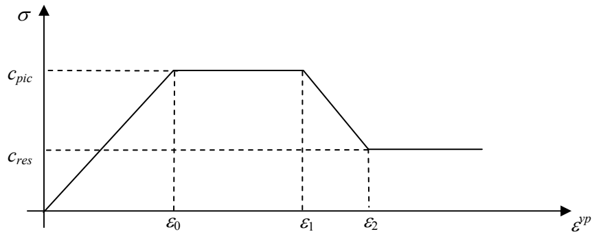
Figure III-18 : Variation du seuil viscoplastique avec le paramètre d'écroissage
