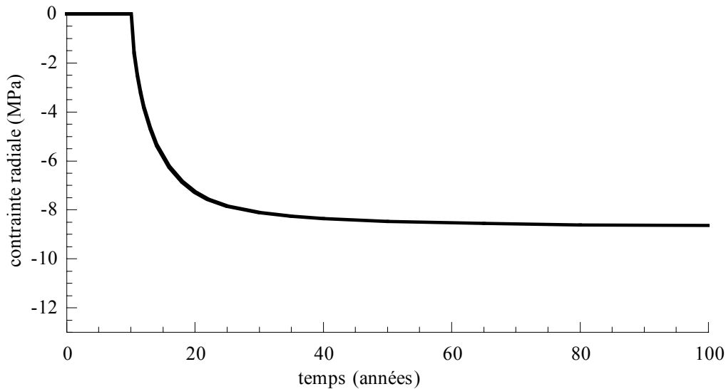
Figure VI-11 : Evolution de la contrainte radiale dans la B.O. (à r = 0,8 R_j ).
