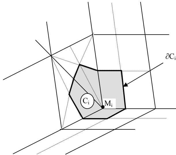
Figure D-1 : Cellule du nœud M_i dans le cas d'une approximation par éléments finis P1 dans Anthyc.
