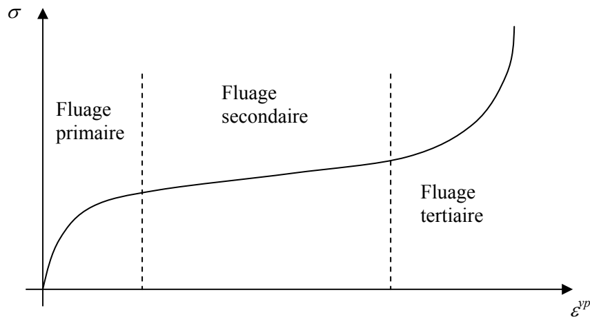
Figure III-6 : schéma d'une courbe de fluage monophasier présentant les trois phases de fluage.
