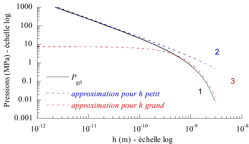
Figure IV-7 : Pression de gonflement calculée pour \Gamma=0,1C/m^2 et C=0,1M .
