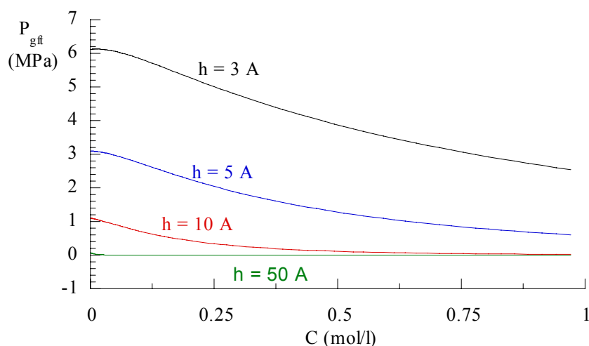
Figure IV-15 : Evolution de P_{\text{gft}} en fonction de C pour plusieurs mi-distances h entre feuillets.
