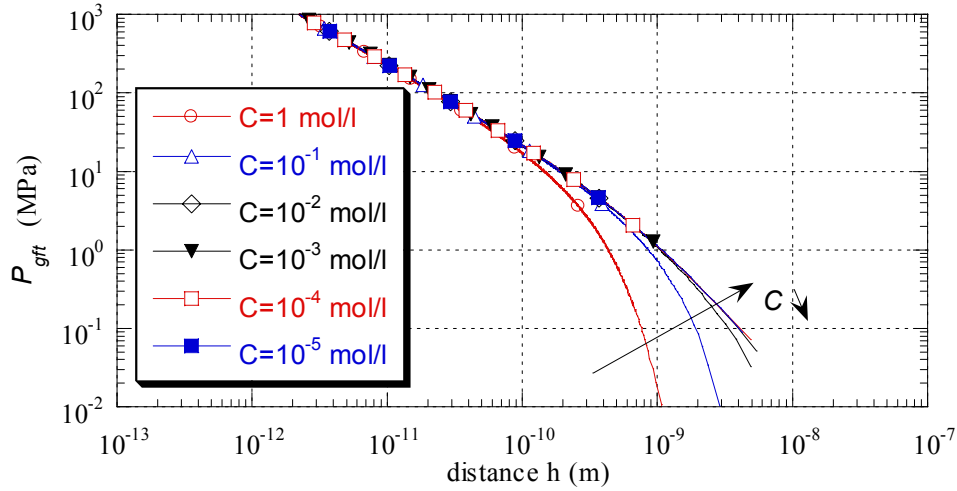
Figure IV-12 : Pression de gonflement en fonction de la mi-distance h , dans le cas d'une charge surfacique \Gamma = -0,1 C/m^2 et pour différentes concentrations entre 1 \text{ mol/l} et 10^{-5} \text{ mol/l} .
