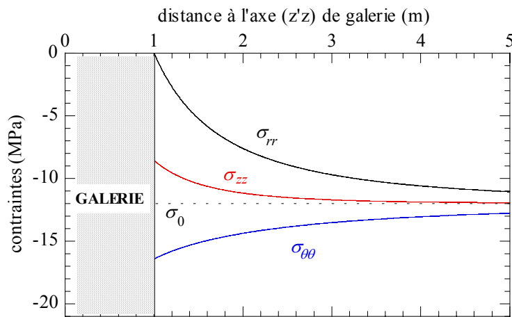
Figure III-16 : Contraintes principales après 100 ans avec la loi de comportement viscoplastique des argilites de l'Est (avec les paramètres de la loi de 1999).
