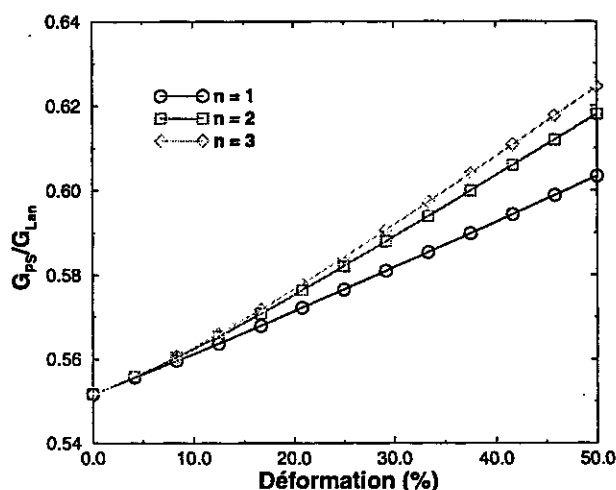
FIG. 15.2-9: Rapport des taux de restitution d'énergie des éprouvettes PS et lanières aux faibles déformations macroscopiques.
