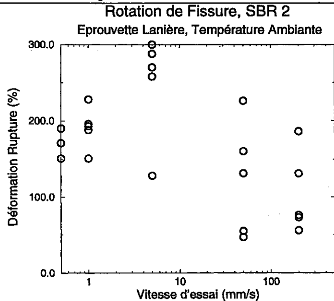
FIG. 1.1-8: Essai de traction uni-axiale sur des éprouvettes lanières pré-entallées d'un SBR (SBR 2) chargé. Test réalisé à l'ambiante. Pour chaque vitesse, 5 essais sont réalisés. On observe d'abord une forte dispersion des résultats et la présence d'un optimum de la déformation à rupture, plutôt mal défini dans cet essai mais localisable à 5 mm/s.
