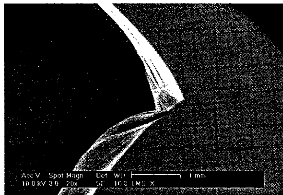
(b) Branchement d'une fissure déviée (en haut) sur une propagation en moustache (en bas).
