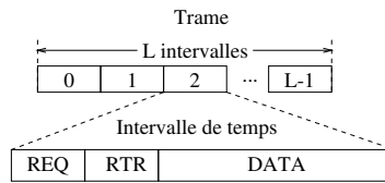
Figure 7: La structure de trame de CROMA.
