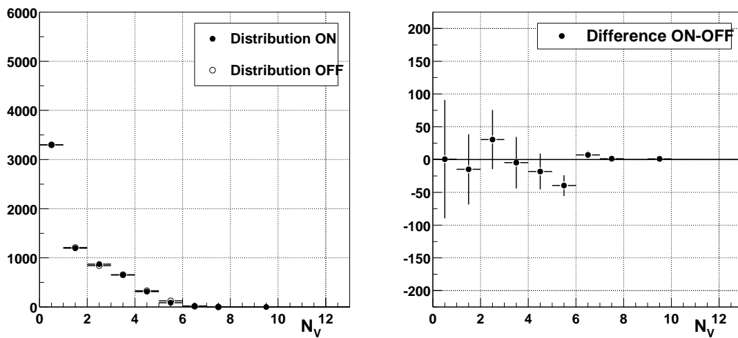
FIG. 10.12 . Distributions de \mathcal{N}_V pour les données IES1426+428 ( \xi_{\text{cor}} < 0.40 ). À gauche : distributions ON et OFF de la variable \mathcal{N}_V pour les données IES1426+428 après coupure sur \xi_{\text{cor}} ( \xi_{\text{cor}} < 0.40 ). À droite, différence ON-OFF de ces mêmes distributions.
