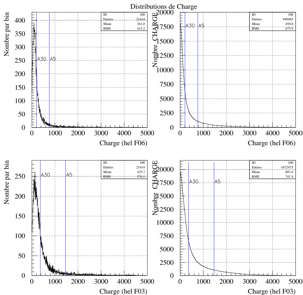
FIG. 4.10. Spektr en charge. À gauche : Spektr en charge pour deux héliostats pour un run. À droite : Ces mêmes spektr en charge sont intégrés par la droite. Les lignes A30 et A5 indiquent les limites à 30% et 5% respectivement.
