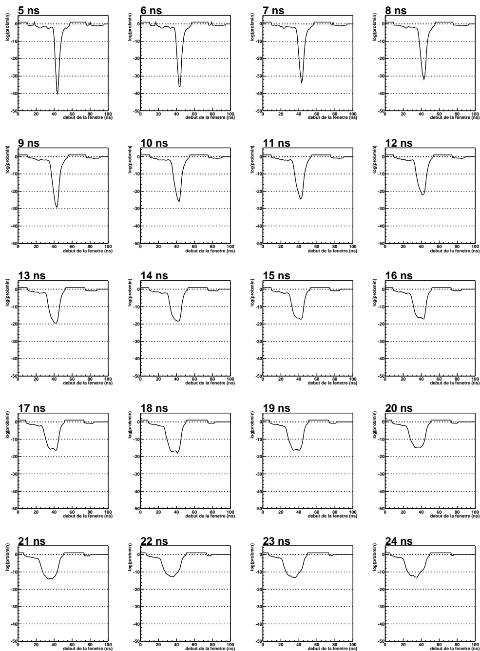
FIG. 7.6 . Recherche de la fluctuation maximale (1). Ci-dessus : Exemple d'un événement à un pic. Les deux premières courbes correspondent à \ln p_w^{min} et t_w^{min} . Ci-dessous : Ensemble des courbes \ln p_w^i pour cet événement.
