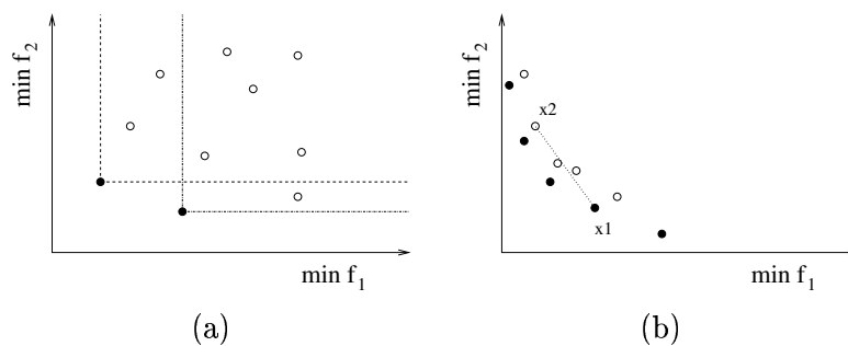
FIG. 6.1 – Situation typique: (a) au tout début de l'évolution, il y a peu d'individus non-dominés mais chacun d'eux domine beaucoup d'individus; (b) au bout d'un certain nombre de générations, la population est constituée de moins de fronts et chaque non-dominé domine très peu d'individus
