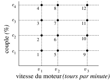
FIG. 8.5 – Un exemple de carte des régimes du moteur ( engine map ) avec 12 points de contrôle
