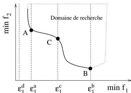
FIG. 1.5 – Illustration de l'approche de \epsilon -contraintes
