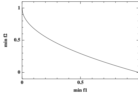
FIG. A.1 – Solution de ZDT1
