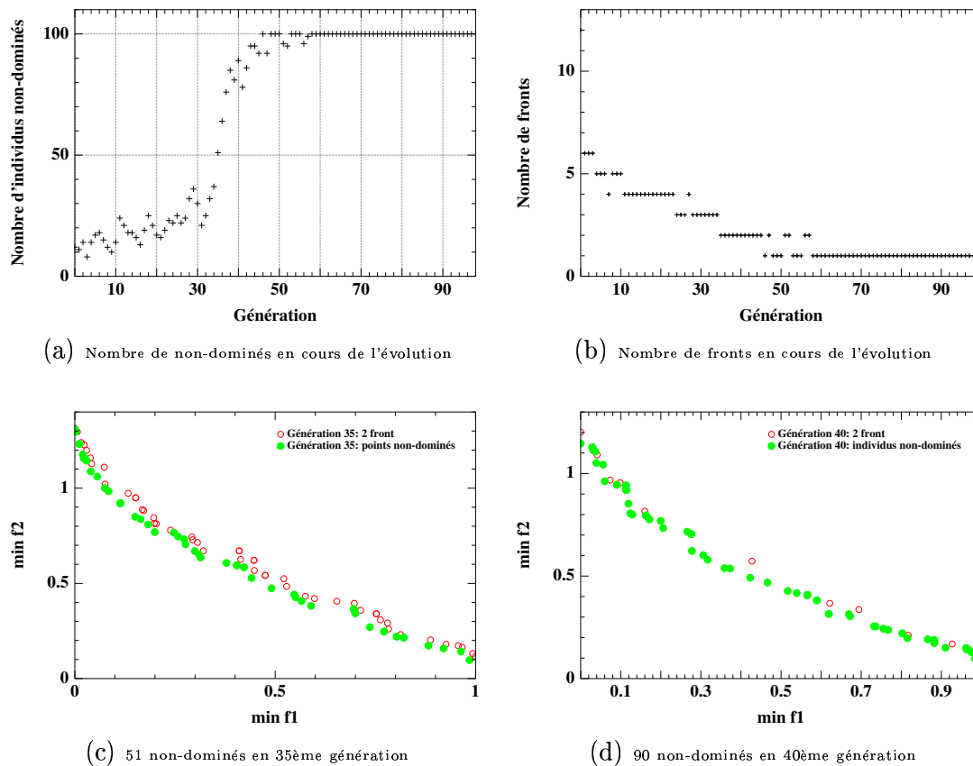
FIG. 6.6 – La moitié de la population rejoint l'ensemble non-dominé environ au même moment que la population devient "bi-frontale"; la taille de population est égale à 100
