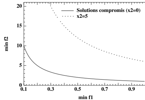
FIG. 1.1 – Les bornes du domaine de recherche du problème (\star)
