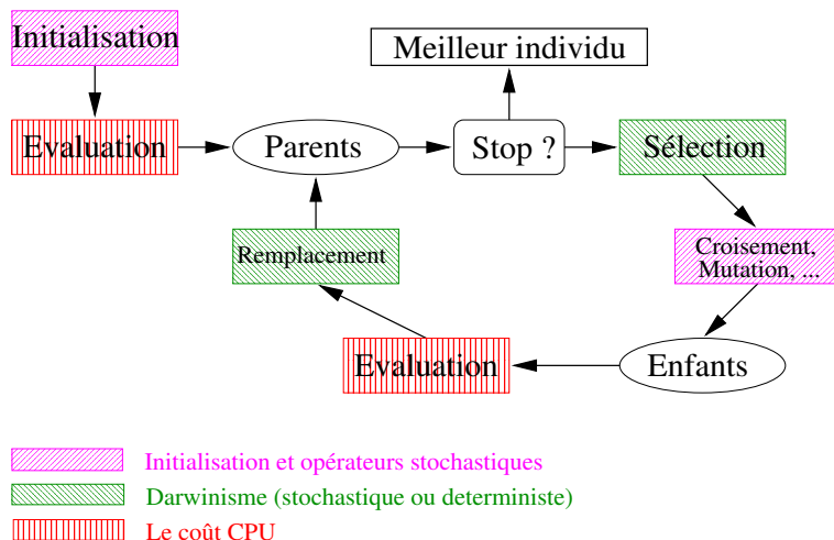
FIG. 2.1 – Cycle d'un AE
