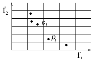
FIG. 3.8 – Préservation de la diversité dans PAES
