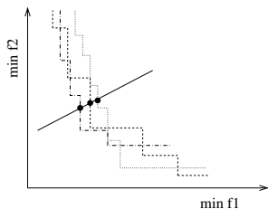
FIG. 4.12 – Frontières de dominance de trois essais différents de l'algorithme
