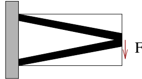
FIG. 4.5 – Problème de la plaque cantilever standard
