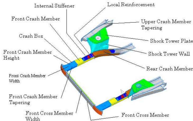
FIG. 7.2 – Paramétrisation du pare-choc
