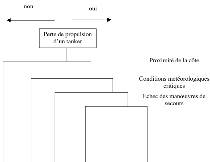
Figure 3 : Exemple d'arbre d'événements simplifié
