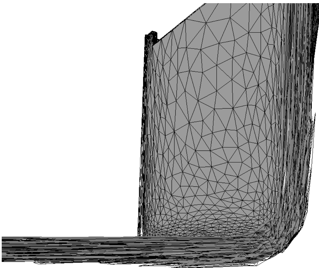
FIG. 4.20 – Maillage dans l'épaisseur de la demi traverse (vue écorchée)
