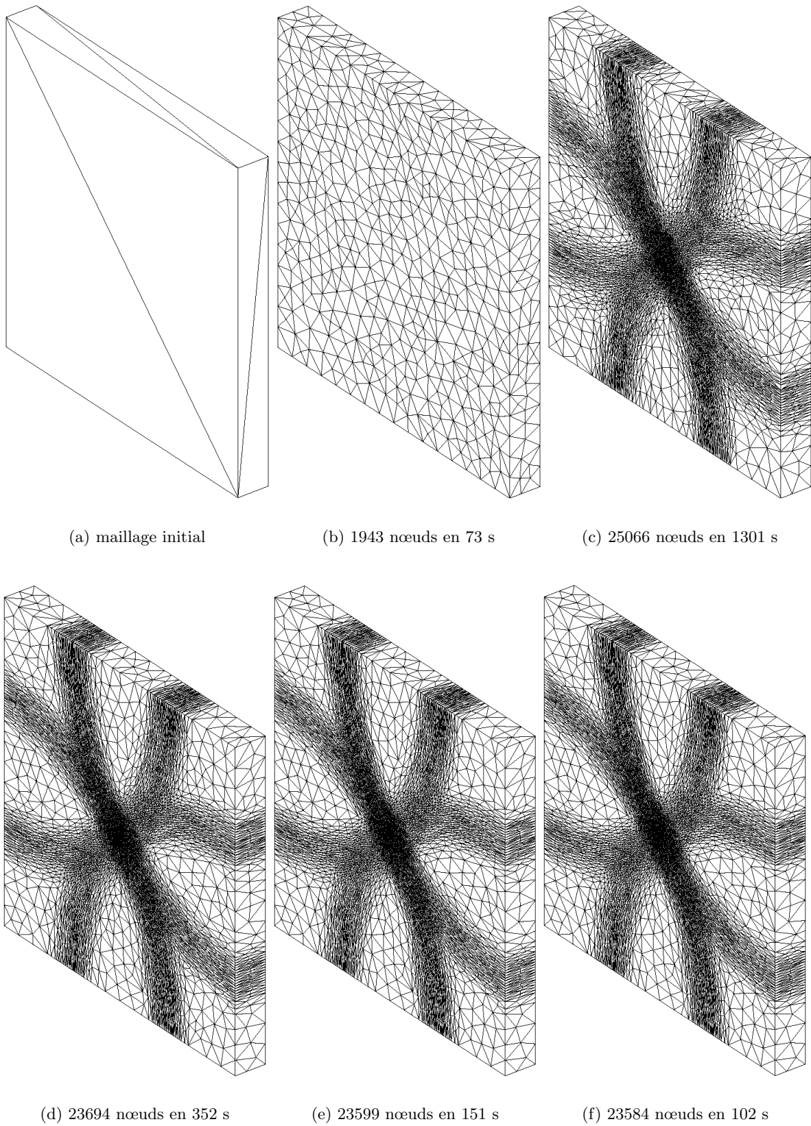
FIG. 3.9 – Processus itératif d'adaptation sur le cas test anisotrope 3D
