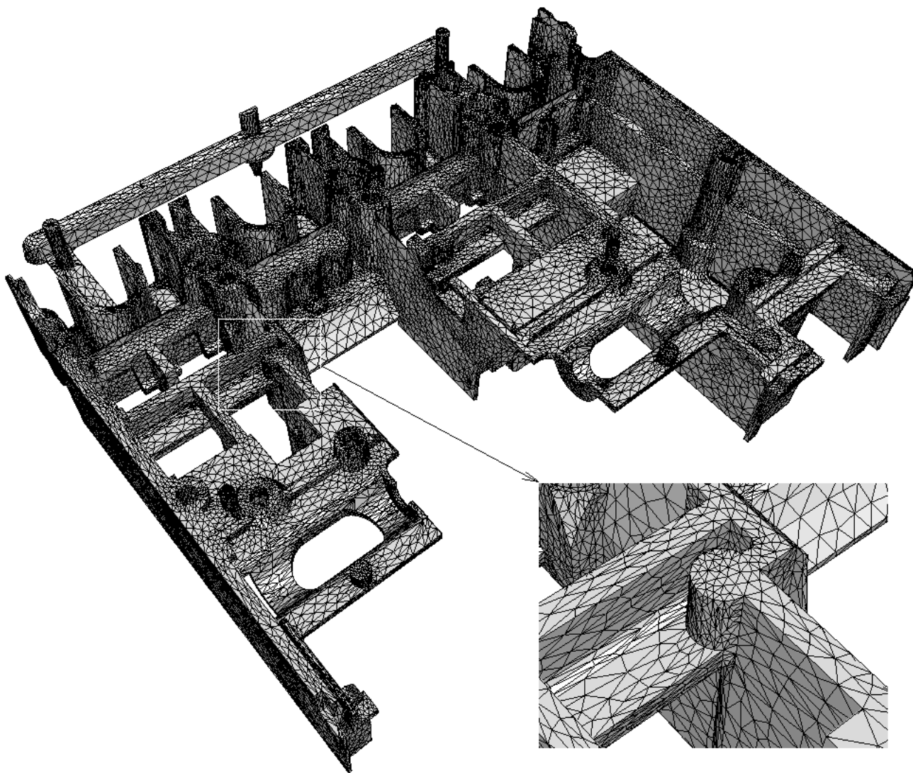
FIG. 4.24 – Maillage naturel (174 759 nœuds) de la pièce présentée sur la figure 3.13 et agrandissement de pièce était inimaginable avant la mise en place de la métrique naturelle. Ce blocage technologique est donc désormais levé.
