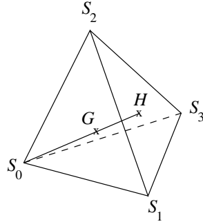
FIG. A.9 – tétraèdre équilatéral ( d = 3 )
