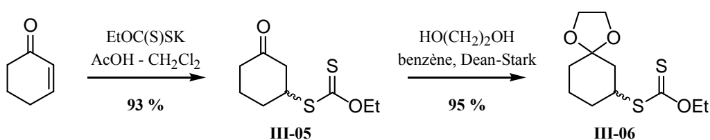
Figure III-105 essai de transformation d'un adduit en dioxolane
