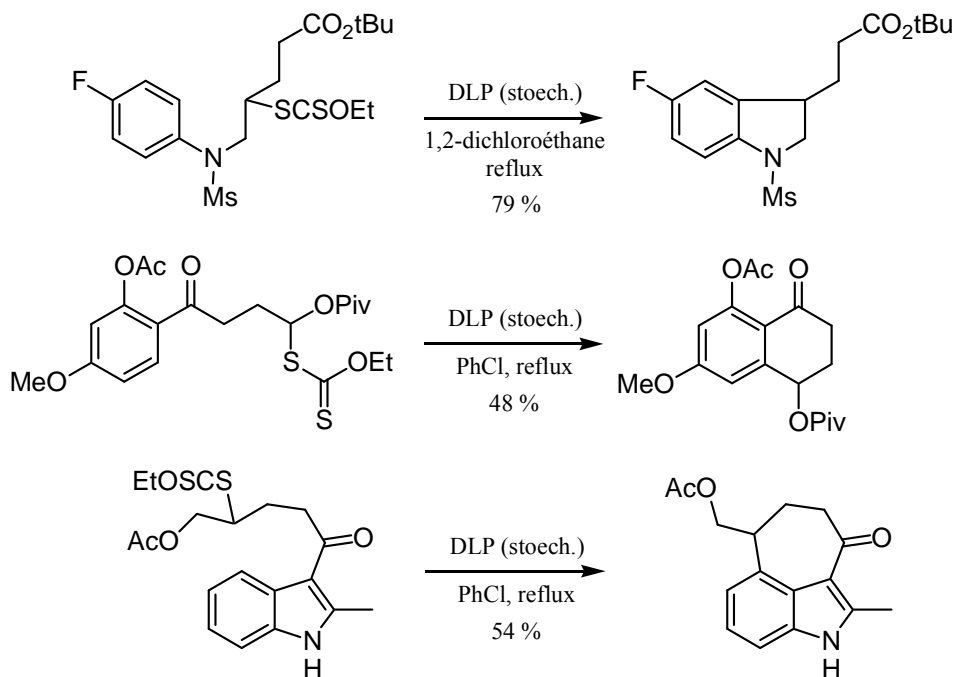
Figure I-19 cyclisations aromatiques
