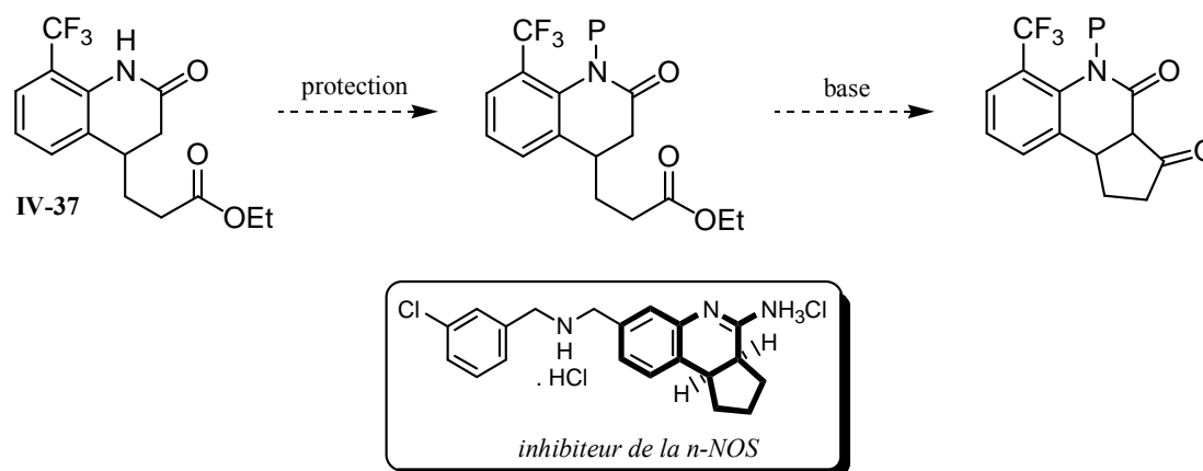
Schéma 9 formation d'une dihydroquinoléinone tricyclique ?
