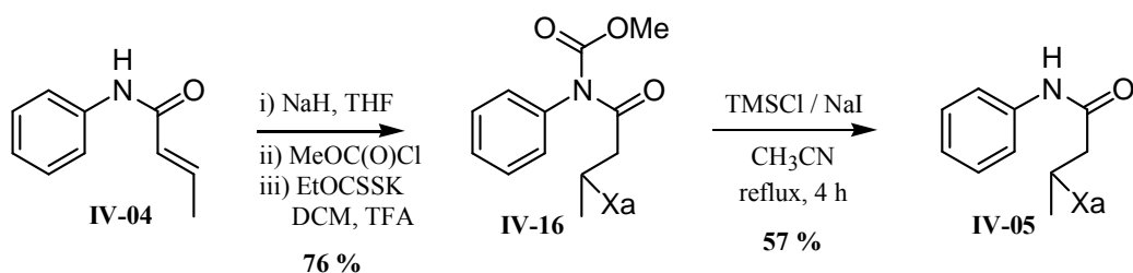
Figure IV-186 utilisation d'un carbamate de méthyle
