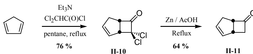
Figure II-25 mise en oeuvre du dichlorocétène
