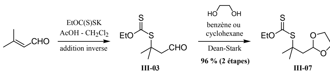
Figure III-106 essai de protection et préparation de III-07
