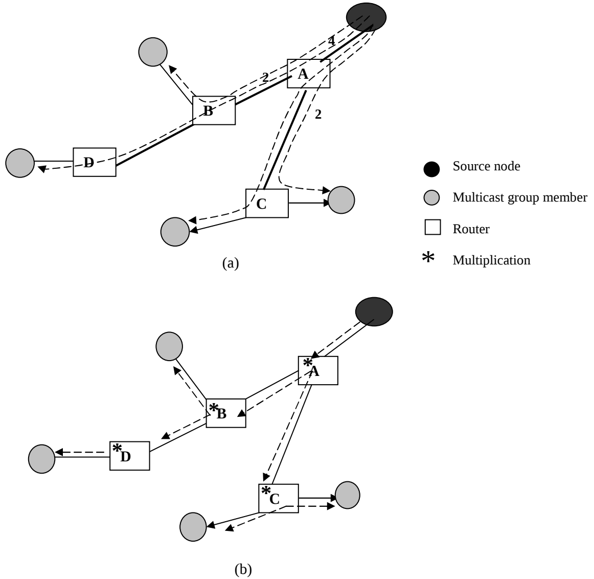
. Figure 3.2 (a) Unicast diffusion versus (b) Multicast diffusion
