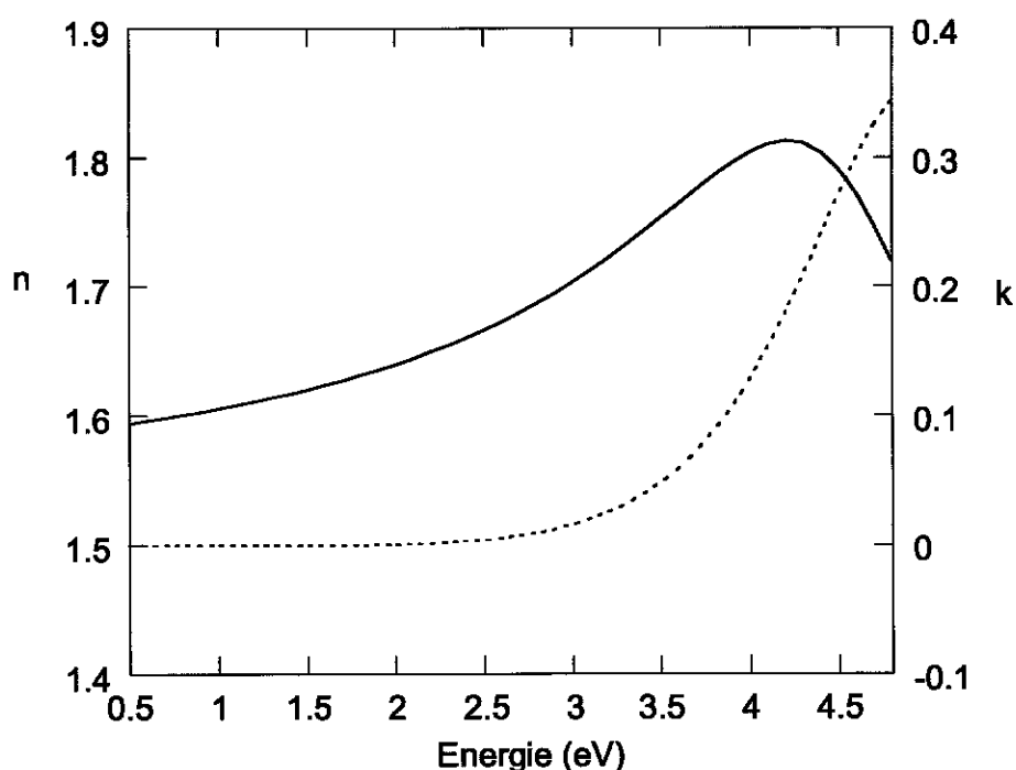
Figure IV-1 : Courbes représentant la partie réelle n (en trait plein) et la partie imaginaire k (en pointillé) de l'indice optique complexe modélisé en fonction de l'énergie suivant les formules (1) et (2). Les paramètres utilisés sont : n_\infty = 1,514 ; \omega_g = 1,737 eV ; f_j = 0,04 ; \omega_j = 4,714 eV ; \Gamma_j = 1,039 eV.
