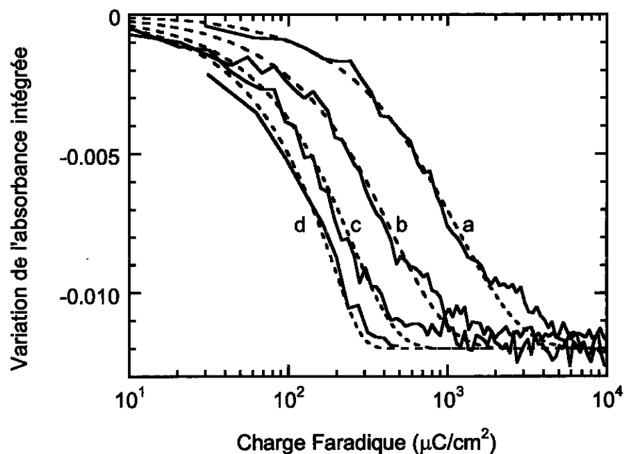
Figure II-12: Variation de la cinétique dans l'iodure de méthylmagnésium (3M), en fonction de la densité de courant appliquée : (a) 30 µA/cm 2 , (b) 100 µA/cm 2 , (c) 300 µA/cm 2 , (d) 1 mA/cm 2 . On constate que Q_0 diminue quand la densité de courant J augmente et que la cinétique passe alors d'une loi exponentielle (a) à une loi quasi linéaire (d). N.B. : l'échelle horizontale est logarithmique.
