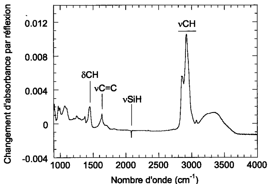
Figure IV-6 : Spectre d'absorption de la surface de Si (111) modifiée dans le bromure de vinylmagnésium ( 0,5\text{mA/cm}^2 , pendant 5 mn), dans le tétrahydrofuranne.
