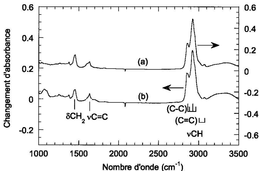
Figure IV-7 : Spectres d'absorption de la surface de Si (111) modifiée dans le bromure de vinylmagnésium ( 0,5\text{mA/cm}^2 , pendant 5 mn) (a) : dans le tétrahydrofurane (b) : dans le dichlorobenzène
