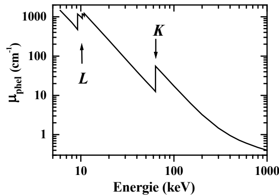
Figure IV 8 : Coefficient d'atténuation de l'effet photoélectrique \mu_{phel} ( \text{cm}^{-1} ) du \text{Lu}_2\text{Si}_2\text{O}_7 (LPS).
