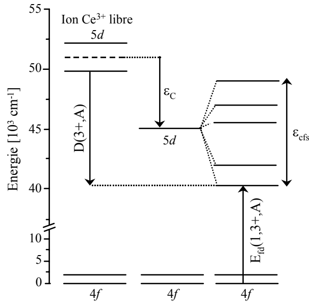
Figure V 7 : Schéma de l'influence du champ cristallin sur l'énergie de la configuration 5d du \text{Ce}^{3+} . L'éclatement du champ cristallin \epsilon_{\text{CFS}} , le déplacement du barycentre \epsilon_{\text{C}} , le “redshift” D(3+,A) et la première transition 4f \rightarrow 5d du \text{Ce}^{3+} , E_{\text{fd}}(1,3+,A) , sont indiqués. D'après [18].
