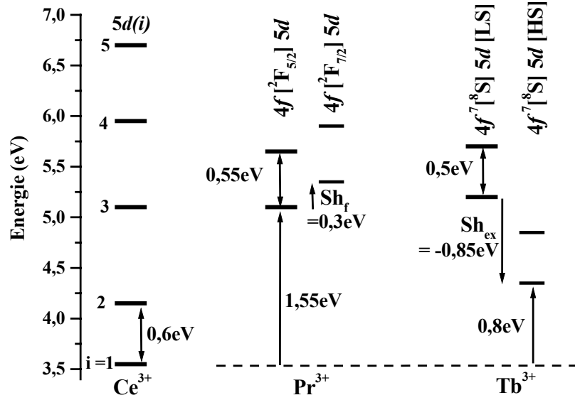
Figure VI 7 : Niveaux d'énergie 5d expérimentaux des ions \text{Ce}^{3+} , \text{Pr}^{3+} et \text{Tb}^{3+} dans la matrice \text{Lu}_2\text{Si}_2\text{O}_7 .
