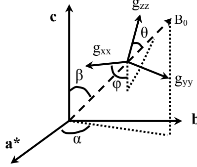
Figure III 1 : Orientation générale des axes principaux du tenseur g par rapport à un trièdre de référence ( a^*bc ). Le champ magnétique \vec{B}_0 est représenté en pointillés.
