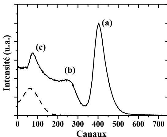
Figure II 14 : Spectre de "pulse height" d'un cristal de \text{Lu}_2\text{Si}_2\text{O}_7:\text{Ce} (LPS) excité par une source de ^{137}\text{Cs} (trait plein). Spectre du "single electron" enregistré sans source, avec un gain total 500 fois supérieur au spectre de "pulse height" (pointillés).
