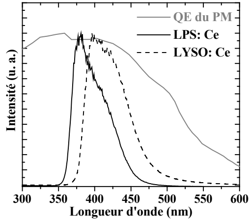
Figure IV 1 : Comparaison des spectres d'émission sous X de \text{Lu}_{1,8}\text{Y}_{0,2}\text{SiO}_5:0,11\%\text{Ce} (LYSO) et \text{Lu}_2\text{Si}_2\text{O}_7:0,5\%\text{Ce} (LPS) avec l'efficacité quantique QE d'un photomultiplicateur Hamamatsu R1791.
