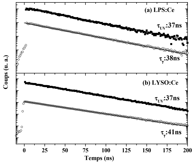
Figure IV 9 : Déclins de fluorescence du \text{Ce}^{3+} dans (a) \text{LPS:0,25\%Ce} et (b) \text{Lu}_{1,8}\text{Y}_{0,2}\text{SiO}_5:0,11\%\text{Ce} sous excitation gamma (source ^{137}\text{Cs} , 662 keV, ○) et UV ( \lambda_{\text{exc}}=355\text{ nm} , ■). Les déclins sont simulés par une loi exponentielle.
