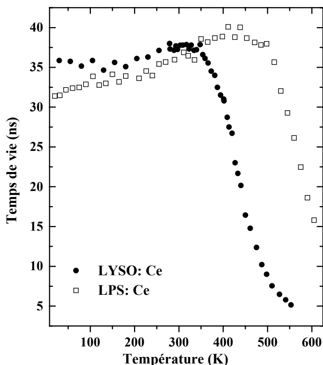
Figure V 8 : Valeurs des temps de vie sous excitation laser-UV ( \lambda_{exc}=355 nm, 3,5 eV) du Ce 3+ dans LPS ( \lambda_{em}=385 nm, □) et LYSO ( \lambda_{em}=393 nm, ●) en fonction de la température.
