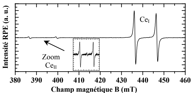
Figure III 17 : Spectres RPE à 12K de l'ion \text{Ce}^{3+} dans LSO tel que le champ magnétique \vec{B}_0 soit parallèle à l'axe a [100] ( \pm 5^\circ ). Puissance : 20 mW ; amplitude de modulation : 0,3 mT ; fréquence de modulation : 100 kHz ; constante de temps : 20 ms et fréquence : 9,5 GHz.
