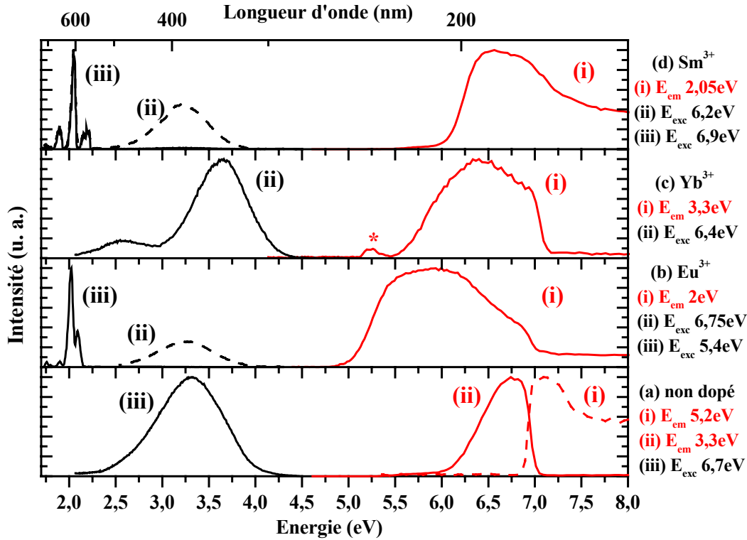
Figure VI 3 : Spectres d'excitation (—) et spectres d'émission (—) à 10 K d'un cristal de \text{Lu}_2\text{Si}_2\text{O}_7 (LPS) : (a) non dopé, (b) dopé \text{Eu}^{3+} , (c) \text{Yb}^{3+} et (d) \text{Sm}^{3+} . Concentrations initiales en dopant : 0,5% pour \text{Eu}^{3+} et \text{Sm}^{3+} , 5% pour l' \text{Yb}^{3+} . Le pic indiqué par une étoile est attribué à une impureté de \text{Tb}^{3+} .
