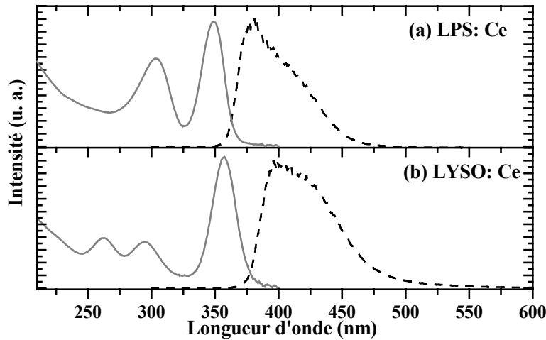
Figure IV 2 : Spectres d'absorption (—) et d'émission sous excitation X (---) à température ambiante de cristaux de \text{Lu}_2\text{Si}_2\text{O}_7:0,5\%\text{Ce} (a) et \text{Lu}_{1,8}\text{Y}_{0,2}\text{SiO}_5:0,11\%\text{Ce}^* (b). Lames de 1 mm.
