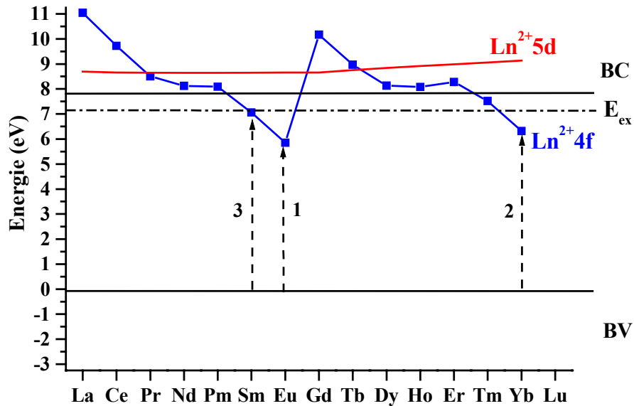
Figure VI 1 : Position des niveaux d'énergie des ions lanthanides divalents dans \text{Lu}_2\text{Si}_2\text{O}_7 . Les flèches en pointillés indiquent les transferts de charge étudiés expérimentalement dans ce travail. Pour l'ion \text{Tm}^{3+} , aucune bande correspondant au transfert de charge n'a été observée expérimentalement.
