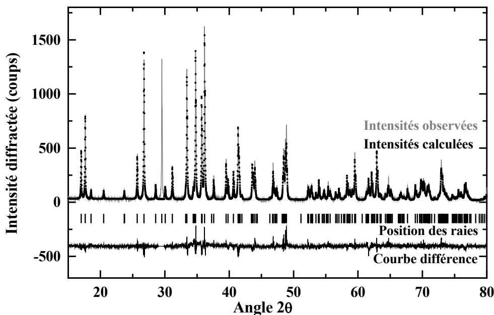
Figure III 4 : Affinement Rietveld du diffractogramme sur cristal broyé de Lu_{1,4}Y_{0,6}SiO_5 (LYSO avec 30% d'yttrium). \lambda_{K\alpha C0} ; \chi^2=2,4 ; facteur de Bragg : R_B=9,2 .
