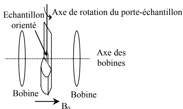
Figure II 23 : Dispositif expérimental du spectromètre RPE dans le cas de variations angulaires du champ magnétique.
