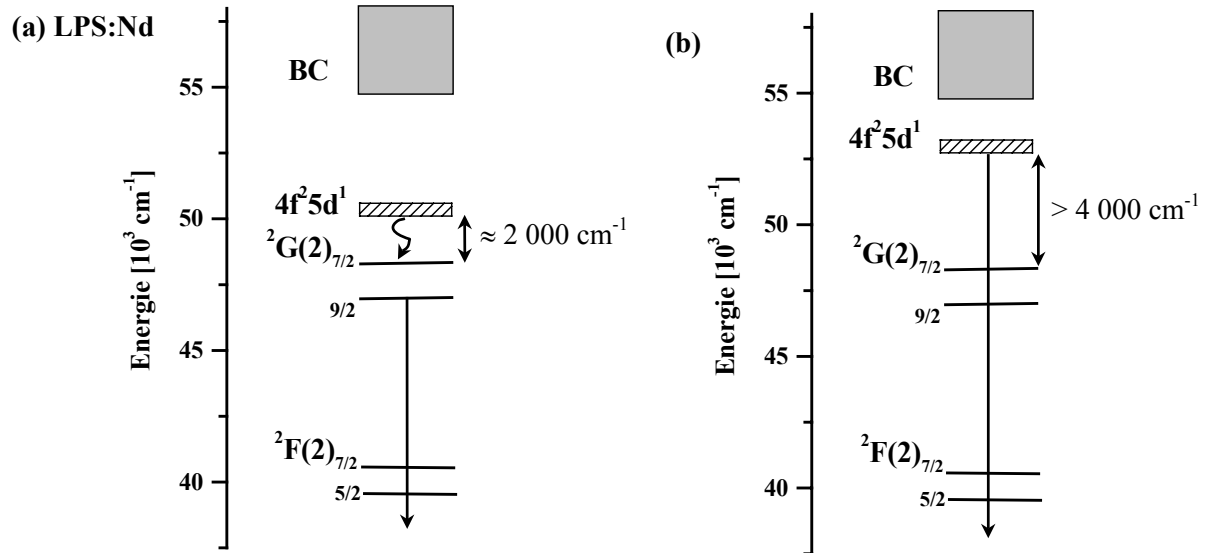
Figure VI 8 : Schémas des niveaux d'énergie de l'ion \text{Nd}^{3+} (a) dans la matrice \text{Lu}_2\text{Si}_2\text{O}_7 où l'émission non-radiative du niveau 4f^25d^1 est suivie de l'émission radiative des transitions f-f , (b) dans une matrice telle que l'émission d-f soit observée.
