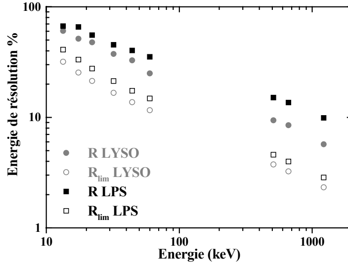
Figure IV 7 : Résolutions énergétiques observée R et intrinsèque R_{lim} de cristaux de \text{Lu}_2\text{Si}_2\text{O}_7:0,5\%\text{Ce} et \text{Lu}_{1,8}\text{Y}_{0,2}\text{SiO}_5:0,11\%\text{Ce} ( 10 \times 10 \times 10 \text{ mm}^3 ) en fonction de l'énergie d'excitation. Temps d'intégration : 3 \mu\text{s} .
