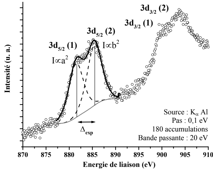
Figure V 16 : Spectre XPS des niveaux 3d du \text{Ce}^{3+} ( 3d_{5/2} et 3d_{3/2} ) dans le LPS:8%Ce (○). Le doublet du niveau 3d_{5/2} est simulé par deux fonctions symétriques de type Gaussienne/ Lorentzienne (50/50) avec les valeurs du Tableau V 4 (pointillés). La somme de ces fonctions et le bruit de fond sont également représentés (—).
