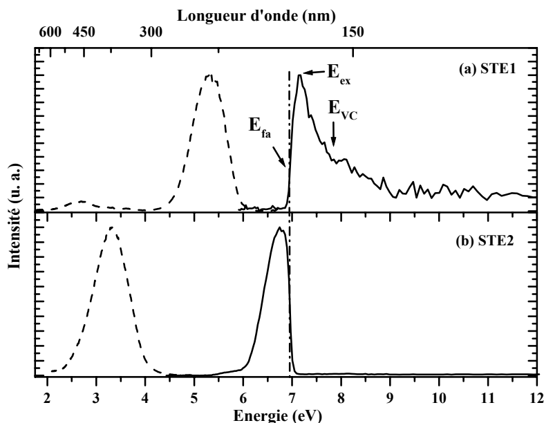
Figure V 1 : Spectres d'excitation (—) du \text{Lu}_2\text{Si}_2\text{O}_7 (LPS) non dopé à 10 K, pour une émission à 5,2 (a) et 3,3 eV (b). Spectres d'émission (---) pour une excitation sous X à 100 K (a) et à 6,7 eV à 10 K (b).
