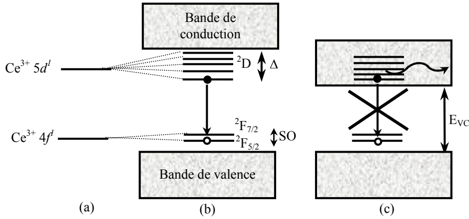
Figure I 6 : Schémas des niveaux d'énergie de l'ion \text{Ce}^{3+} (a) libre, (b) au sein d'une matrice à large bande interdite, (c) au sein d'une matrice à faible bande interdite.
