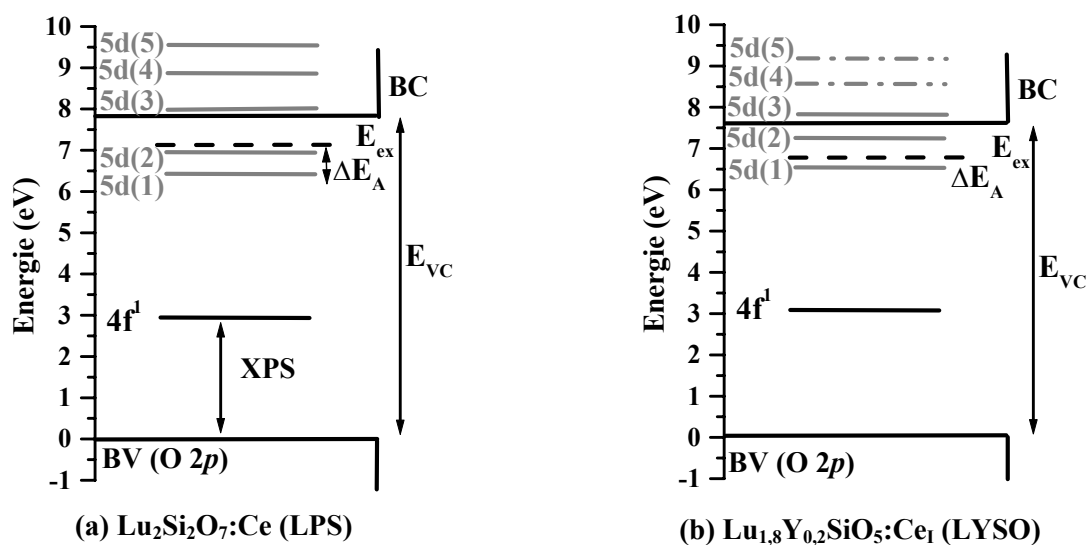
Figure V 17 : Représentation schématisée de la position relative des niveaux 4f^1 et 5d^1 du \text{Ce}^{3+} par rapport aux niveaux de la matrice et au niveau excitonique pour LPS et LYSO. Le niveau 4f^1 est composé de 2 niveaux séparés de 0,25 eV, non représentés ici.
