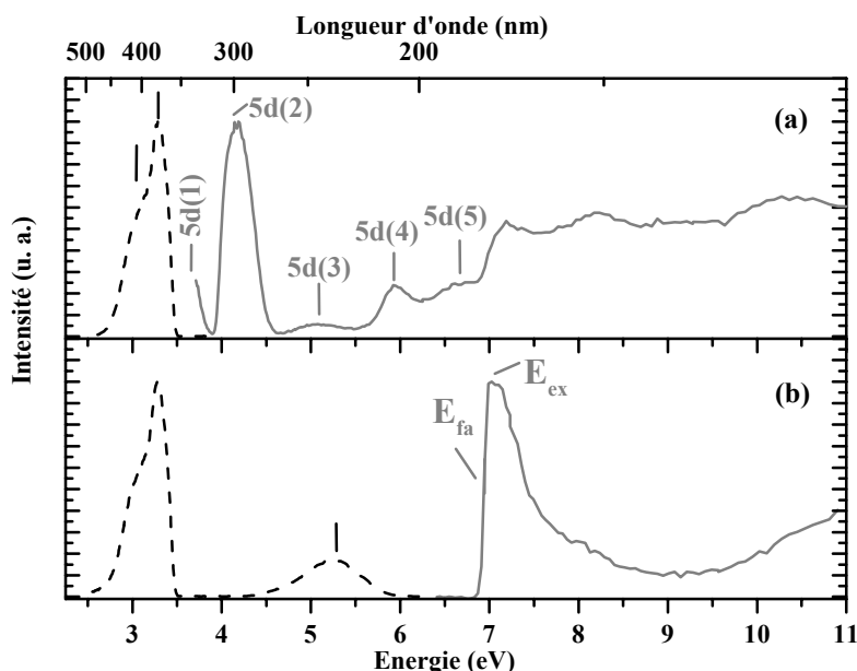
Figure V 5 : Spectres d'excitation (—) du \text{Lu}_2\text{Si}_2\text{O}_7:\text{Ce}^{3+} pour l'émission du cérium à 3,3 eV (a) et l'émission de la matrice à 5,3 eV (b) et spectres d'émission (- - -) pour une excitation du cérium à 4,1 eV (a) et une excitation du niveau excitonique à 7,15 eV (b) à 10 K.
