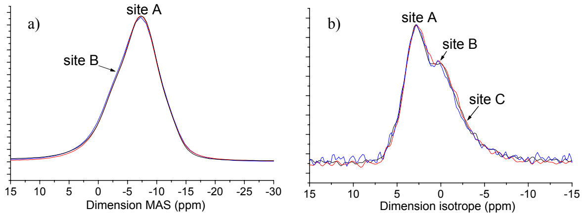
Figure VI.9 : Projections dans la dimension MAS (a) et isotrope (b) du spectre 3Q-MAS des hollandites \text{Ba}_{1,16}\text{Al}_{2,32}\text{Ti}_{5,68}\text{O}_{16} , avant (noir) et après irradiation (bleu : irradiée 1 MeV F=8,7 \cdot 10^{18} \text{ cm}^{-2} ; rouge : irradiée 1,5 MeV F=5,8 \cdot 10^{18} \text{ cm}^{-2} ), ( B_0=11,75 \text{ T} , \nu_R = 31500 \text{ Hz} ). L'intensité des spectres a été ramenée à la même échelle.
