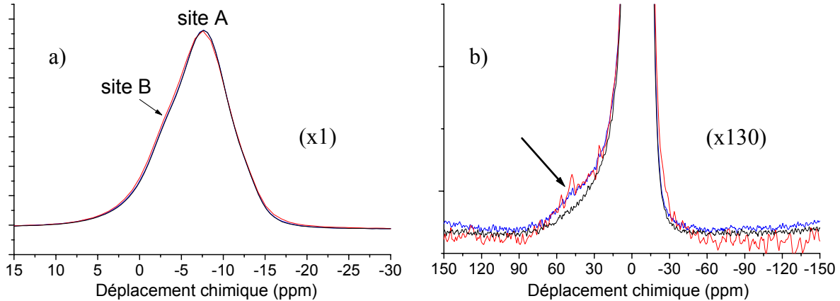
Figure VI.8: Spectres RMN MAS ^{27}\text{Al} de la hollandite \text{Ba}_{1,16}\text{Al}_{2,32}\text{Ti}_{5,68}\text{O}_{16} avant (noir) et après irradiation (bleu: irradiée 1 MeV F=8,7 \cdot 10^{18} \text{ cm}^{-2} ; rouge: irradiée 1,5 MeV F=5,8 \cdot 10^{18} \text{ cm}^{-2} ); ( B_0=11,74 \text{ T} , \nu_R = 31500 \text{ Hz} ).
