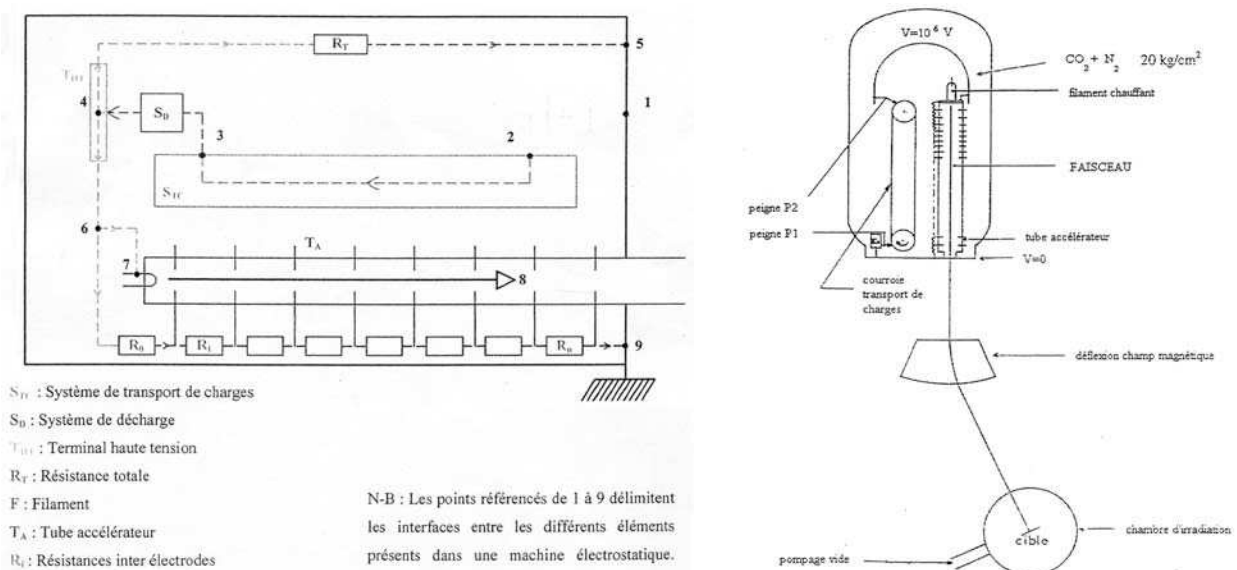
Figure A.V.1 Schémas de fonctionnement d'un accélérateur de Van de Graaff.
