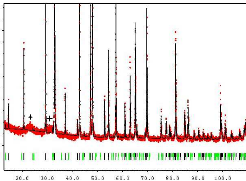
Figure IV.12 : Diagramme de diffraction X de poudre de la hollandite Ba_{1,16}Al_{2,32}Ti_{5,68}O_{16} (en rouge) avec les raies larges supplémentaires (◆) et diagramme simulé en considérant la structure I4/m(000,38)00 (en noir). Les traits verts indiquent les positions des raies satellites calculées, ceux de couleur noire correspondent aux raies principales. ( \lambda_{Co}=1,789 \text{ \AA} ).
