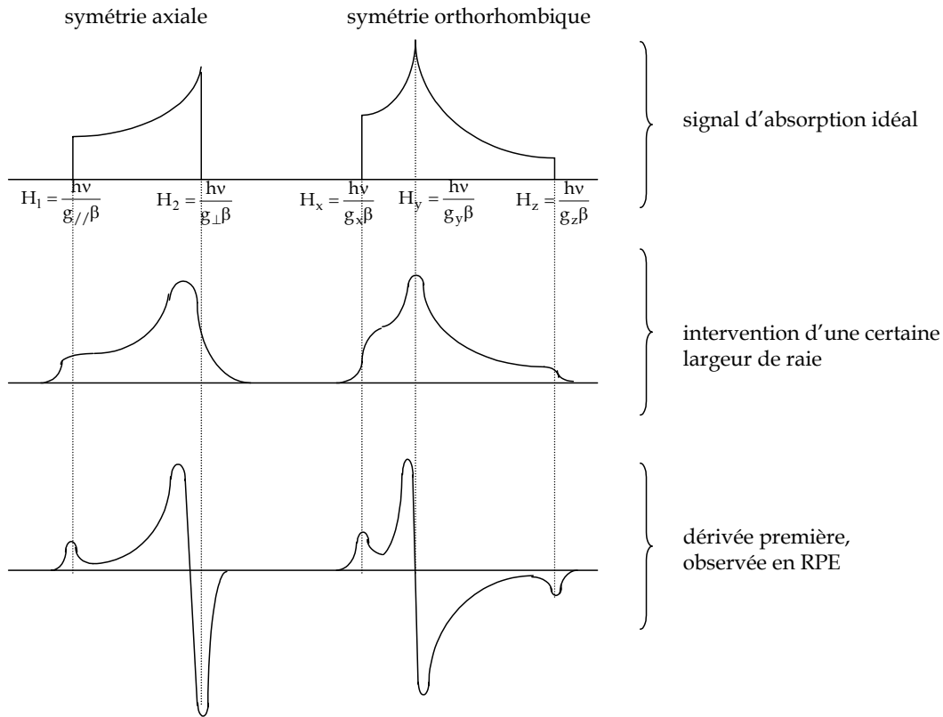
Figure A.VII.9 : spectres RPE de poudre d'un centre paramagnétique selon la symétrie de son site.
