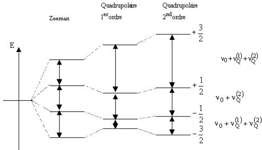
Figure A.VII.6 : Représentation schématique des niveaux d'énergie d'un spin I=3/2 soumis à une interaction quadrupolaire du premier ordre et du second ordre avec v_Q = \frac{3C_Q(1+\eta^2/3)^{1/2}}{2I(2I-1)} , v_0 la fréquence de Larmor.
