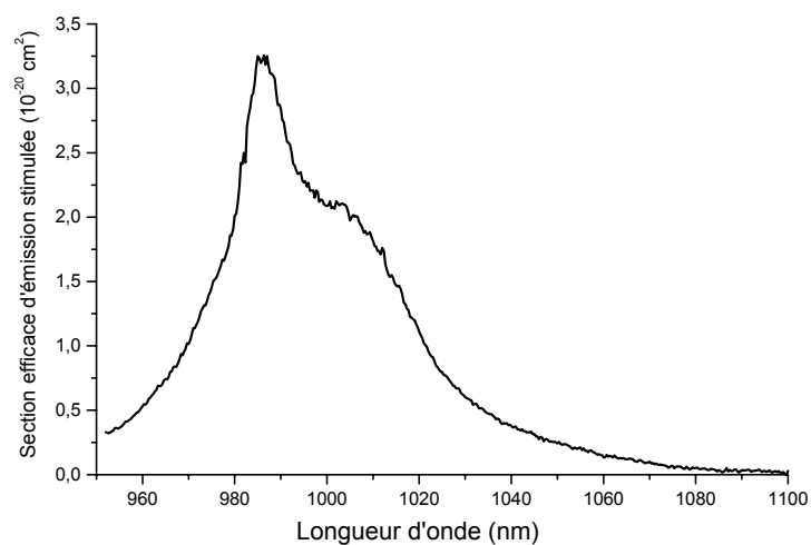
Figure 4. 39. Section efficace d'émission stimulée de \text{GdVO}_4:\text{Yb}^{3+} .
