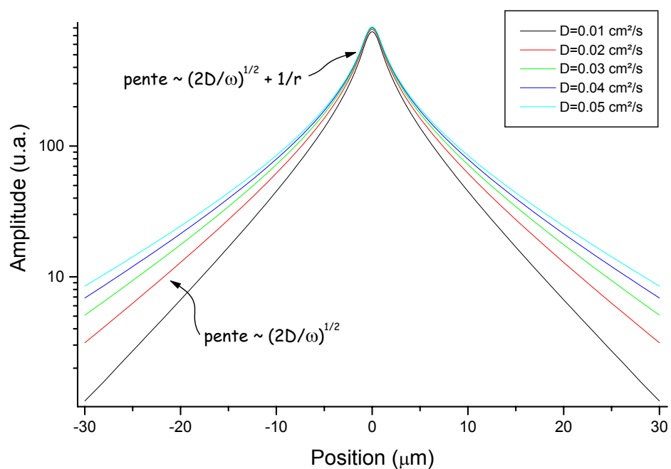
Figure 4. 5. Evolution théorique de l'amplitude du faisceau sonde réfléchi en fonction de la distance entre les faisceaux de pompe et de sonde. On a fait varier la valeur de la diffusivité thermique D de l'échantillon. La pente dépend de la longueur de diffusion et varie comme l'inverse de la distance r séparant les deux faisceaux. Cette dépendance devient négligeable loin de l'origine du graphique.
