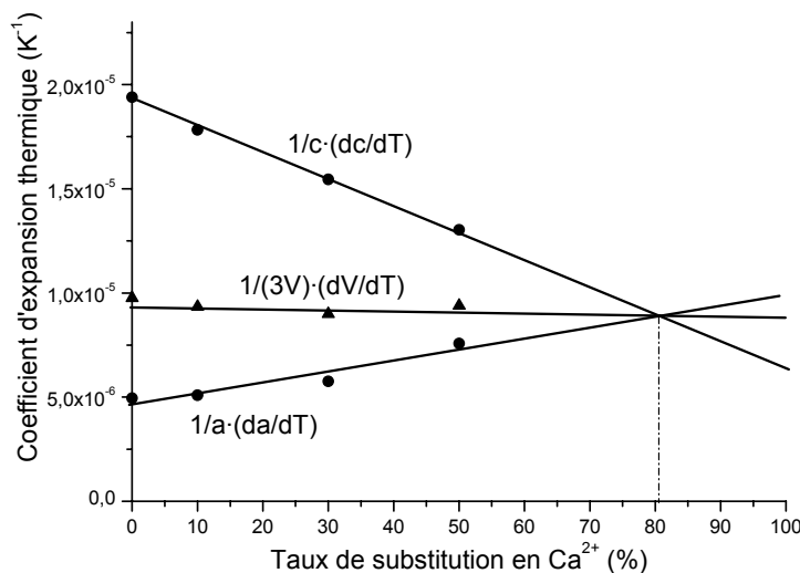
Figure 3.10 Coefficients d'expansion thermique de (\text{Sr}_{1-x}\text{Ca}_x)_3\text{Y}(\text{BO}_3)_3 : \text{Yb}^{3+} pour différents taux de substitution en calcium 0 < x < 0,5 .
