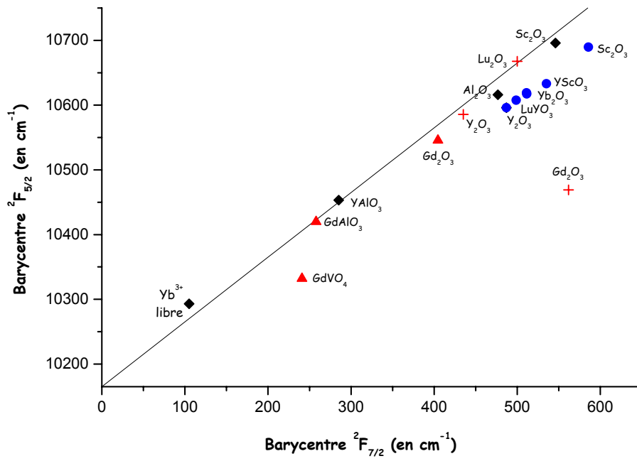
Figure 4. 46. Diagramme des barycentres de l'ion \text{Yb}^{3+} dans différentes matrices sesquioxydes et pérovskites. (+ : [48], • [61], ◆ [cf. Annexe A], ▲ [ce travail])
