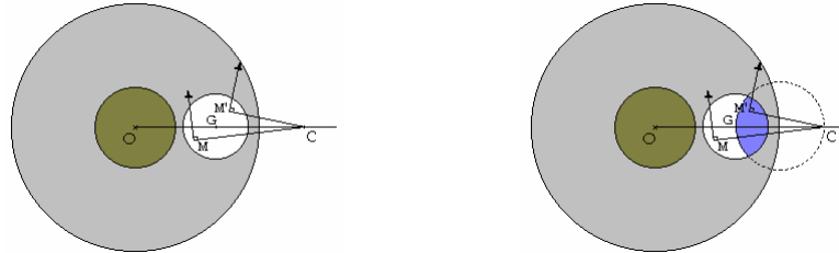
Figure 2.15 Effet du couple des forces de frottement.
