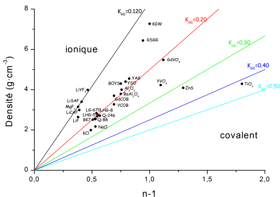
Figure 4. 18. Relation entre la densité et l'indice de réfraction moyen pour différents solides cristallins.
