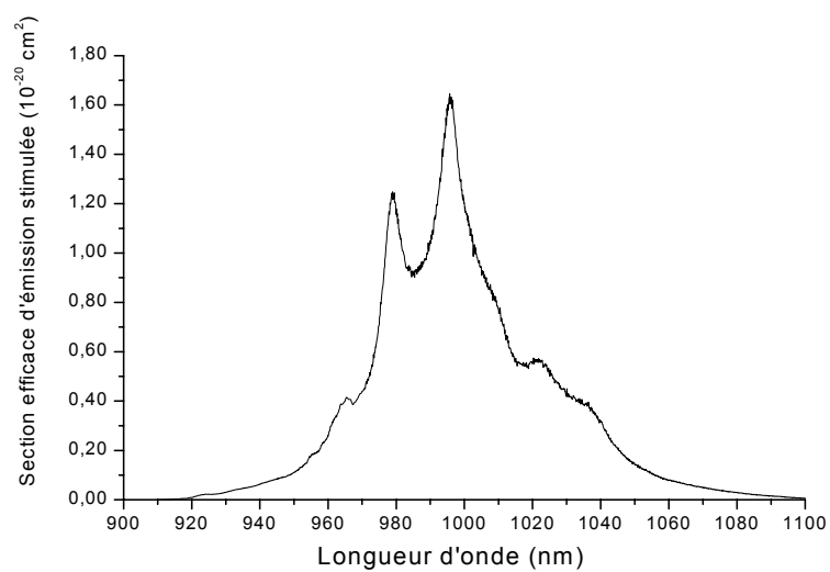
Figure 4. 41. Section efficace d'émission stimulée de \text{GdAlO}_3:\text{Yb}^{3+} .
