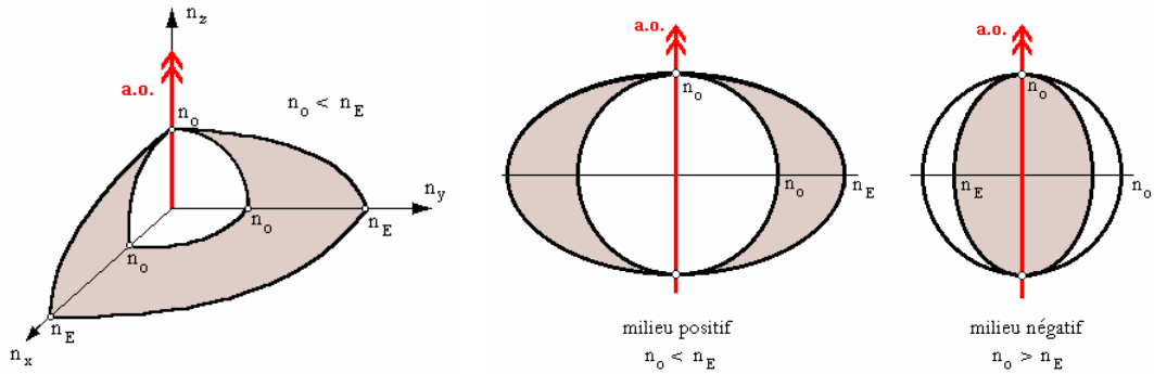
Figure 2.4 Surface des indices d'un cristal uniaxe
