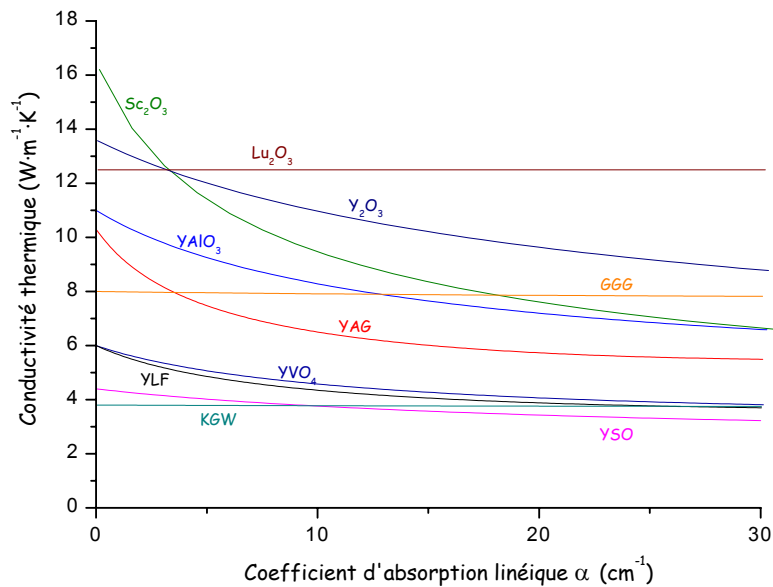
Figure 4. 12. Evolution de la conductivité thermique avec le coefficient d'absorption linéique \alpha au voisinage de 980 nm dans des matériaux dopés à l'Yb 3+ (On suppose la raie d'absorption infiniment fine pour ne pas avoir à tenir compte du recouvrement spectral avec la diode laser de pompage).
