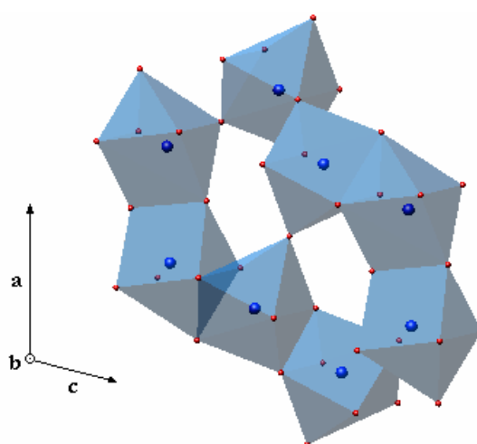
Figure 4. 24. Empilements des polyèdres de coordination dans Gd 2 O 3 monoclinique.
