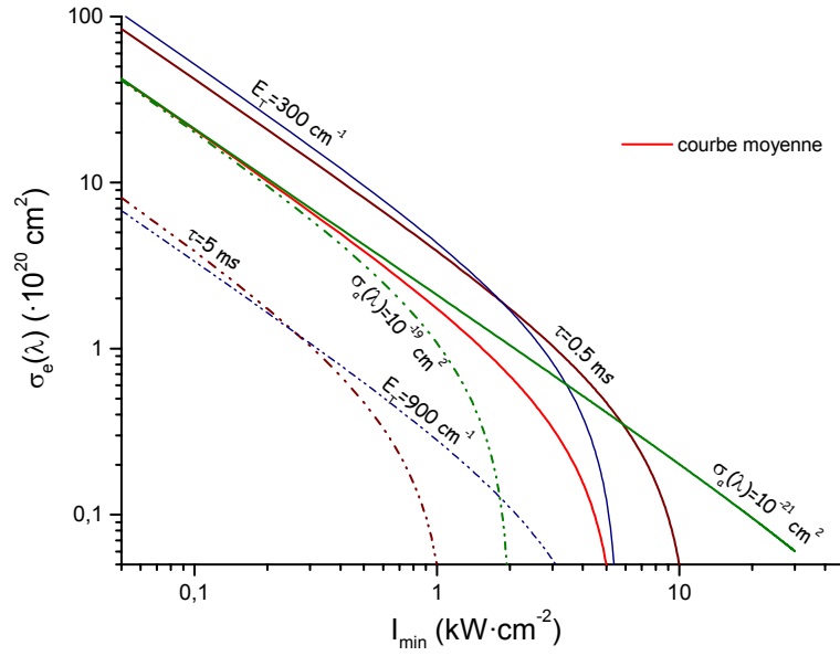
Figure 1. 20. \sigma_e vs I_{\min} : Influence des paramètres E_T , \tau et \sigma_a(\lambda_p) , la figure est obtenue selon la relation eq. 1.42 en ne faisant varier qu'un paramètre, les autres étant fixés à leurs valeurs moyennes.
