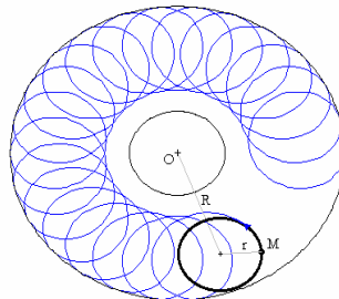
Figure 2.24 Mouvement hypocycloïdal d'un point du porte-échantillon. La conditions de périodicité du mouvement hypocycloïdal s'écrit : \alpha \tau / (R+r) \in \mathbb{Q} où \alpha est le coefficient de glissement du porte-échantillon sur le plateau.
