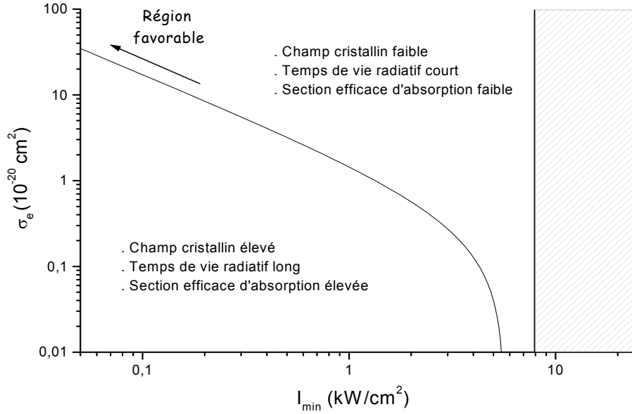
Figure 1. 19. \sigma_e vs I_{\min} : version schématique.
