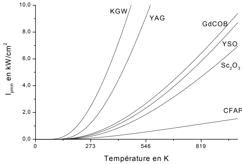
Figure 1. 27. I_s vs T pour quelques matériaux laser usuels.
