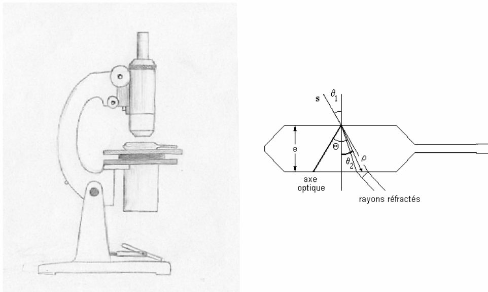
Figure 2.5 Conoscope de Descloizeaux, et représentation d'un cristal biréfringent dans les conditions d'observation.
