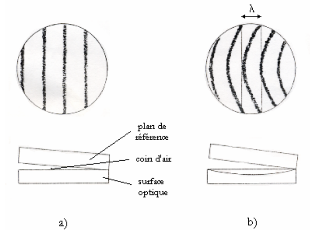
Figure 2. 28. Contrôle de la planéité d'une surface optique. On observe les franges de coin d'air formées entre un plan de référence et la surface à contrôler. Si la surface est plane, les franges sont rectilignes (figure a), elles sont courbes dans le cas contraire (figure b). Dans ce cas, l'espacement entre l'arc d'une frange et sa corde correspond à un déphasage de l'onde égal à la longueur d'onde \lambda .
