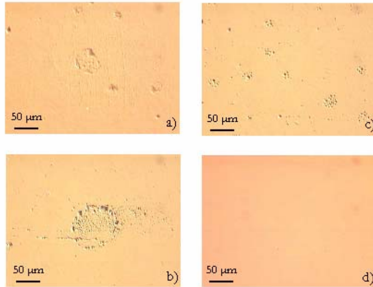
Figure 2.26 Mise en évidence de l'hygroscopicité du borate YCOB (photos a, b et c).
