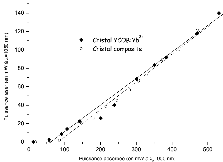
Figure 2.38 Test laser comparatif entre un cristal YCOB:Yb 3+ 15 % et un cristal composite YCOB:Yb 3+ 15 % || YCOB. La polarisation de la pompe selon Z et la propagation selon X.
