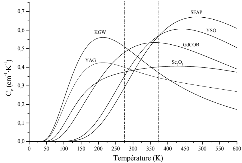
Figure 1. 26. Capacité thermique électronique des ions \text{Yb}^{3+} en fonction de la température pour une inversion de population \beta_{\min}(T) .
