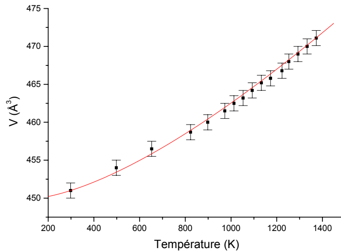
Figure 4. 15. Evolution du volume de la maille cristalline du GdCOB avec la température. Le meilleur ajustement aux données expérimentales est obtenu pour n=1.46 et \varepsilon=1.019 . Données expérimentales d'après [32].
