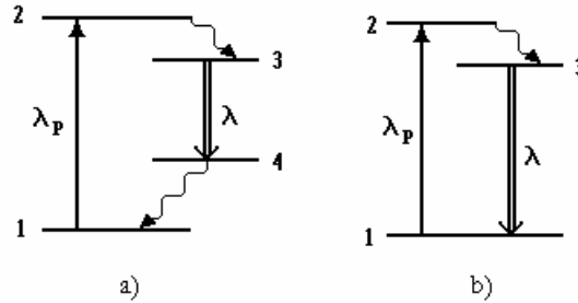
Figure 1. 13. Fonctionnement d'un laser à 4 niveaux (a) et à 3 niveaux (b).
