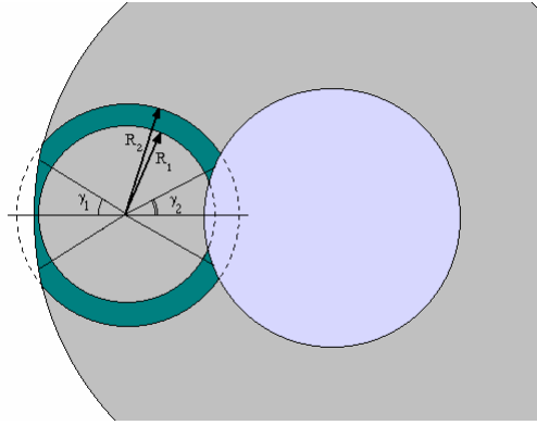
Figure 2.17. Dépassement de la semelle du porte-échantillon (en vert) sur le plateau tournant (en gris). Les notations indiquées sont reprises dans le texte.
