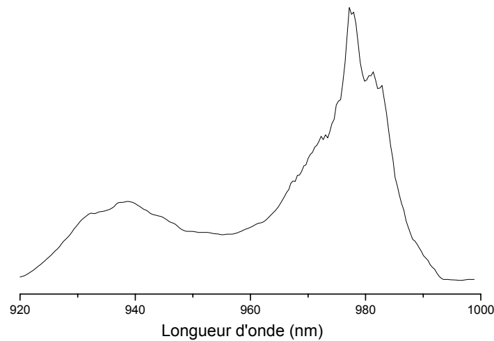
Figure 4. 37. Spectre d'excitation de la fluorescence à température ambiante de \text{Gd}_2\text{O}_3:\text{Yb}^{3+} ( \lambda_{\text{em}}=1008\ \text{nm} ).
