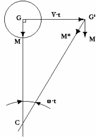
Figure 2.10 Définition du centre instantané de rotation du porte-échantillon dans le repère mobile lié au plateau tournant.
