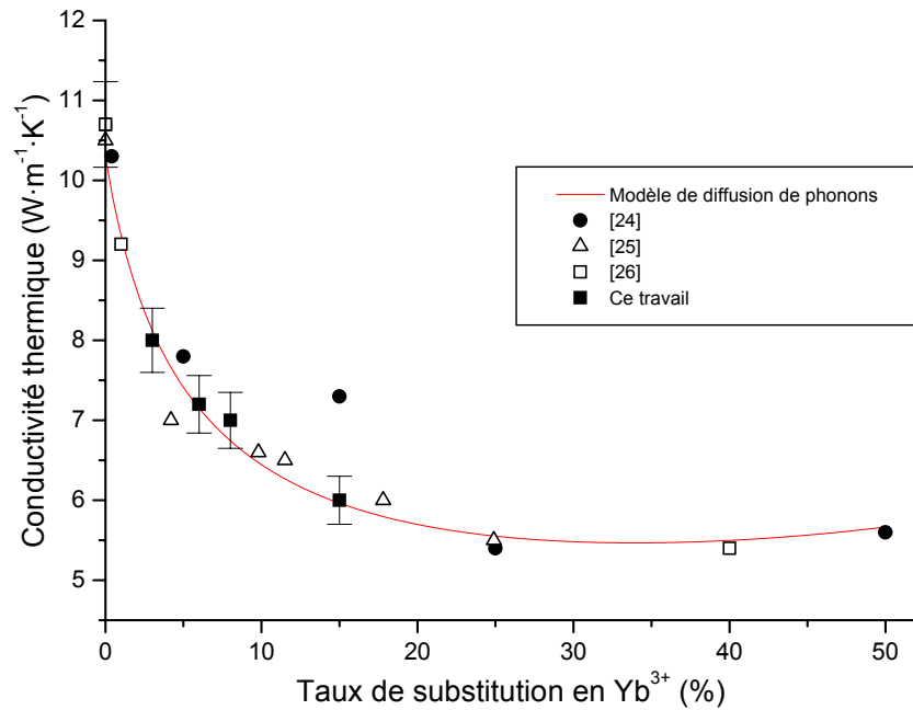
Figure 4. 3. Evolution de la conductivité thermique avec le taux de substitution en Yb³⁺ dans le YAG : Yb³⁺.
