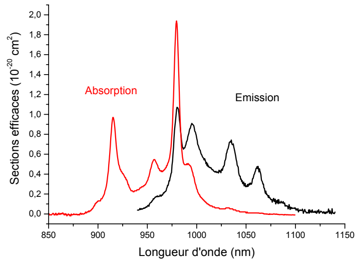
Figure 4. 33. Sections efficaces d'absorption et d'émission stimulée dans \text{Sc}_2\text{SiO}_5:\text{Yb}^{3+} 1 at. % à température ambiante.
