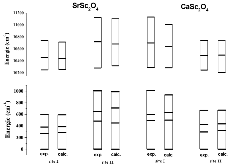
Figure 4. 32. Niveaux d'énergie expérimentaux et calculés dans les composés \text{CaSc}_2\text{O}_4:\text{Yb}^{3+} et \text{SrSc}_2\text{O}_4:\text{Yb}^{3+} . Deux sites cristallographiques sont possibles pour la substitution de l'ytterbium et sont effectivement observés expérimentalement.
