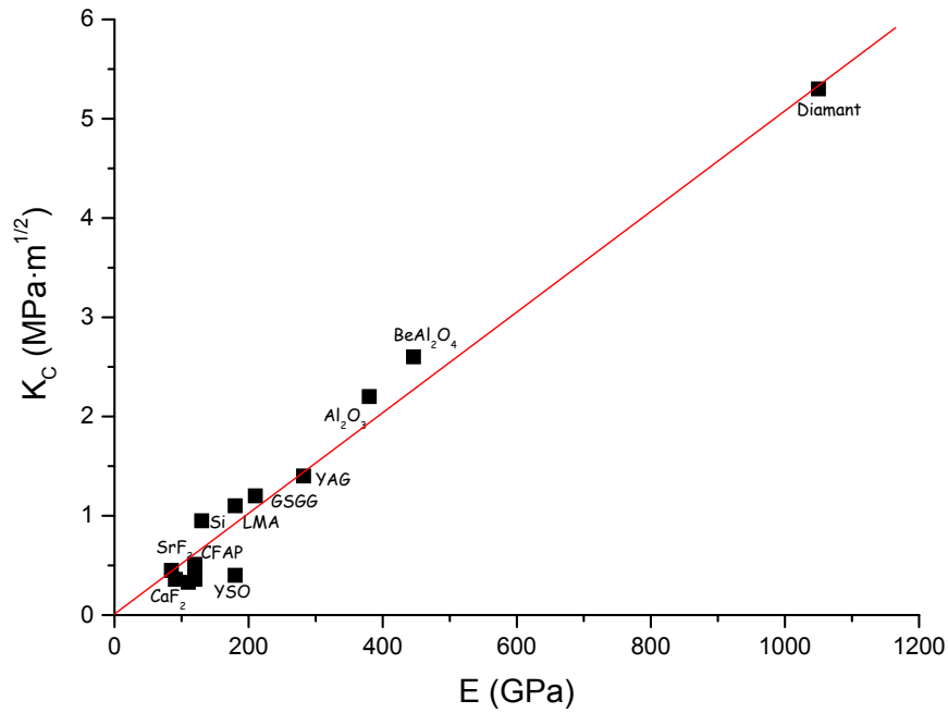
Figure 4. 17. Evolution du coefficient de résistance à la fracture K_C avec le module d'Young E .
