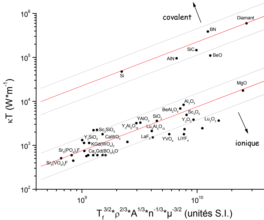
Figure 4. 1. Représentation en coordonnées logarithmiques de la relation 4.41 pour quelques matrices cristallines non dopées à température ambiante. Les droites de pentes unité représentées en rouge figurent la tendance générale suivie par les composés ioniques et covalents. Les droites grises qui les encadrent
