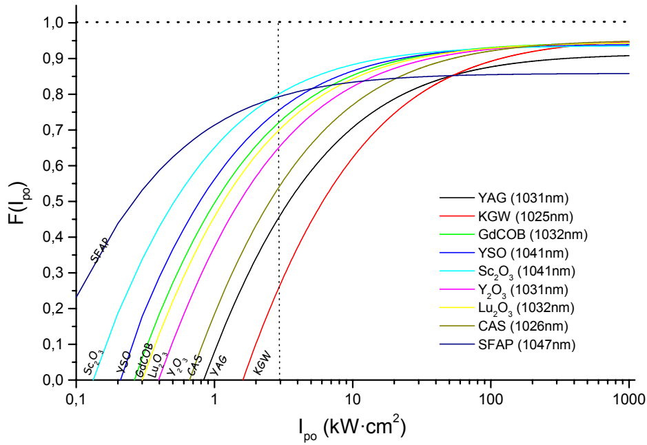
Figure 1.23. Comparaison des rendements différentiels réduits de quelques matériaux laser dopés à l'ytterbium suivant la valeur de l'intensité de pompage I_{po} . La droite verticale en pointillés indique la valeur de I_{po} pour une puissance de 1W concentrée sur un disque de 200 \mu\text{m} de diamètre. Pour les tests laser à moyenne puissance des chapitres 2 et 3 (pages 85 et 107), la valeur de I_{po} est de l'ordre de 30 \text{kW} \cdot \text{cm}^{-2} .
