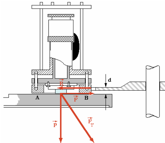
Figure 2.23 Bilan des forces appliquées au porte-échantillon. La réaction du plateau tournant, normale à sa surface et de direction opposée à celle du poids \mathbf{P} n'est pas représentée. Les deux facteurs du torseur de basculement sont la réaction \mathbf{R} de la fourche de maintien et la distance d du point d'appui du porte-échantillon sur cette fourche à la surface du plateau tournant.
