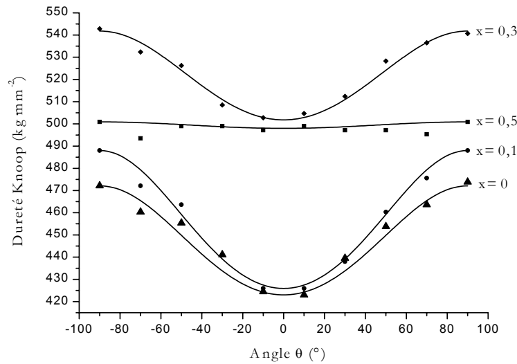
Figure 3. 11. Variation de la dureté Knoop suivant l'orientation cristalline.
