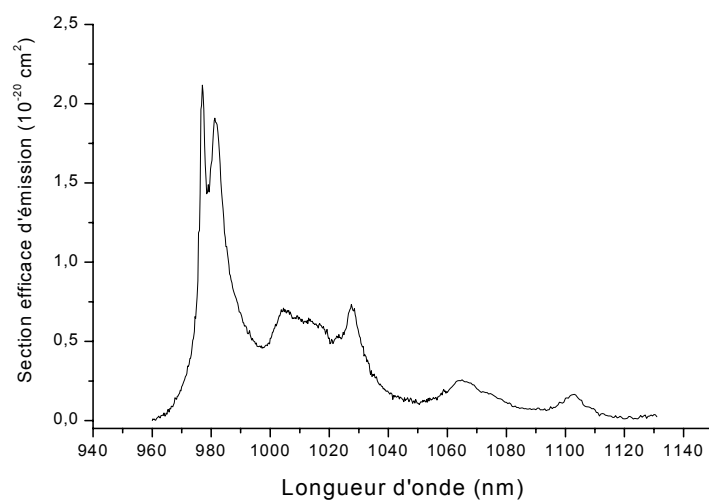
Figure 4. 40. Section efficace de fluorescence du composé \text{Gd}_2\text{O}_3:\text{Yb}^{3+} .
