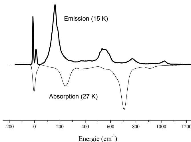
Figure 4. 34. Spectres d'émission et d'absorption de \text{Sc}_2\text{SiO}_5: \text{Yb}^{3+} à basse température (77 K). En abscisse, l'énergie de la transition fondamentale entre les premiers sous-niveaux Stark des multiplets ^2\text{F}_{7/2} et ^2\text{F}_{5/2} sert de référence.
