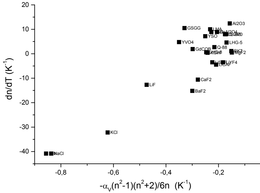
Figure 4. 20. Coefficient thermo-optique dn/dT en fonction du coefficient d'expansion volumique ( \gamma=1/3 ).
