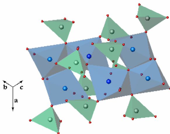
Figure 4. 26. Structure cristalline de l'orthosilicate \text{Sc}_2\text{SiO}_5 .
