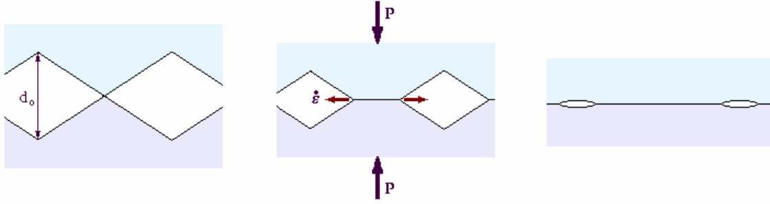
Figure 2.31 Interface entre les cristaux dans le modèle de Hamilton.
