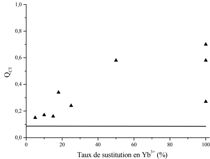
Figure 1.25. Evolution de la charge thermique (mesurée par calorimétrie) dans différents échantillons monocristallins de YAG:Yb. On notera la grande dispersion des mesures. La charge thermique minimale déduite de l'efficacité quantique est représentée par la droite horizontale Q_{CT}=9\% . D'après [51].
