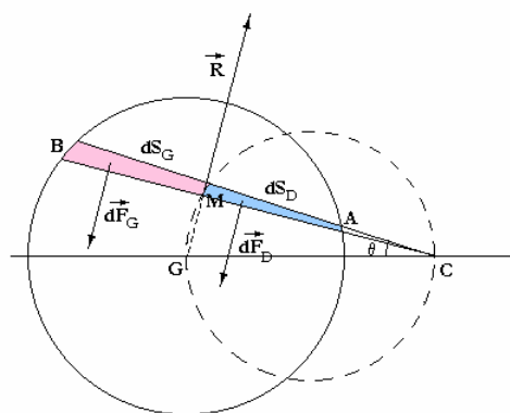
Figure 2.16 Couple des forces de frottement
