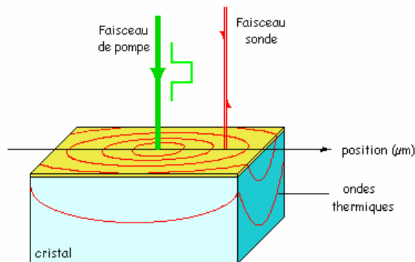
Figure 4. 8. Position relative des faisceaux sonde et de pompe à la surface d'un échantillon.
