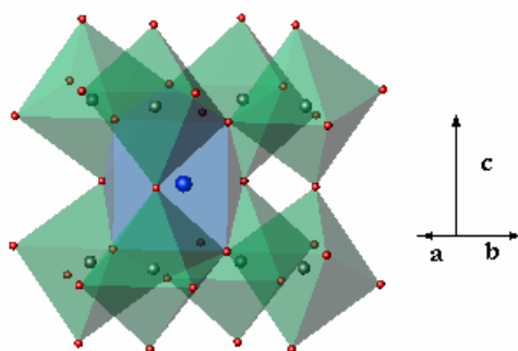
Figure 4. 23. Empilements des polyèdres de coordination [\text{GdO}_8] et [\text{AlO}_6] dans la matrice pérovskite \text{GdAlO}_3 .
