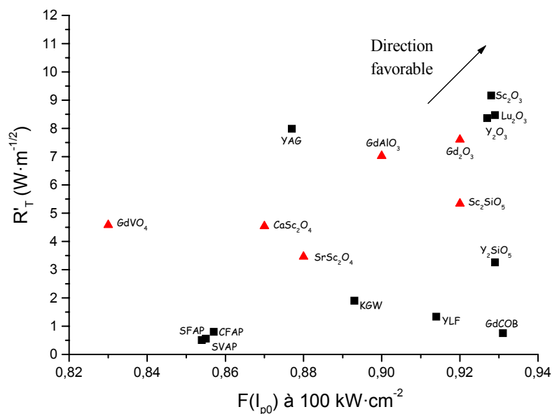
Figure 4. 49. Facteur de mérite pour une intensité de 100 kW cm -2 . Les composés étudiés dans ce travail sont représentés par les triangles rouges.
