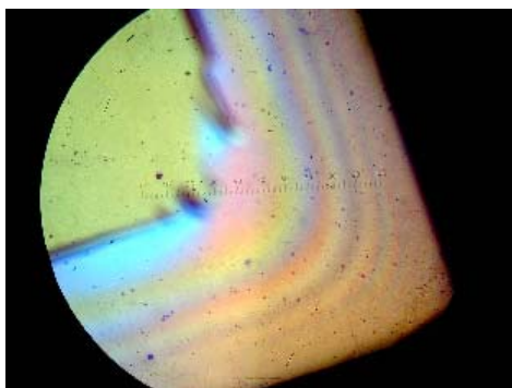
Figure 2.29 Cliché montrant les anneaux de Newton en périphérie de la zone contactée (en haut à gauche) entre un cristal de YAG et un cristal de SYS dopé \text{Yb}^{3+} .
