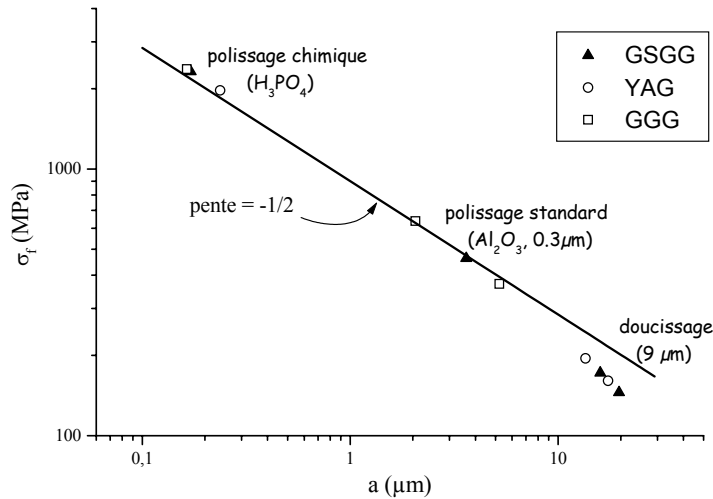
Figure 2.21 Contrainte maximale avant rupture \sigma_f de trois grenats en fonction de la profondeur des rayures. La loi de Griffith est superposée aux points expérimentaux de la référence [10].
