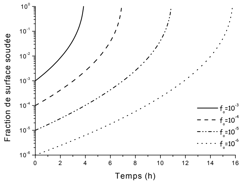
Figure 2.34 Fraction de surface soudée en fonction du temps ( T_s=600^\circ\text{C} ) pour différents rapports de surface contactée à froid f_o . On suppose d_o=5 \text{ \AA} .
