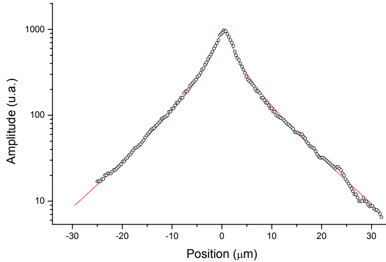
Figure 4. 9. Evolution expérimentale de l'amplitude du faisceau sonde réfléchi par une surface métallique déposée en surface d'un cristal de \text{Sc}_2\text{SiO}_5:\text{Yb}^{3+} 1 %, en fonction de la distance entre les faisceaux de pompe et de sonde. L'évolution théorique obtenue par ajustement est superposée en trait plein.
