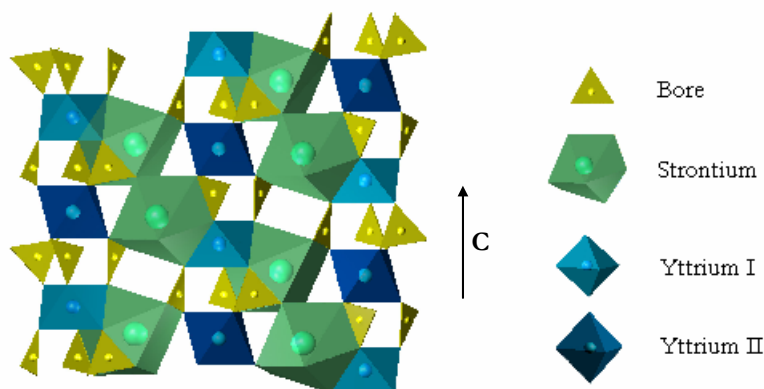
Figure 3. 1. Structure de la matrice cristalline \text{Sr}_3\text{Y}(\text{BO}_3)_3 . On distingue les empilements verticaux le long de l'axe c des octaèdres \text{YO}_6 et les polyèdres de coordination du strontium intercalés entre ces chaînes.
