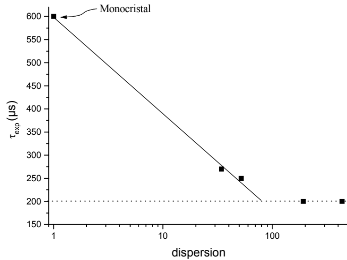
Figure 1. 7. Temps de vie expérimental de \text{KYb(WO}_4)_2 pour différentes valeurs de la dispersion dans l'éthylène glycol. Pour de fortes dispersions, on obtient le temps de vie intrinsèque de l'ytterbium (200 \mu\text{s} ). Ce temps de vie est à comparer au temps de vie intrinsèque de 300 \mu\text{s} obtenu dans des échantillons dilués de \text{KY(WO}_4)_2\text{:Yb} . Données expérimentales d'après [20].
