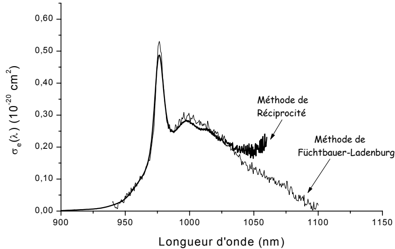
Figure 3. 18. Comparaison des sections efficaces d'émission stimulée d'un monocristal de (\text{Sr}_{0.7}\text{Ca}_{0.3})_3\text{Y}(\text{BO}_3)_3:\text{Yb}^{3+} calculées par la méthode de Füchtbauer-Ladenburg et celle utilisant le principe de réciprocité. La valeur du temps de vie effectif déduit de cette comparaison est de 1.7 ms.
