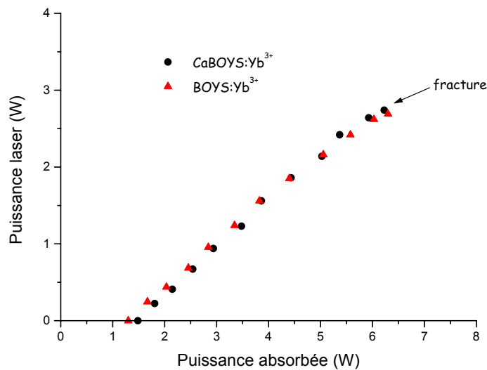
Figure 3. 21. Test laser comparatif sous pompage par diode fibrée sur des cristaux de BOYS :Yb 3+ et de BOYS:Ca 2+ :Yb 3+ traités anti-reflets.
