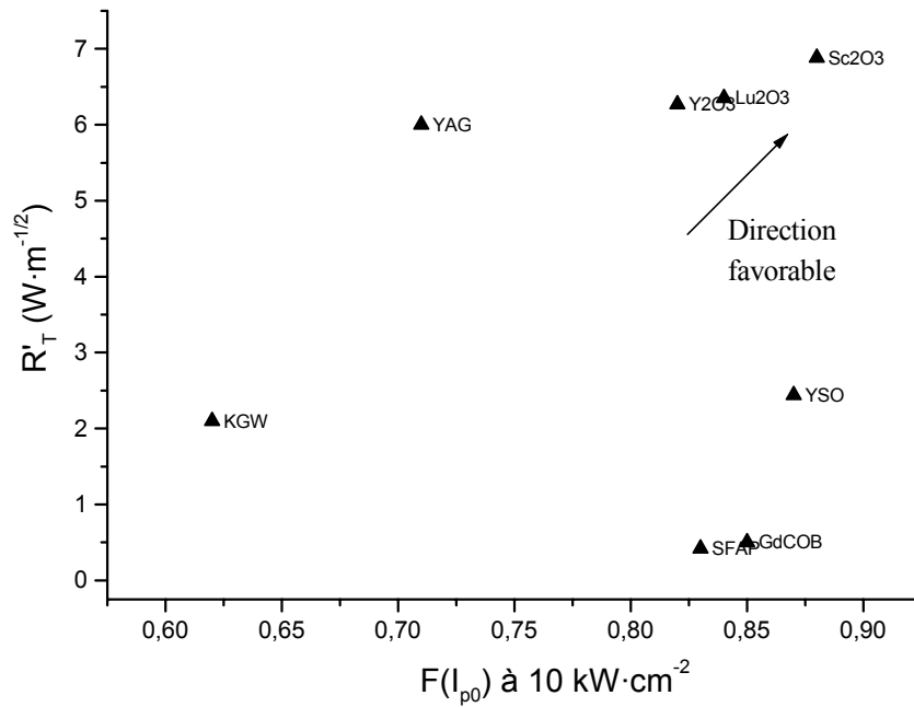
Figure 1. 29. Facteur de mérite pour un éclairement de 10 \text{ kW} \cdot \text{cm}^{-2} .
