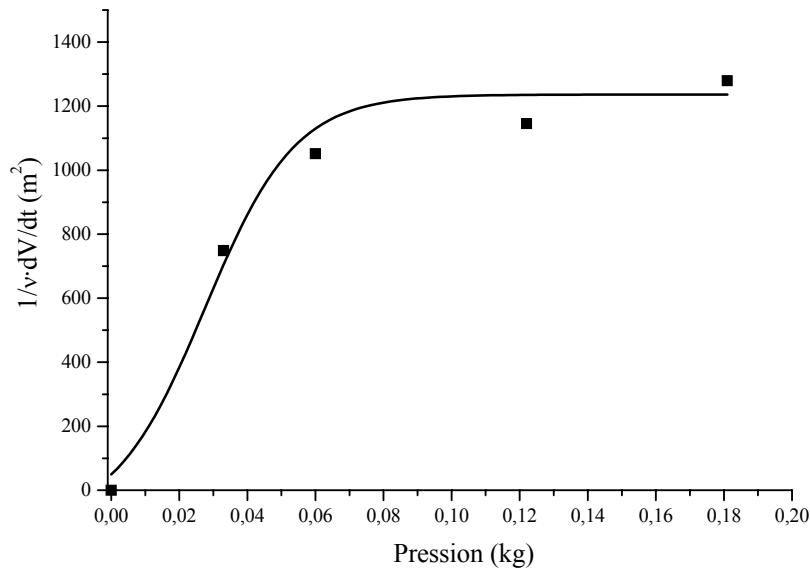
Figure 2.20 Evolution de la vitesse d'usure en fonction de la pression appliquée à l'échantillon.
