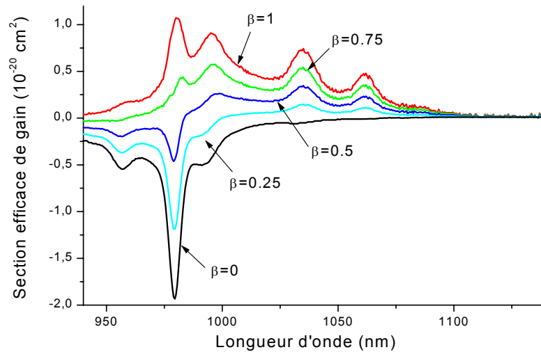
Figure 4. 48. Section efficace de gain \sigma_{\text{gain}}(\lambda) dans \text{Sc}_2\text{SiO}_5:\text{Yb}^{3+} à température ambiante pour différents taux d'inversion de population. Les sections efficaces d'émission stimulée et d'absorption \sigma_e(\lambda) et \sigma_a(\lambda) correspondent aux courbes \sigma_{\text{gain}}(\lambda) avec \beta=1 et 0 respectivement.
