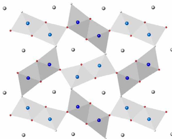
Figure 4.25. Structure cristalline des composés \text{CaSc}_2\text{O}_4 et \text{SrSc}_2\text{O}_4 projetée suivant l'axe c . Les deux sites du scandium sont représentés dans des polyèdres de contrastes différents. Les ions alcalino-terreux occupent les larges sites entre les groupes d'octaèdres [\text{ScO}_6] .
