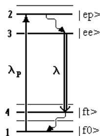
Figure 1. 14. Fonctionnement d'un laser quasi-3-niveaux ( |f0\rangle et |ft\rangle désignent les états fondamentaux initial et terminal du processus laser, et les états |ee\rangle et |ep\rangle sont les états excités émetteur et de pompage, respectivement).
