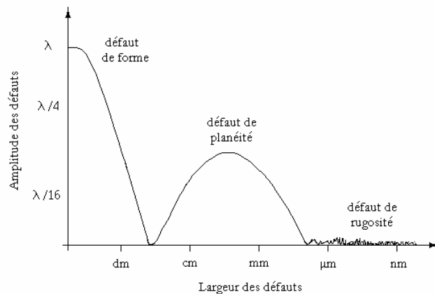
Figure 2.27. Echelle et ordres de grandeurs des défauts d'une surface optique.
