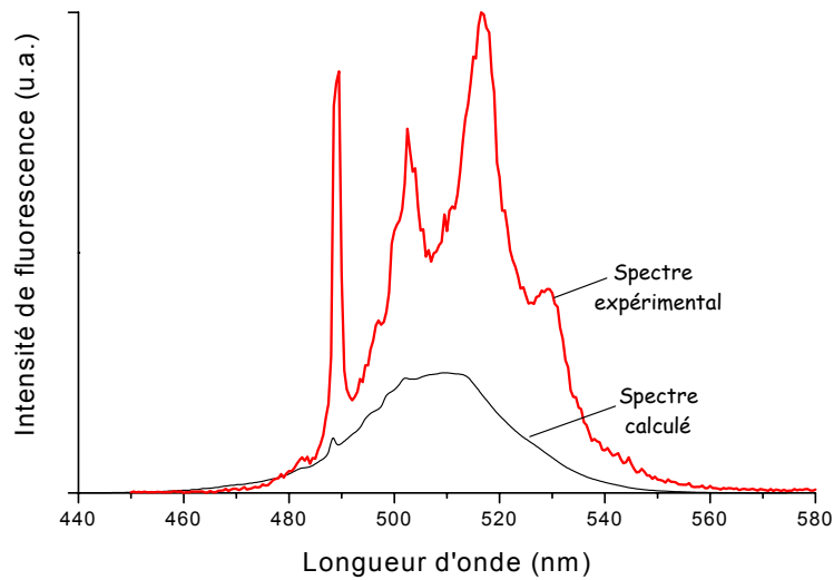
Figure 1. 12. Mise en évidence du phénomène de luminescence coopérative dans \text{Ca}_4\text{Y}(\text{BO}_3)_3\text{O}:\text{Yb}^{3+} 35%.
