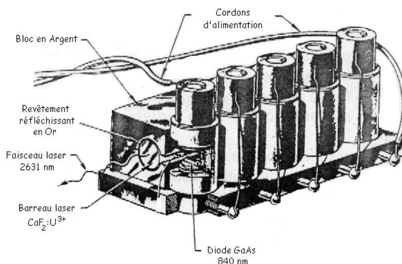
Figure 1. Premier laser solide pompé par diode : \text{CaF}_2:\text{U}^{3+} [3]. On notera l'utilisation d'un bloc en argent pour refroidir le laser.
