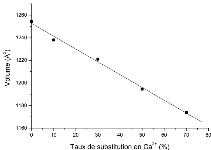
Figure 3. 6. Vérification de la loi de Vegard sur les composés de formule (\text{Sr}_{1-x}\text{Ca}_x)_3\text{Y}(\text{BO}_3)_3:\text{Yb}^{3+} .
