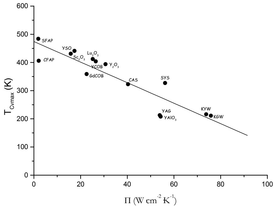
Figure 1. 28. Corrélation entre la température T_{Cvmax} et le coefficient \Pi .
