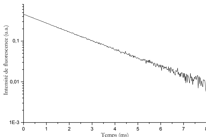
Figure 3. 19. Déclin de fluorescence du niveau excité de l'ion \text{Yb}^{3+} dans le composé (\text{Sr}_{0,7}\text{Ca}_{0,3})_3\text{Y}(\text{BO}_3)_3 : \text{Yb}^{3+} .
