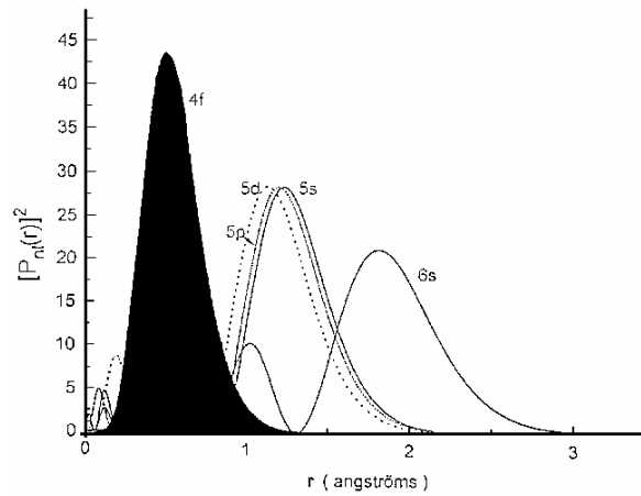
Figure 1. 1. Probabilité de présence radiale des électrons en fonction de leur distance au noyau pour les orbitales 4f, 5d, 5s, 5p et 6s.
