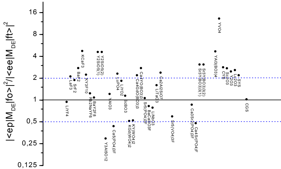
Figure 1. 17. Vérification de l'égalité des moments de transition.
