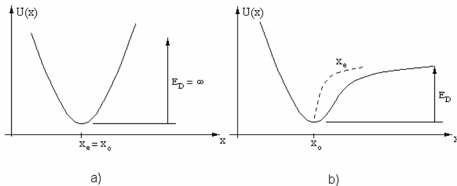
Figure 4. 13. Evolution du potentiel au voisinage d'un atome. a) Potentiel harmonique, b) Potentiel de Morse (anharmonique). Sur la figure b, on a repéré la position d'équilibre x_e pour chaque énergie U de la liaison chimique.
