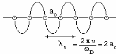
Figure B. 1. Fréquence de Debye dans une chaîne monoatomique linéaire
