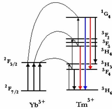
Figure 1. 10. Addition de Photons par Transfert d'Energie (APTE). La longue durée de vie des niveaux ^3\text{F}_4 et ^3\text{H}_4 permet les deuxième et troisième transferts. Les longueurs d'onde des émissions du thulium sont environ \lambda(^1\text{G}_4 \rightarrow ^3\text{H}_5) = 790 \text{ nm} , \lambda(^1\text{G}_4 \rightarrow ^3\text{F}_4) = 650 \text{ nm} , \lambda(^1\text{G}_4 \rightarrow ^3\text{H}_6) = 477 \text{ nm} , \lambda(^3\text{H}_4 \rightarrow ^3\text{H}_6) = 779 \text{ nm} , \lambda(^3\text{F}_4 \rightarrow ^3\text{H}_6) = 1800 \text{ nm} .
