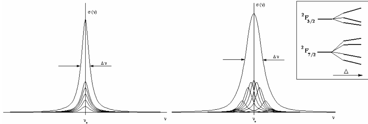
Figure 1. 5. Elargissements homogène et inhomogène d'une raie. On a représenté schématiquement le diagramme des niveaux d'énergie de l'ytterbium pour une distribution de sites \Delta .
