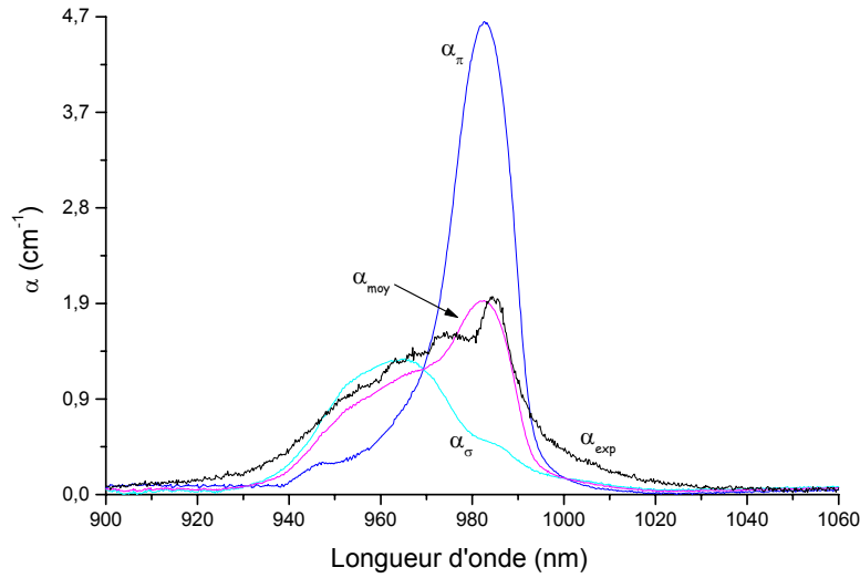
Figure 4. 36. Spectres d'absorption de \text{GdVO}_4:\text{Yb}^{3+} \alpha_\sigma(\lambda) et \alpha_\pi(\lambda) obtenus en lumière polarisée. Nous avons également représenté le spectre moyen \alpha_{\text{moy}}(\lambda) obtenu à l'aide des spectres polarisés et le comparons au spectre expérimental \alpha_{\text{exp}}(\lambda) non polarisé.
