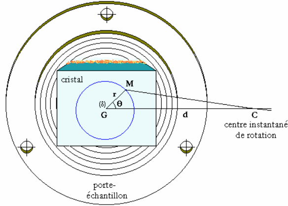
Figure 2.12. Cristal en cours de surfacage collé sur son porte-échantillon (cf. texte).
