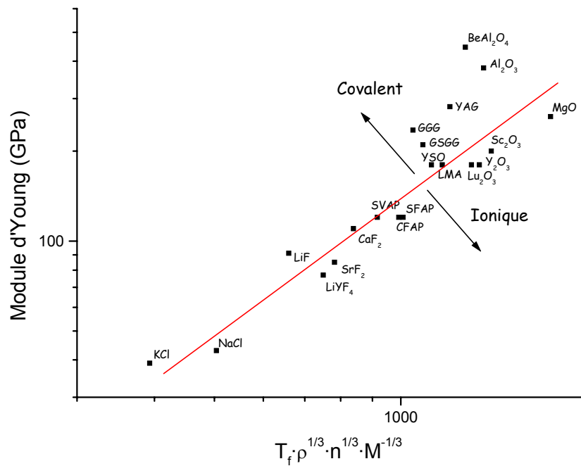
Figure 4. 14. Relation entre le module d'Young E et le paramètre de rigidité T_f \cdot \rho^{1/3} \cdot n^{1/3} \cdot M^{-1/3} pour différents matériaux.
