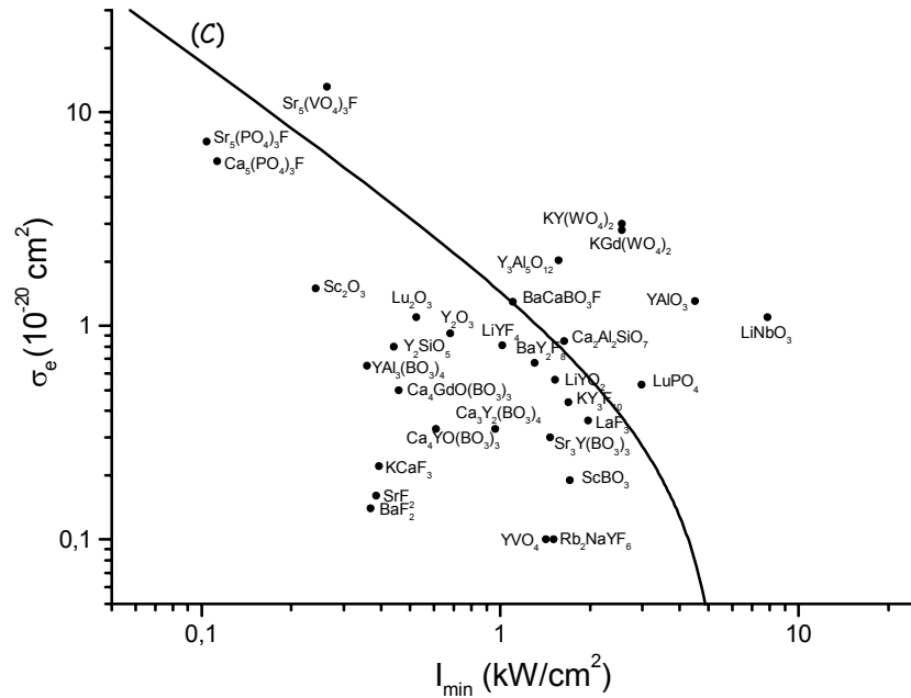
Figure 1.18. Diagramme \sigma_e vs I_{\min} . La courbe noire représente l'évolution théorique de \sigma_e = f(I_{\min}) pour des paramètres moyens.
