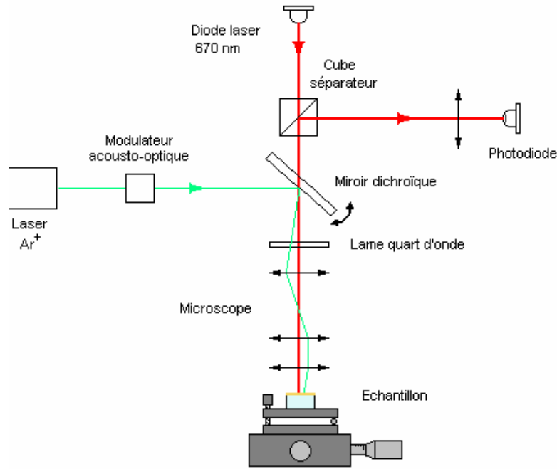
Figure 4. 4. Schéma du microscope à photoréflexance.
