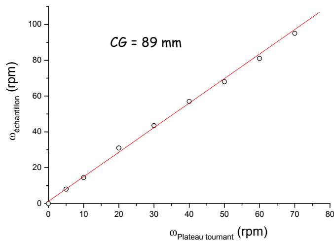
Figure 2.11 Détermination expérimentale de la distance CG entre l'échantillon et le centre instantané de rotation. Les points représentés correspondent au douçissage sur le plateau en fonte de la polisseuse PM-5.
