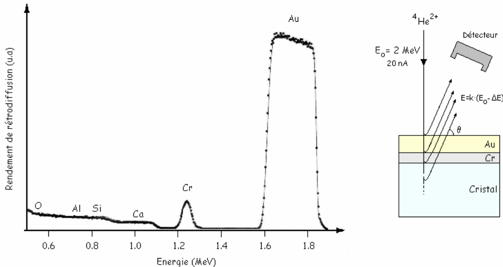
Figure 4. 7. Spectre RBS du revêtement métallique déposé sur un cristal de \text{Ca}_2\text{Al}_2\text{SiO}_7 . Le spectre simulé en fonction de la nature des couches et du substrat est superposé aux points expérimentaux. Les épaisseurs des dépôts métalliques obtenues par cet ajustement aux données expérimentales sont de 170 \pm 4 nm pour l'or et 36 \pm 2 nm pour le chrome. A droite, le principe de cette mesure est représenté schématiquement : des particules \alpha de grande énergie cinétique E_0 entrent en collision avec les atomes de l'échantillon. On mesure le nombre et l'énergie des particules \alpha rétrodiffusées dans une direction \theta donnée. Le coefficient de rétrodiffusion k d'un atome cible est une fonction de \theta et de la masse de cet atome. On tient compte également de la perte d'énergie \Delta E des particules \alpha induite par la traversée des couches atomiques supérieures lors du retour dans la direction du détecteur.
