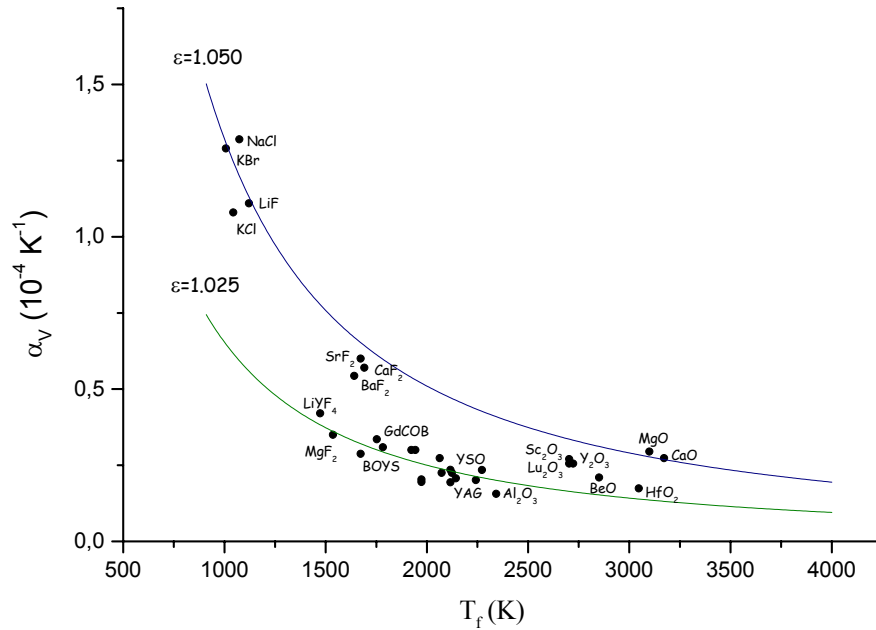
Figure 4. 16. Evolution du coefficient d'expansion thermique avec la température de fusion pour différents matériaux cristallins. On a pris pour les deux ajustements n=1.4 .
