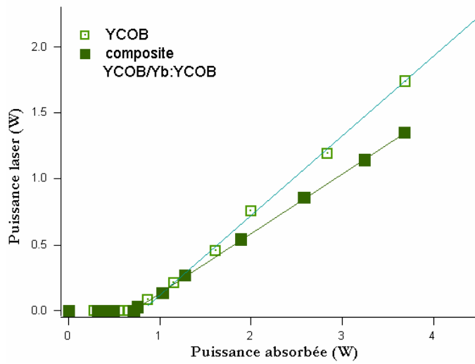
Figure 2. 39 Performances laser comparées d'un cristal YCOB:Yb³⁺ et d'un cristal composite YCOB:Yb³⁺ 15 % || YCOB sous pompage par diode.
