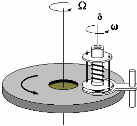
Figure 2.9 Vue schématique d'un tour automatique. On reconnaît le plateau tournant à la vitesse \Omega , le porte-échantillon en rotation libre autour de son axe de symétrie, retenu par une fourche fixe dans le référentiel du laboratoire. La pression sur l'échantillon peut être réglée à l'aide d'un ressort visualisé sur la figure.
