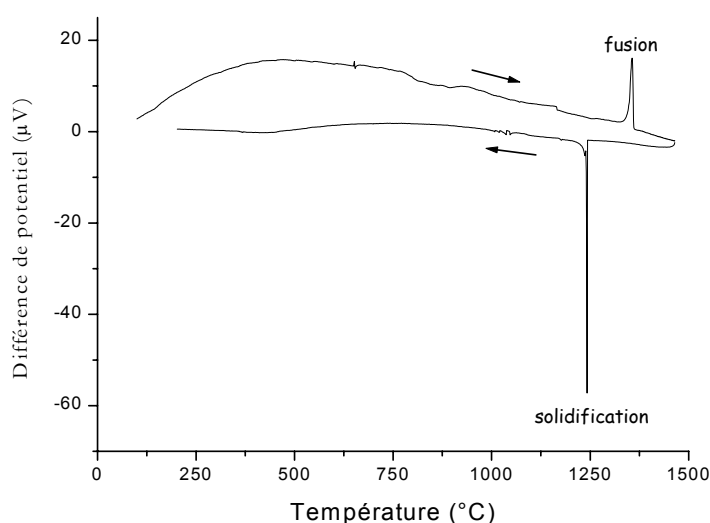
Figure 3. 7. Diagramme d'analyse thermique différentielle d'un échantillon de (Sr_{1-x}Ca_x)_3(Y_{1-y}Yb_y)(BO_3)_3 , x=0.3 , y=0.15 .
