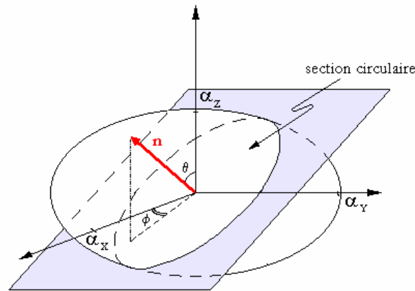
Figure 2.37 Ellipsoïde de dilatation d'un cristal anisotrope.
