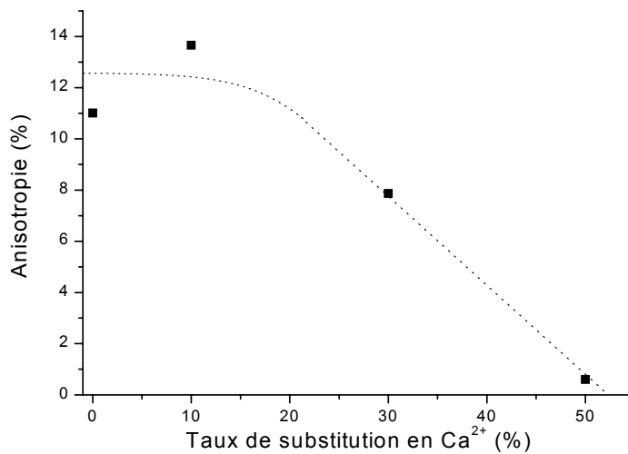
Figure 3. 13. Evolution de l'anisotropie de dureté avec le taux de substitution en calcium.
