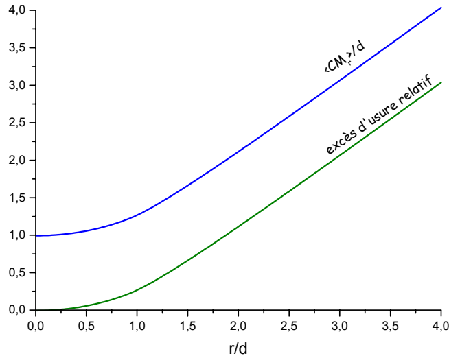
Figure 2.13 Variation de \langle CM_r \rangle / d en fonction de r/d .
