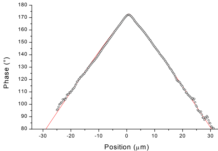
Figure 4. 10. Evolution expérimentale de la phase du faisceau sonde réfléchi par une surface métallique déposée en surface d'un cristal de \text{Sc}_2\text{SiO}_5:\text{Yb}^{3+} 1 %, en fonction de la distance entre les faisceaux de pompe et de sonde. L'évolution théorique obtenue par ajustement est superposée en trait plein.
