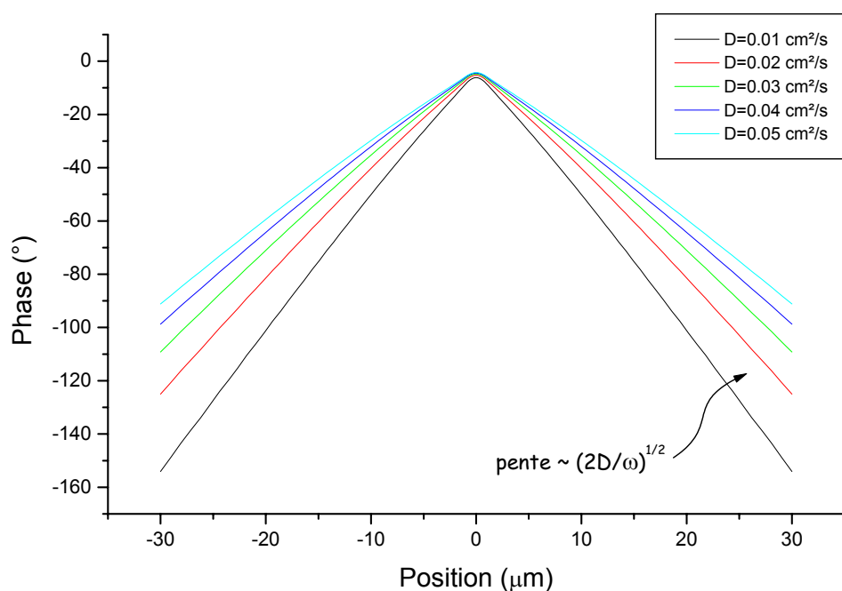
Figure 4. 6. Evolution théorique du déphasage du faisceau sonde réfléchi par rapport à l'excitation en fonction de la distance entre les faisceaux de pompe et de sonde. On a fait varier la valeur de la diffusivité thermique D de l'échantillon.
