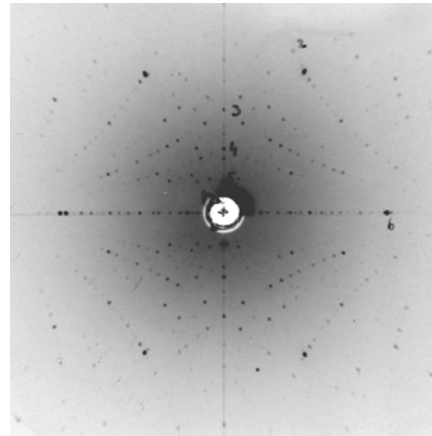
Figure 2.2 Cliché de diffraction de rayons X obtenu par la méthode de Laue « en retour » sur un monocristal de \text{SrY}_4(\text{SiO}_4)\text{O}:\text{Yb} . On distingue la symétrie sénaire de la structure de cette apatite silicatée.
