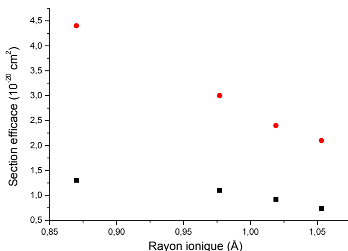
Figure 4. 42. Evolution des sections efficaces d'émission à 1030 nm (■) et d'absorption à 980 nm (●) dans les oxydes \text{Sc}_2\text{O}_3 , \text{Lu}_2\text{O}_3 , \text{Y}_2\text{O}_3 , \text{Gd}_2\text{O}_3 dopés à l'ytterbium en fonction de la taille du site dodécaédrique substitué.
