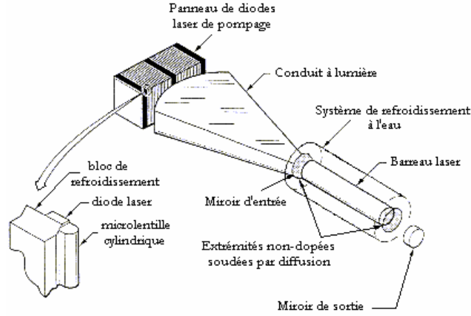
Figure 1. 22. Système laser de puissance utilisant un barreau composite soudé par diffusion. D'après [47].
