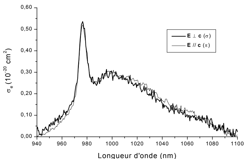
Figure 3. 17. Spectres d'émission en lumière polarisée à température ambiante sur un monocristal de (\text{Sr}_{0,7}\text{Ca}_{0,3})_3\text{Y}_{0,85}\text{Yb}_{0,15}(\text{BO}_3)_3 .
