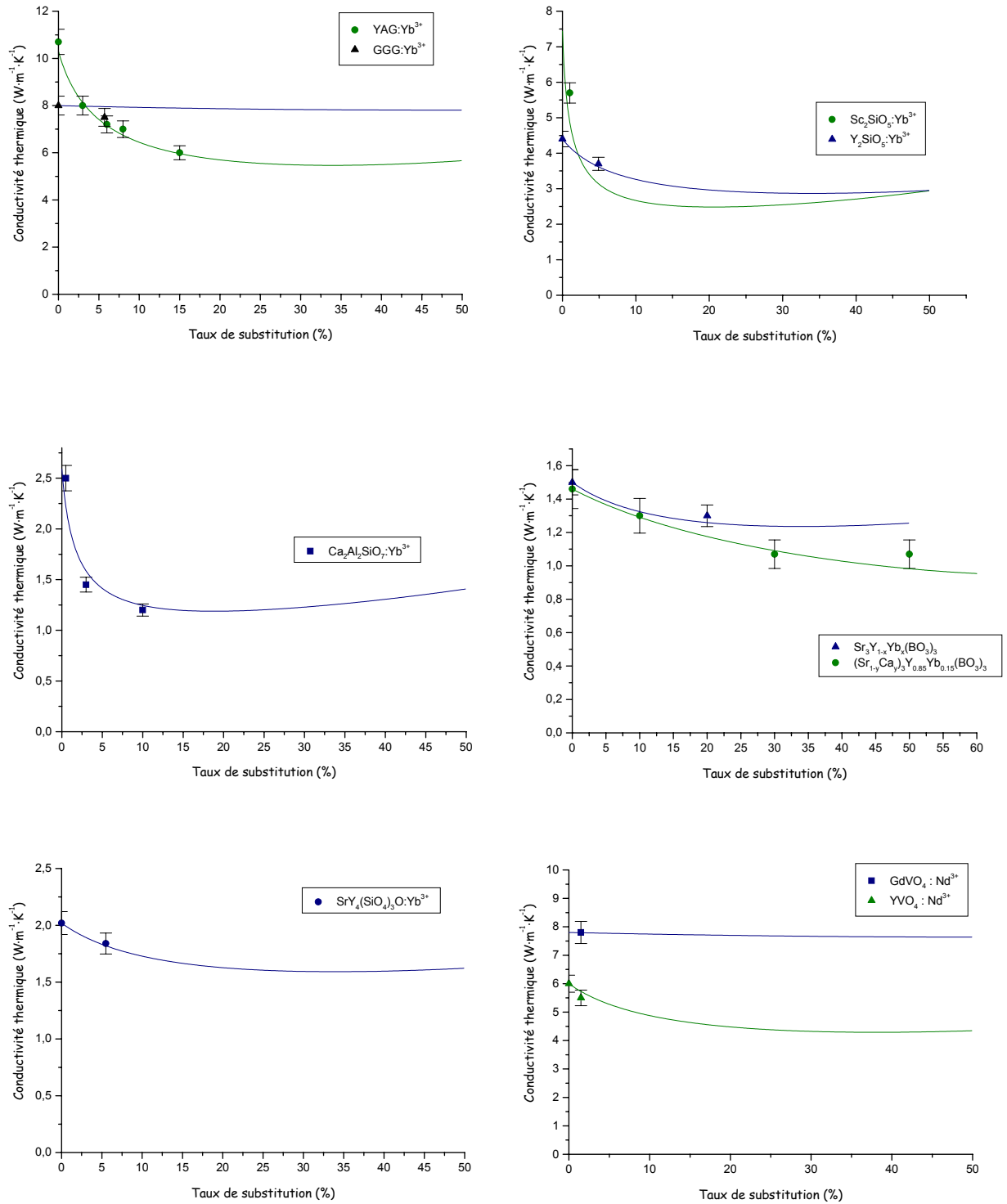
Figure 4.11. Evolution de la conductivité thermique avec le taux de substitution en impuretés (Yb³⁺, Nd³⁺ et Ca²⁺).
