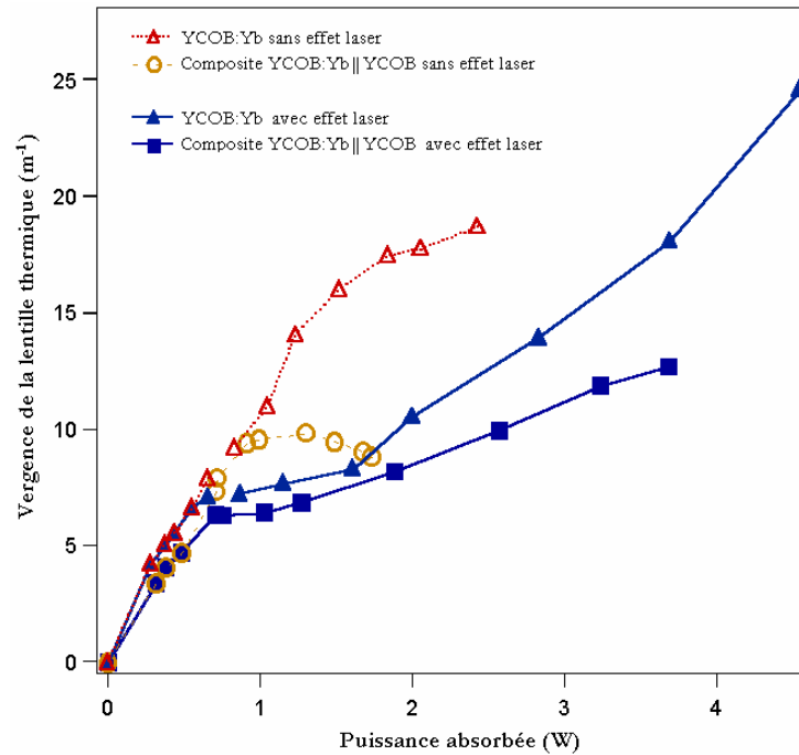
Figure 2. 40 Réduction de l'effet de lentille thermique dans un cristal composite, comparaison avec un cristal non-soudé.
