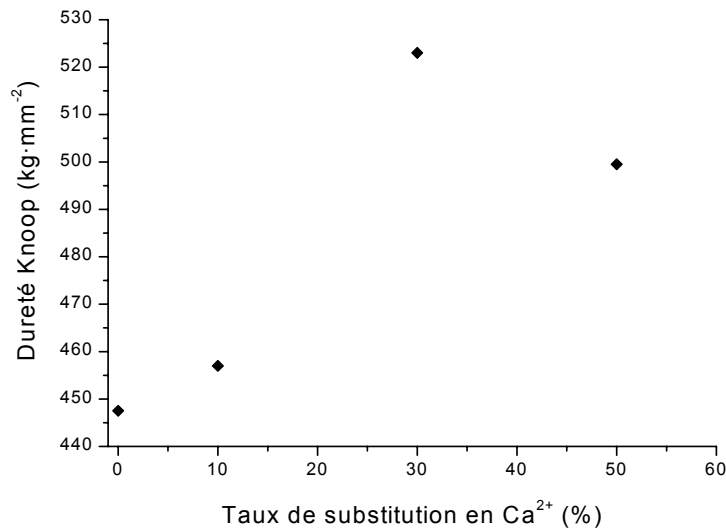
Figure 3. 12. Evolution de la dureté moyenne avec le taux de substitution en calcium.
