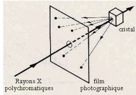
Figure 2.1 Montage expérimental de diffraction des rayons X par la méthode de Laue « en retour ».
