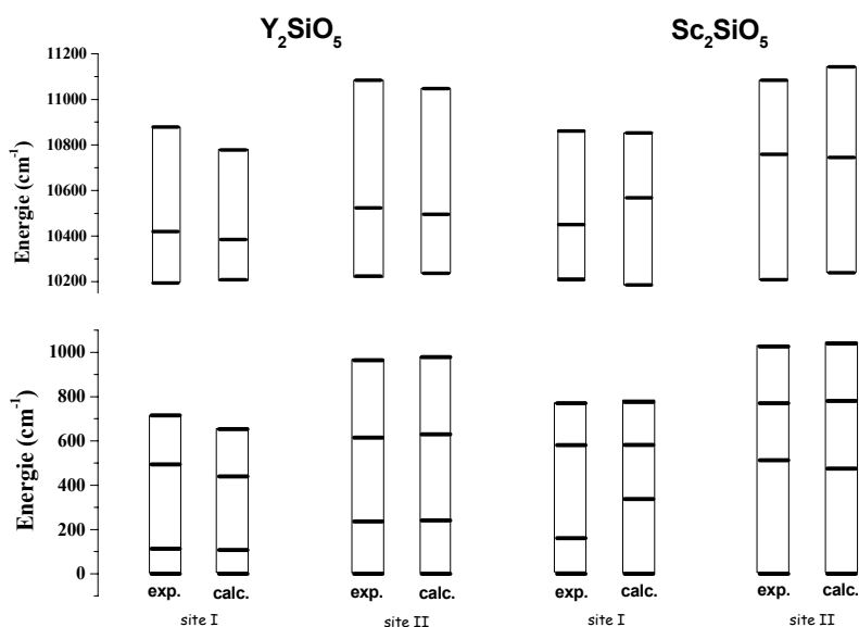
Figure 4. 35. Niveaux d'énergie expérimentaux et calculés dans les composés Sc_2SiO_5:Yb^{3+} et Y_2SiO_5:Yb^{3+} . Deux sites cristallographiques sont possibles pour la substitution de l'yttrium et sont effectivement observés expérimentalement.
