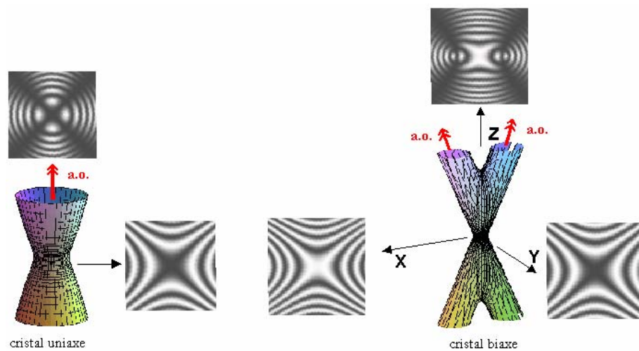
Figure 2.6 Surfaces d'égale différence de phase et figures d'interférences pour des milieux uniaxes et biaxes.
