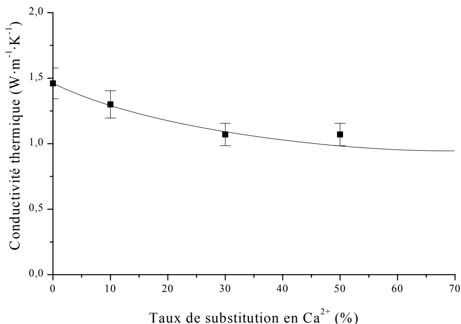
Figure 3. 14. Evolution de la conductivité thermique moyenne des solutions solides (\text{Sr}_{1-x}\text{Ca}_x)_3\text{Y}(\text{BO}_3)_3:\text{Yb}^{3+} en fonction du taux de substitution en calcium.
