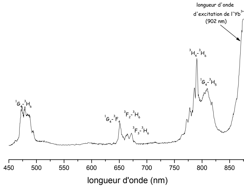
Figure 1. 9. Mise en évidence d'un effet d'up-conversion dans \text{Y}_2\text{SiO}_5:\text{Yb}^{3+} .
