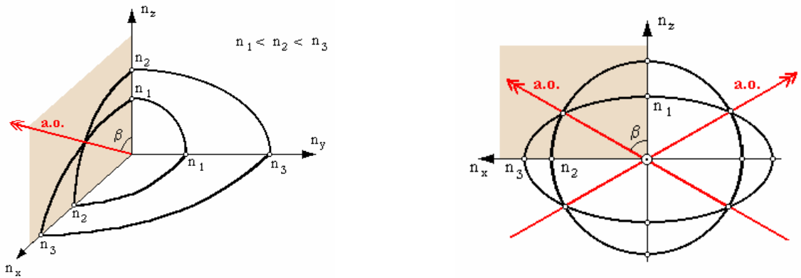
Figure 2.3 Surface des indices d'un cristal biaxe
