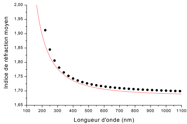
Figure 4. 19. Comparaison de la dispersion expérimentale moyenne dans le GdCOB et du modèle de dispersion décrit plus haut. La fréquence de résonance effective choisie est de 110 nm.
