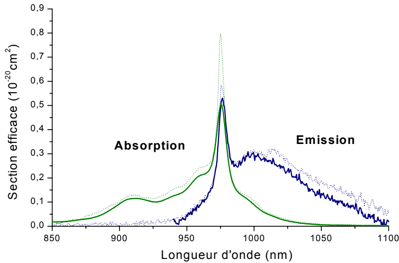
Figure 3. 20. Comparaison des spectres d'absorption et d'émission du BOYS :Yb 3+ (pointillés) et du composé substitué (\text{Sr}_{0.7}\text{Ca}_{0.3})_3\text{Y}(\text{BO}_3)_3 : \text{Yb}^{3+} (trait plein). (Cette comparaison est réalisée dans des états de polarisation identiques).
