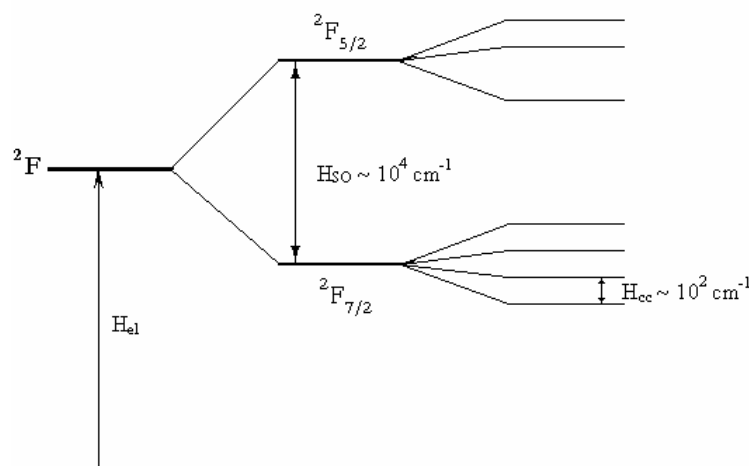
Figure 1. 2. Eclatement de la configuration 4f 13 de l'ion \text{Yb}^{3+} sous l'effet des différents termes du Hamiltonien.
