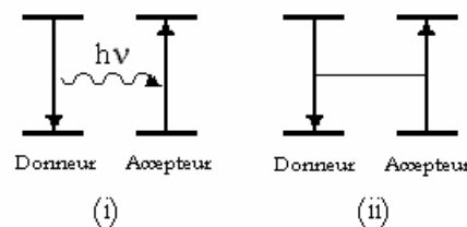
Figure 1. 6. Processus d'interaction entre deux ions \text{Yb}^{3+} par (i) émission et réabsorption d'un photon, ou par (ii) interaction inter-ionique de nature multipolaire électrique,
