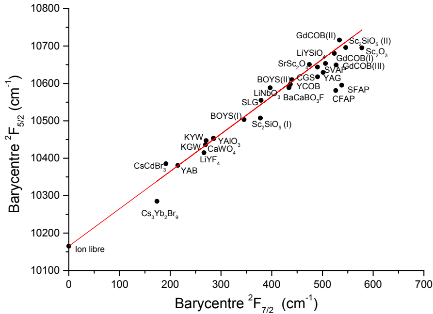
Figure 1. 4. Diagramme des barycentres. D'après [6]
