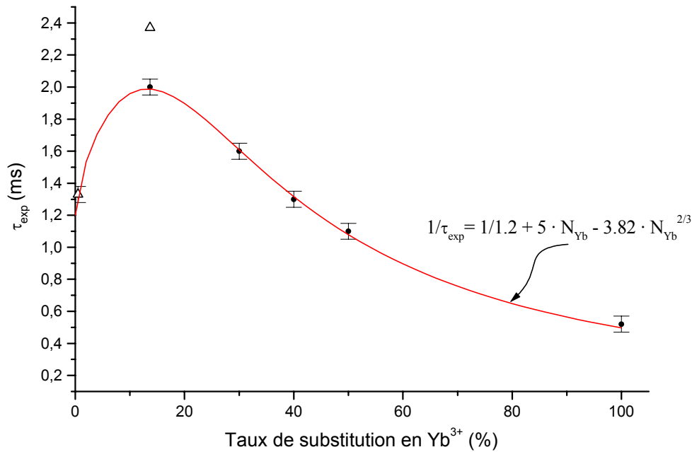
Figure 1. 8. Evolution du temps de vie expérimental dans \text{Sr}_3\text{Y}(\text{BO}_3)_3:\text{Yb}^{3+} .
