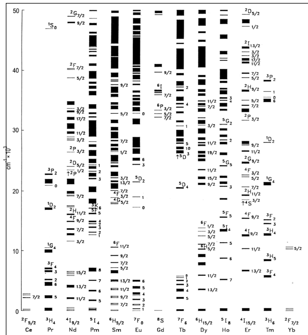
Figure 1. 3. Niveaux d'énergie ^{2S+1}L_J des ions lanthanides trivalents dans les chlorures. D'après [1].
