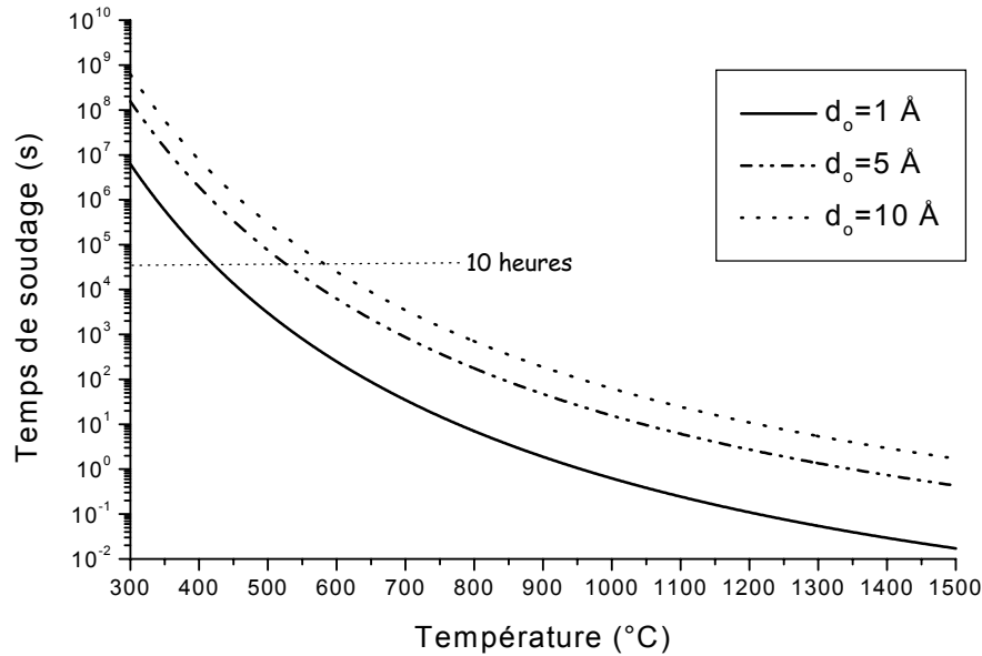
Figure 2.33. Temps de soudage t_s en fonction de la température T_s . On notera l'effet de la rugosité d_o . Le rapport des surfaces contactées choisi est de f_o=10^{-4} .
