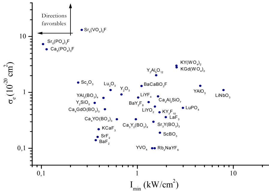
Figure 1. 16. Critère de mérite proposé par L.D. DeLoach et al. dans la référence [38] complété
