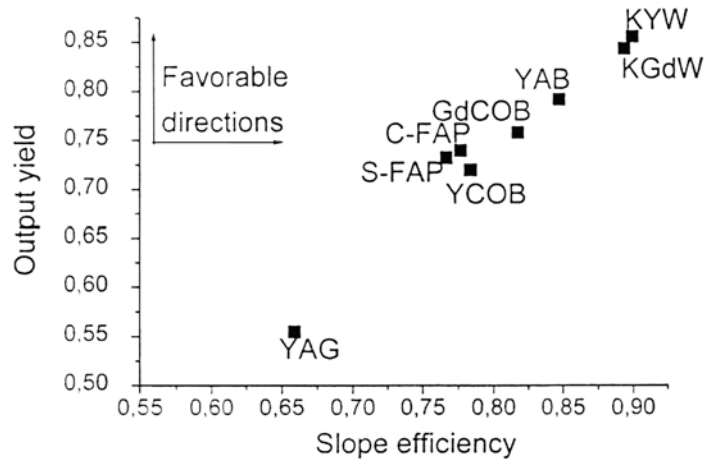
Figure 1. 21. Prévision des performances laser de quelques milieux à gain dopés à l'Yb 3+ .
