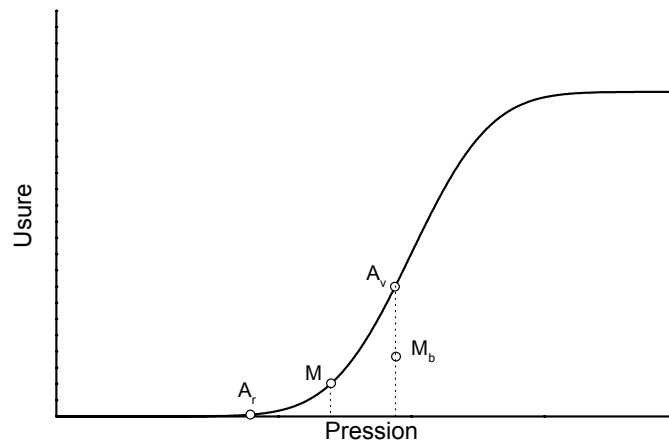
Figure 2.22 Evolution qualitative de l'usure en fonction de la pression
