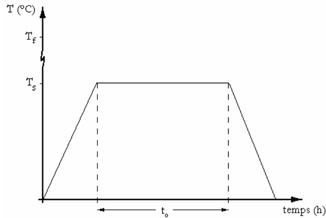
Figure 2.35 Programme de température pour le soudage par diffusion.
