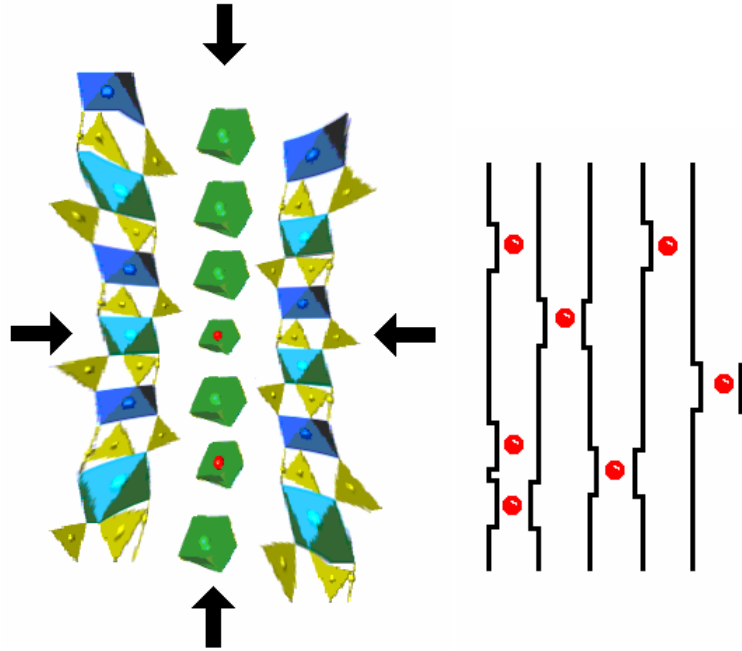
Figure 3. 4. Représentations schématiques de l'effet de la substitution partielle et statistique du strontium par le calcium sur la structure du BOYS. On distingue, entre les empilements verticaux des octaèdres [\text{YO}_6] , les polyèdres de coordination du strontium et du calcium. Sur la figure de droite, seuls les ions calcium sont représentés.
