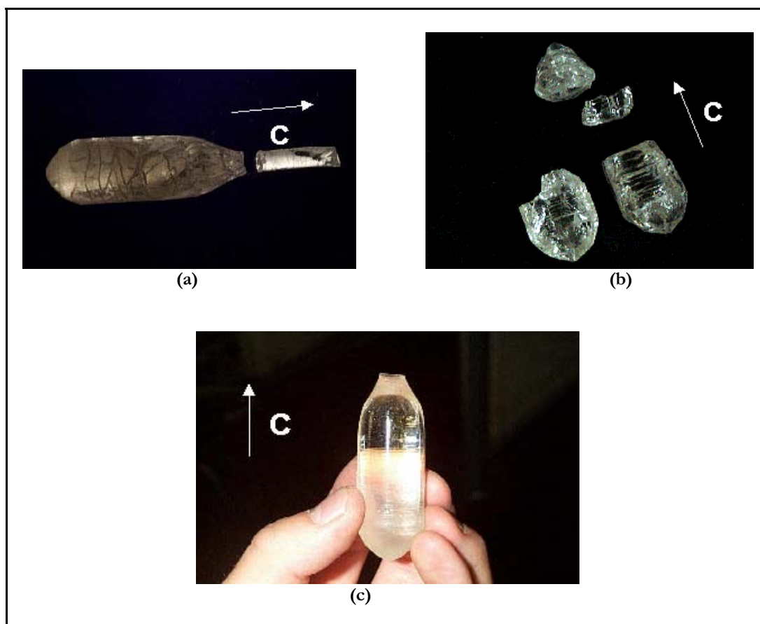
Figure 3. 9. Cristaux de composition (\text{Sr}_{1-x}\text{Ca}_x)_3(\text{Y}_{0.85}\text{Yb}_{0.15})(\text{BO}_3)_3 élaborés par la méthode de Czochralski. (a) x=0.1 , (b) x=0.5 , (c) x=0.3 .
