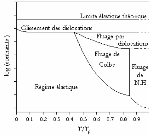
Figure 2.32. Mécanismes de fluage en fonction de la contrainte et de la température (normalisée à la température de fusion T_f ). L'étendue des différents domaines est qualitative. Fluage de N.H. : fluage de Nabarro-Herring. La limite élastique théorique est de l'ordre de 10^{-1} \cdot E .
