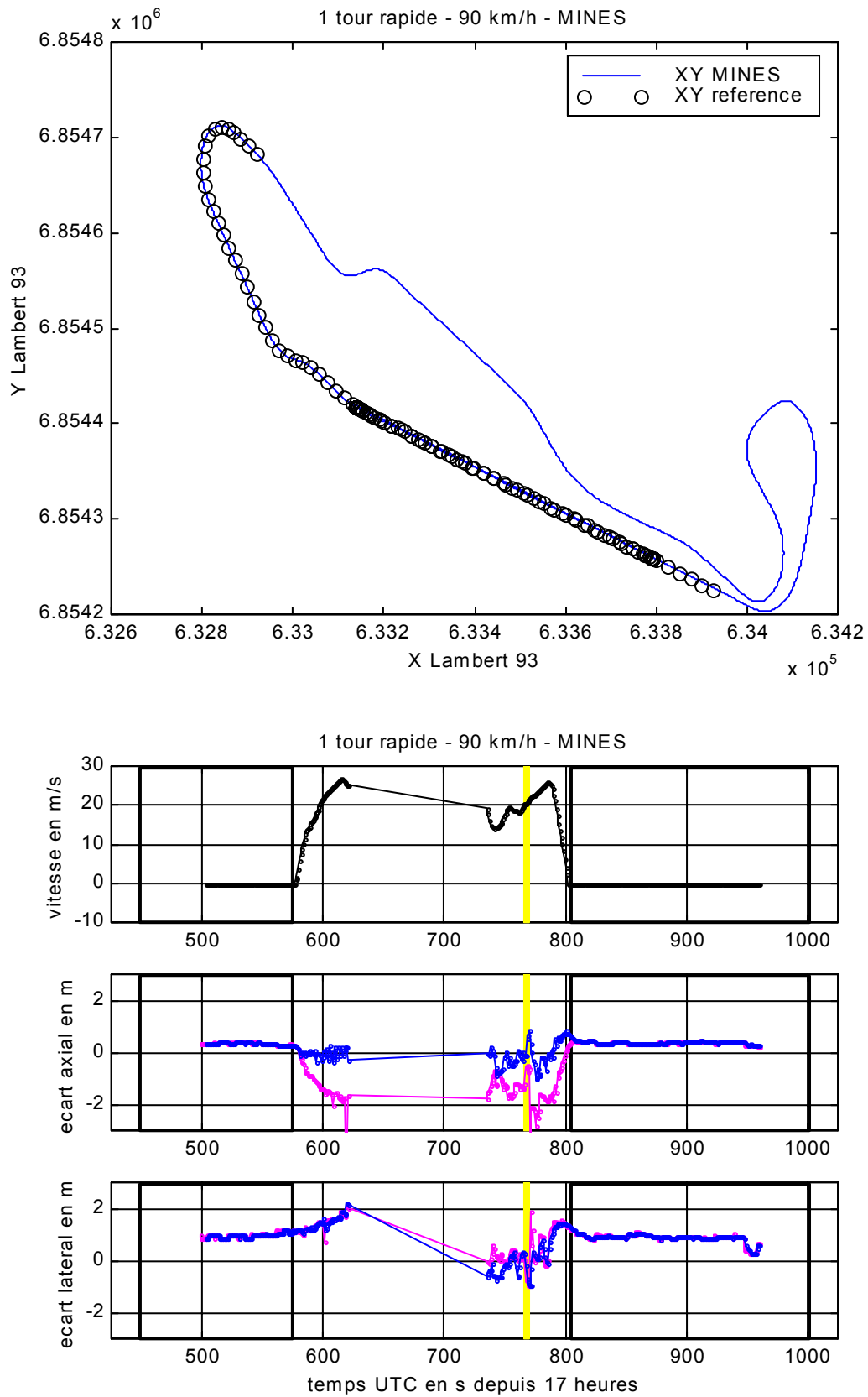
Figure 71: Graphique des écarts axial et latéral (vitesse rapide), pour sorties prototype (—) et DGPS (—) par rapport à la référence PPK.
