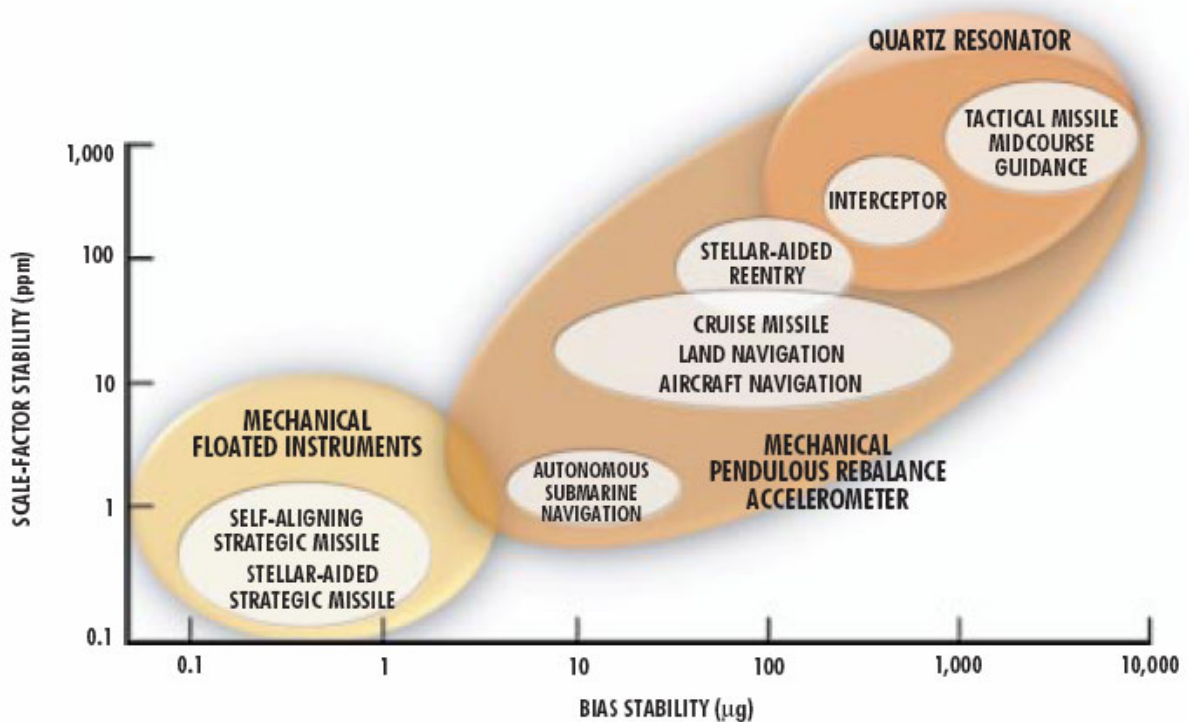
Figure 13: Applications courantes de la technologie d'accéléromètre
