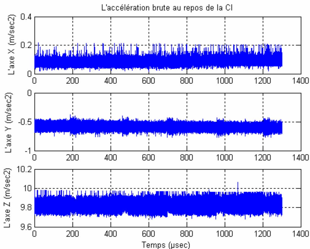
Figure 45: Mesures des accéléromètres bruts au repos
