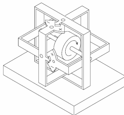
Figure 7: Gyroscopie Mécanique
