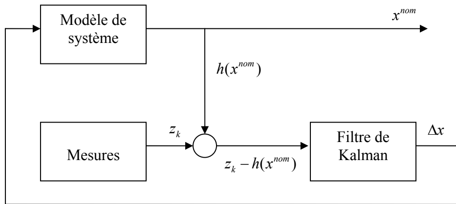
Figure 23: Filtre de Kalman Etendu
