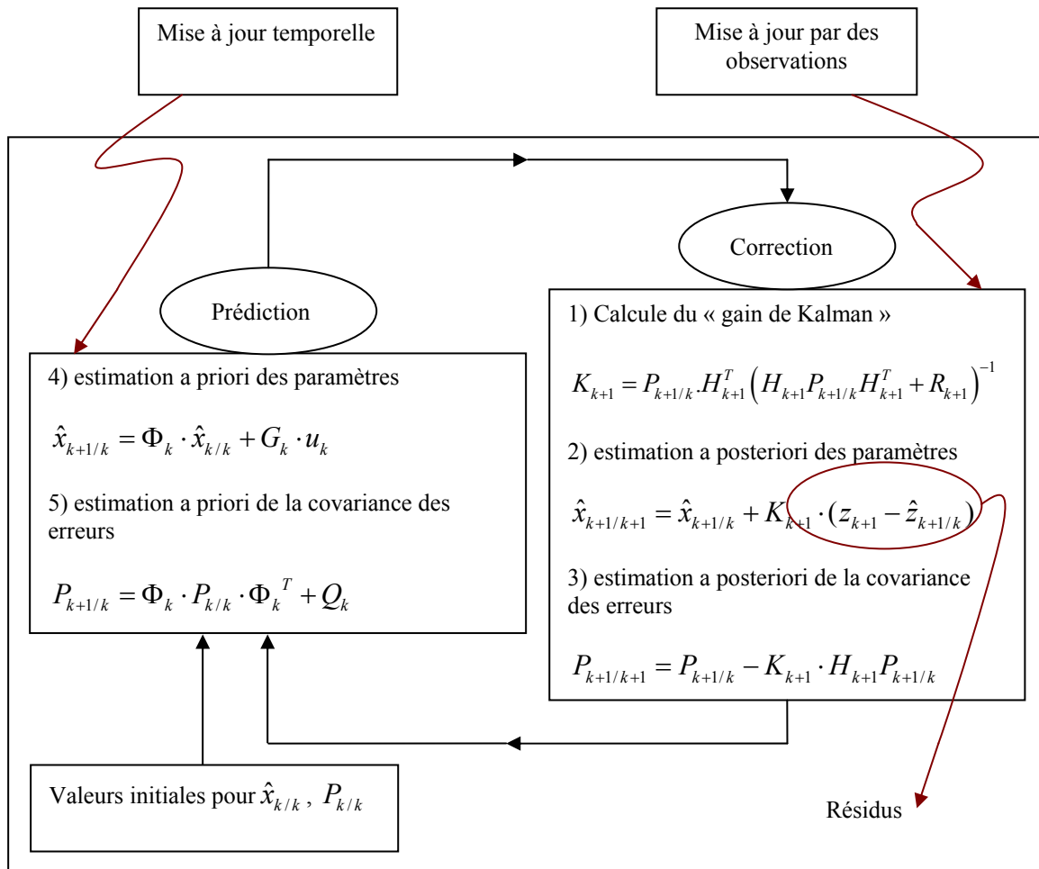
Figure 19: Le filtre de Kalman
