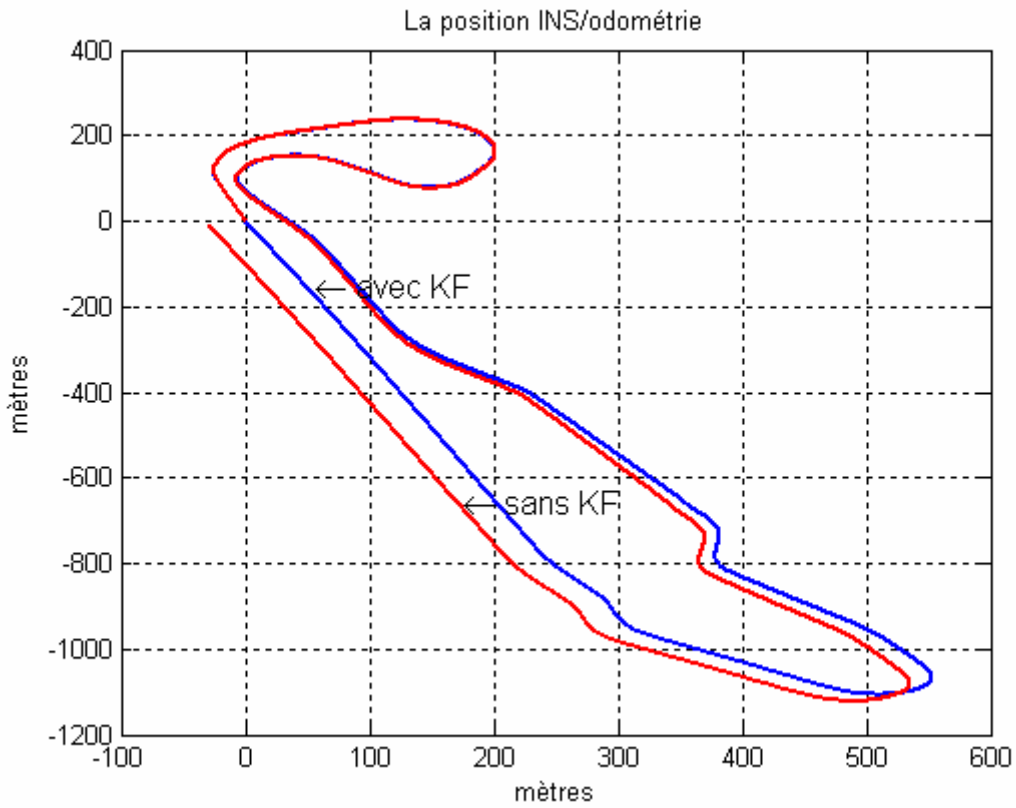
Figure 74: Intégration INS/odométrie
