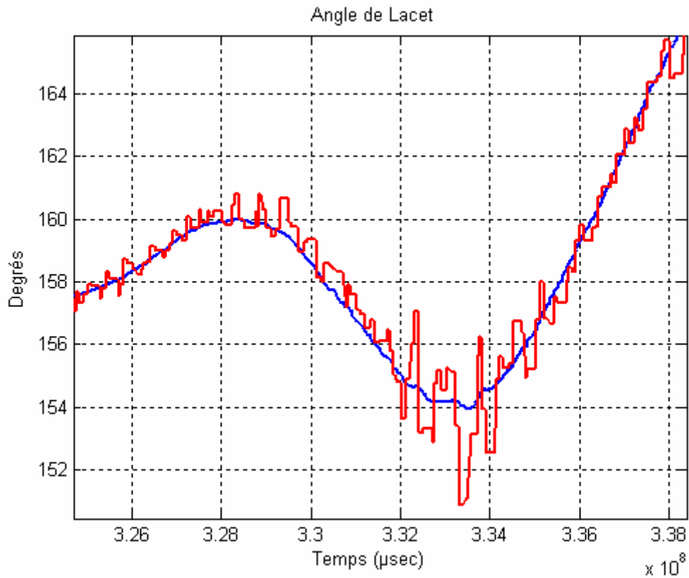
Figure 79: Zoom sur les résultats de l'angle de cap à partir du GPS simple et du couplage INS/GPS
