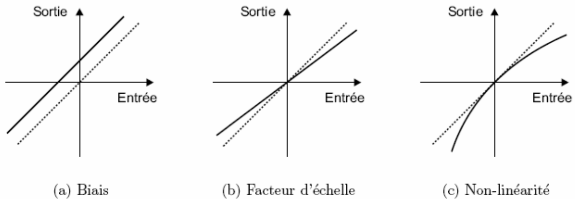
Figure 14: Types d'erreurs de mesure classiques
