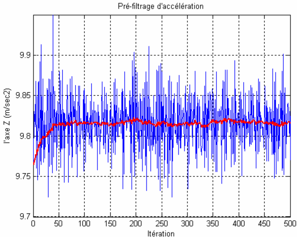
Figure 49: L'accélération brute et pré-filtrée sur l'axe z (zoom)
