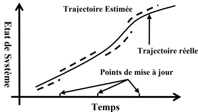
Figure 22: Trajectoire estimée (nominale) et réelle pour un filtre de Kalman étendu
