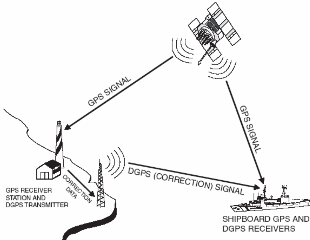
Figure 4: La correction différentielle
