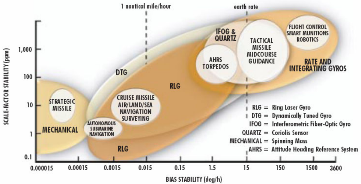
Figure 12: Applications courantes de la technologie gyroskopique
