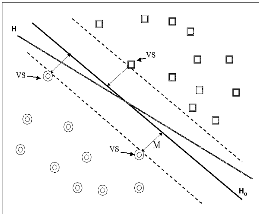
FIG. 2.3 – Hyperplans séparateurs : H est un hyperplan quelconque, H_o est l'hyperplan optimal et M est la marge qui représente la distance entre les différentes classes et H_o (VS sont les Vecteurs Supports).
