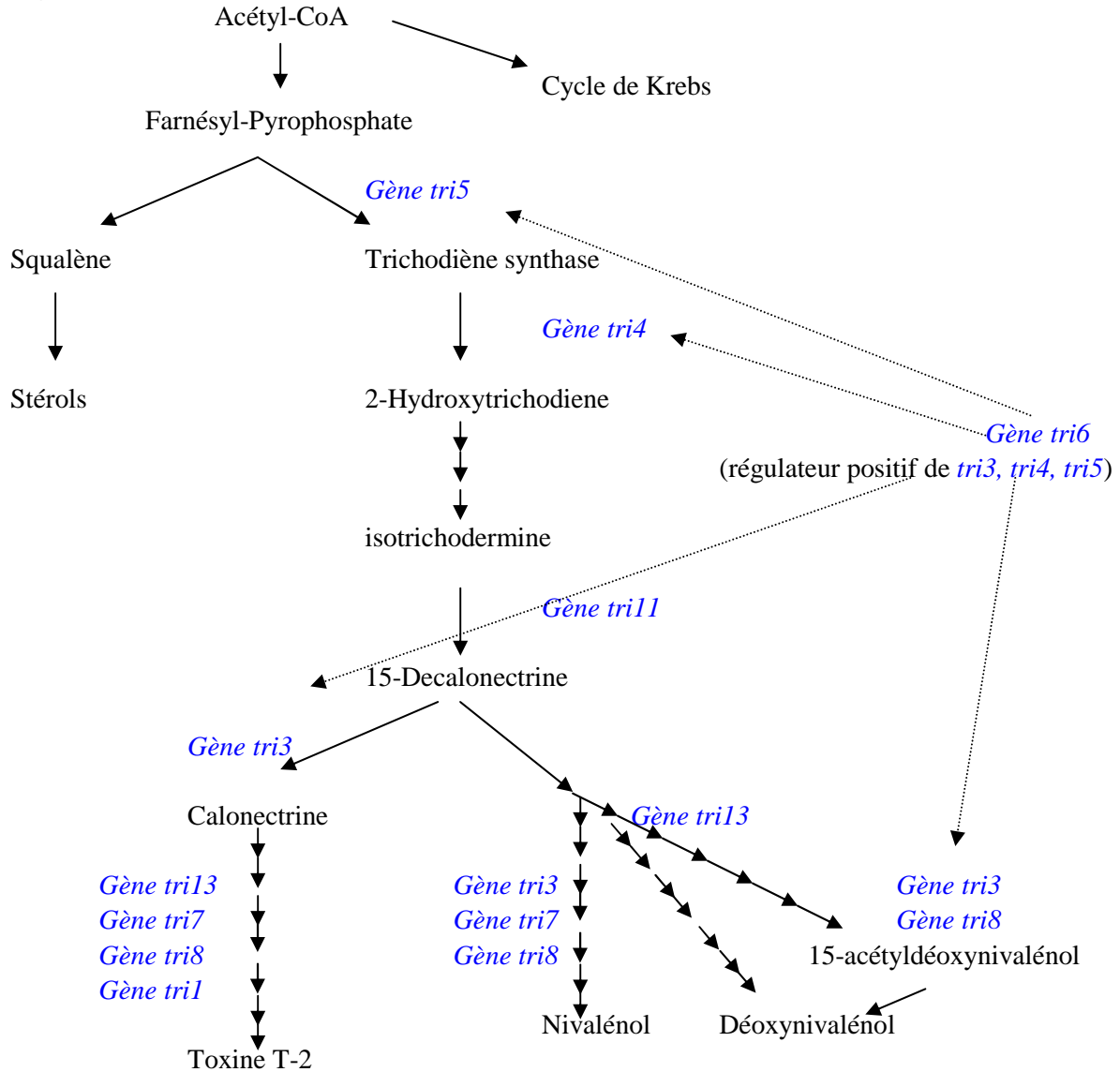
Figure 2-5 : Voie de biosynthèse des trichothécènes
