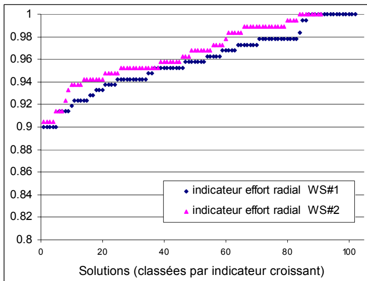
Figure 71: Valeurs croissantes de l'indicateur de performance "effort radial", pour chaque concept.
