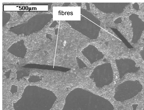
Figure 41. Fibres polypropylène dispersés dans un BHP. Image MEB 50x, échantillon poli.
