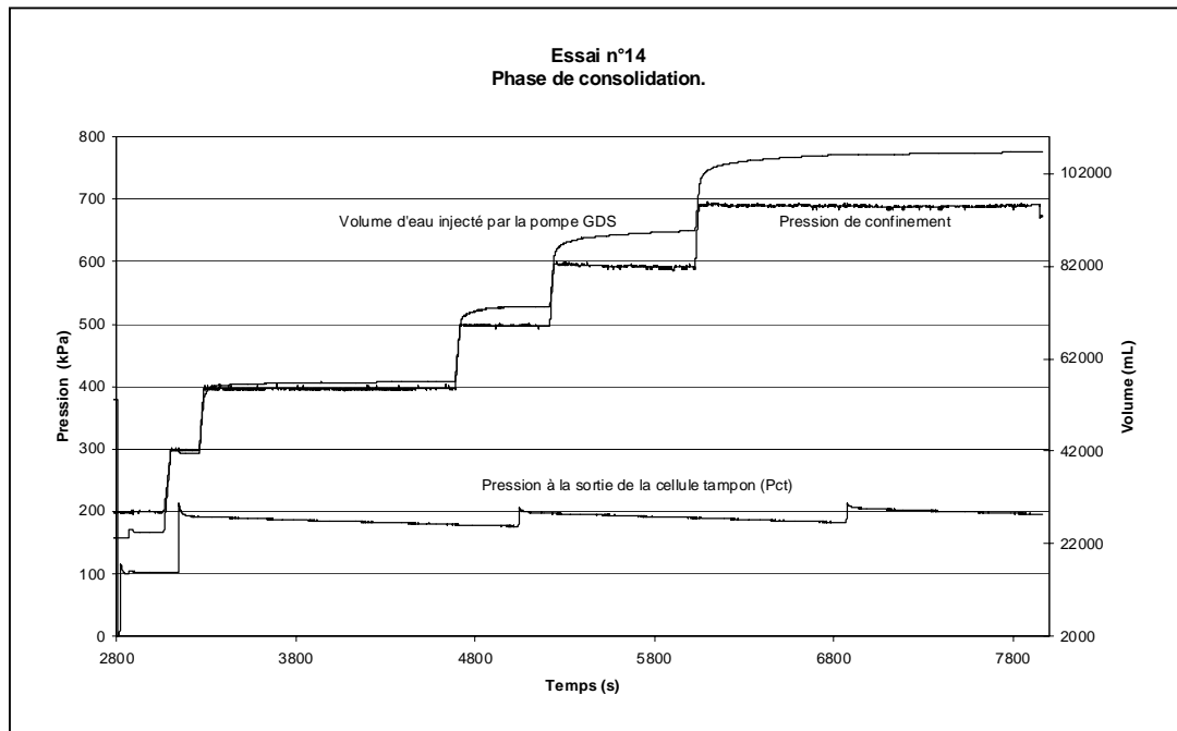
Fig. A4-1 : Phase de consolidation de l'échantillon. Essai
