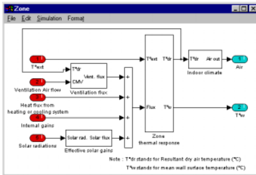
Figure 3.22 : Le niveau fonctionnel du modèle bâtiment
