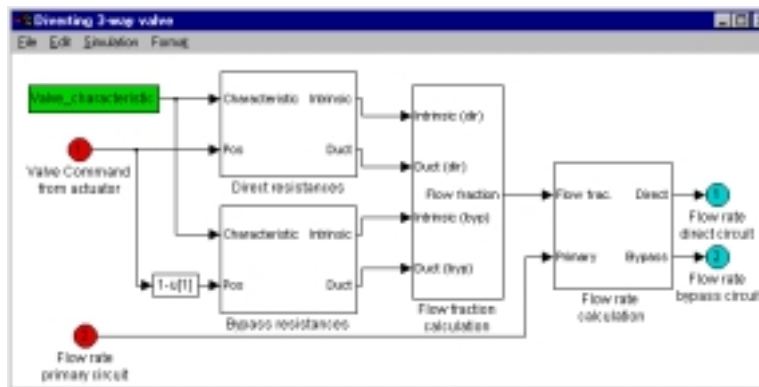
Figure 3.12 : Le niveau fonctionnel d'une vanne trois voies montée en diviseuse.
