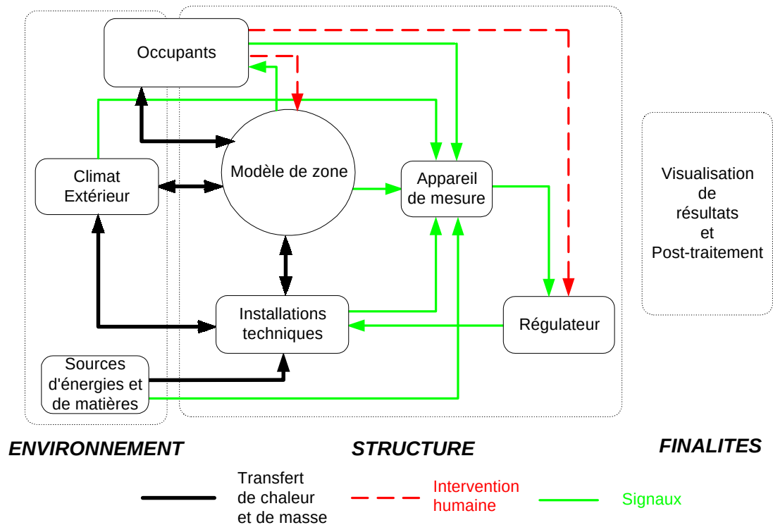
Figure 2.4 : Le schéma graphique générique du modèle bâtiment
