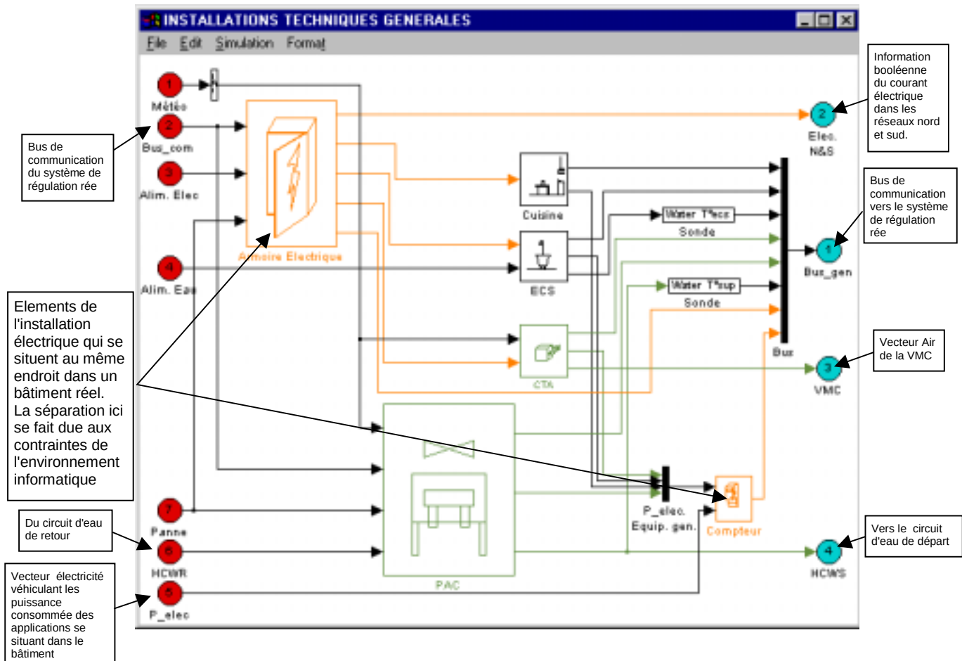
Figure 4.3 : Les équipements généraux à partir du niveau général
