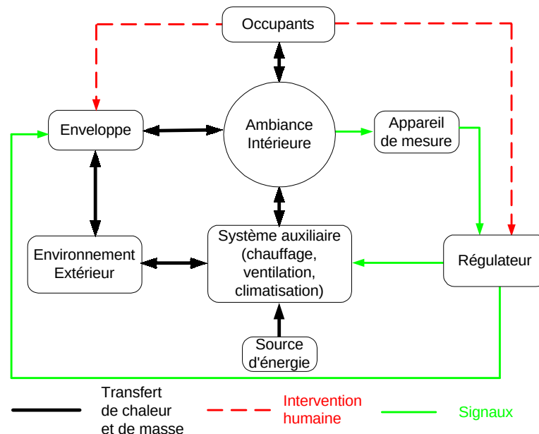
Figure 2.3 : Schéma générique du bâtiment selon [Hensen 91]
