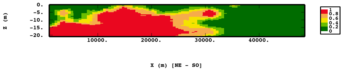
(a) Proportion moyenne sur toutes les simulations
