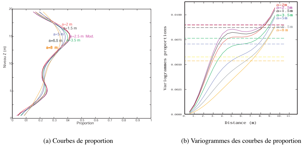
FIG. 6.8 – Courbes et variogrammes des proportions obtenues avec différents couples intensité - objet. La proportion initiale de référence correspond à a = 2.5\text{ m} .
