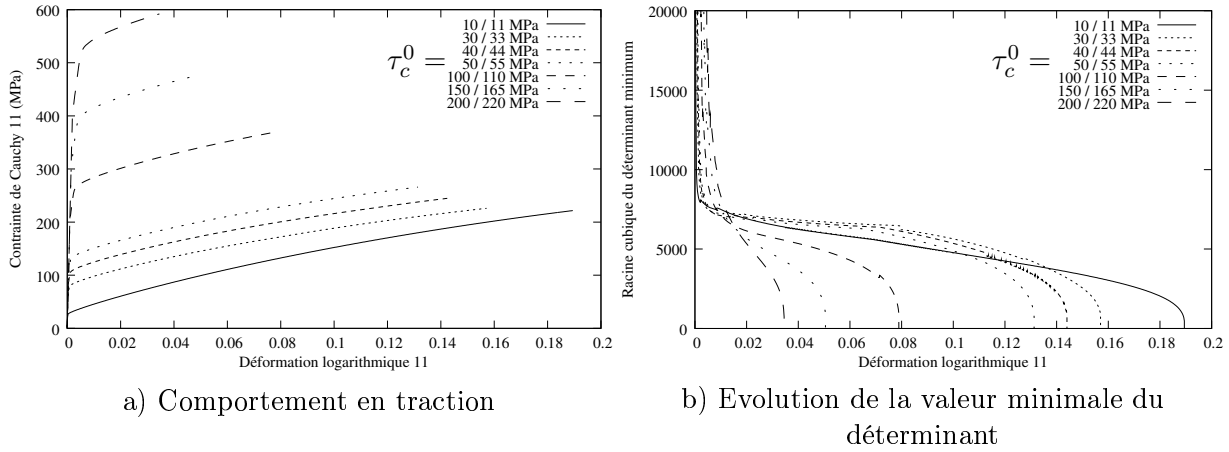
FIG. 3.13 – Influence de la cisson critique initiale \tau_c^0
