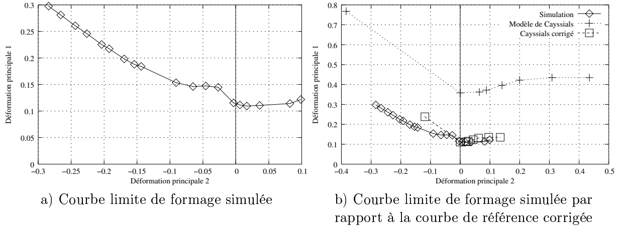
FIG. 3.26 – Courbes limite de formage simulée et corrigée d'après Cayssials [Cay00] de l'acier C1754
