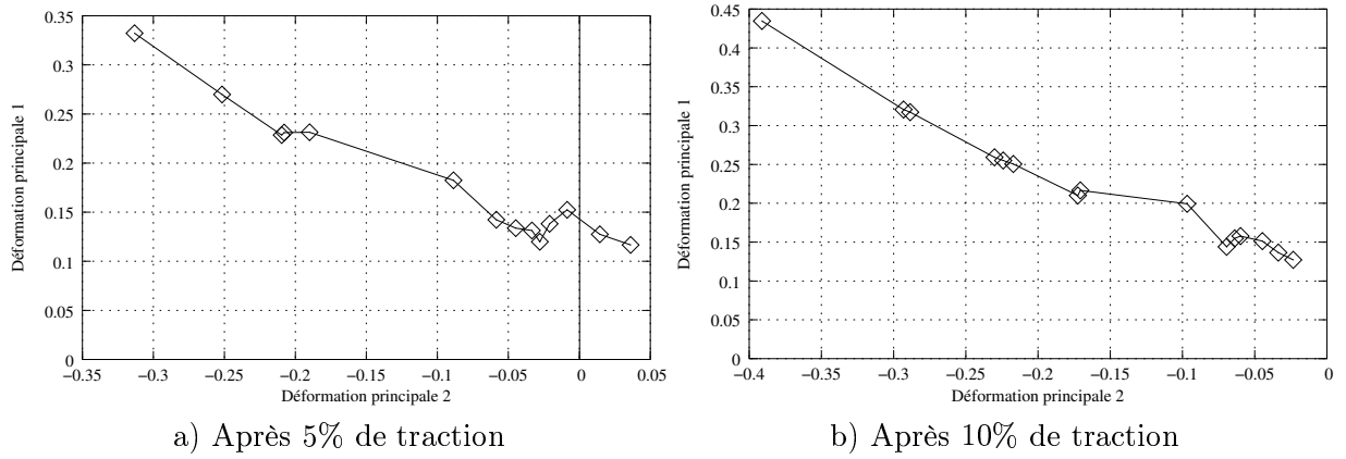
FIG. 3.27 – Courbes limite de formage simulées après une prédéformation en traction uniaxiale de l'acier C1754
