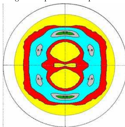
Figure de pôles 200 expérimentale
