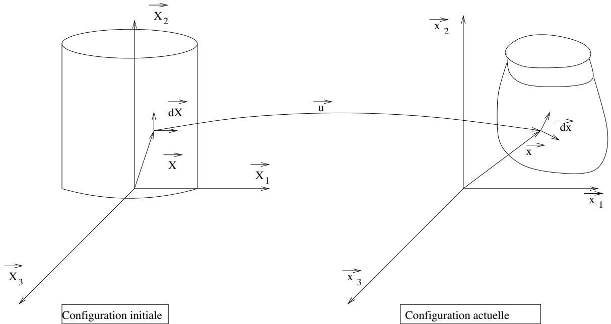
FIG. A.1 – Déformation d'un solide
