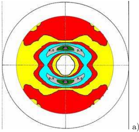
Figure de pôles 110 expérimentale
