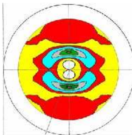
Figure de pôles 110 expérimentale
