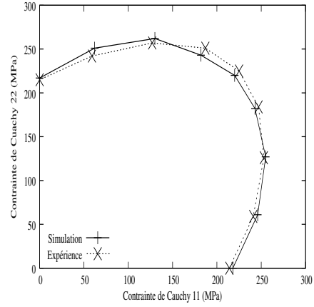
d) 1% de déformation plastique en TU
