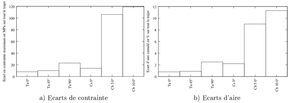
FIG. 2.35 – Ecart en aire et en contrainte pour l'acier A159
