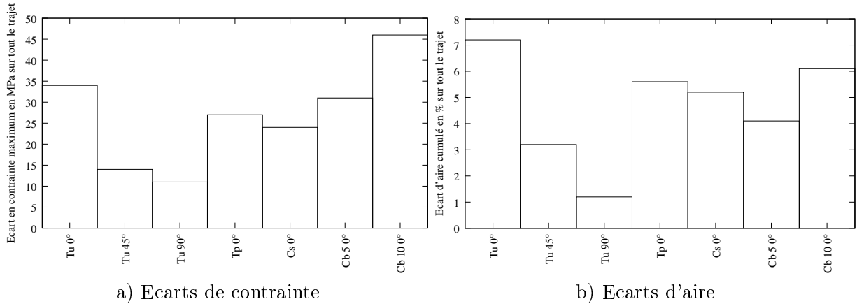
FIG. 2.20 – Ecart en aire et en contrainte pour l'acier S2325
