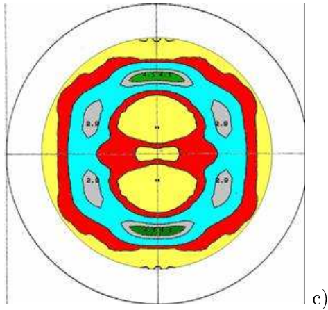
Figure de pôles 200 expérimentale
