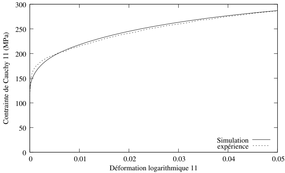
FIG. 2.21 – Identification paramétrique pour l'acier DDQ
