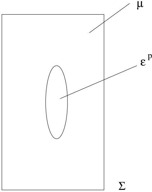
FIG. 2.1 – Modélisation d'Eshelby
