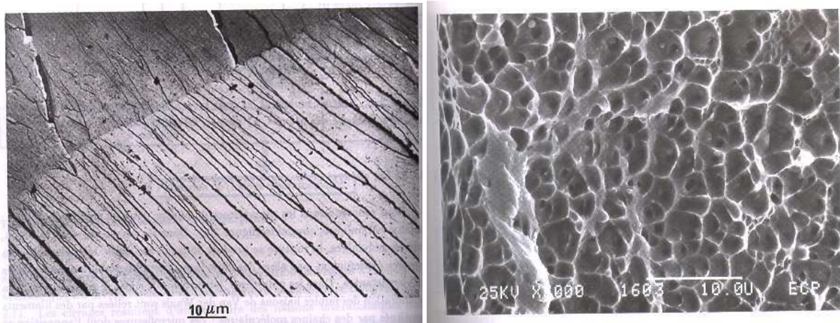
a) Rivières de clivage [FPZ95b]
