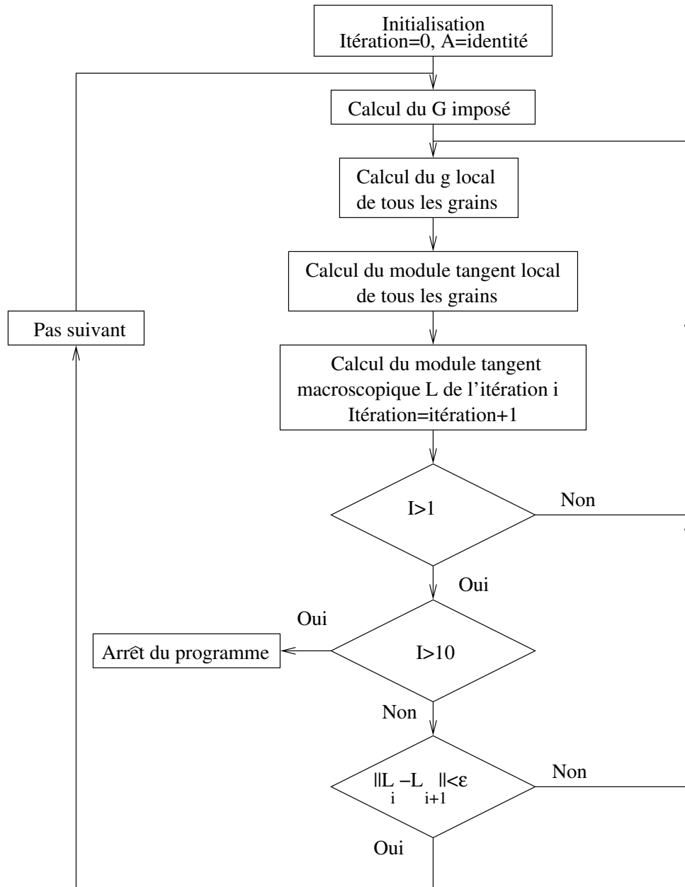
FIG. 2.5 – Algorithme de résolution du schéma autocohérent
