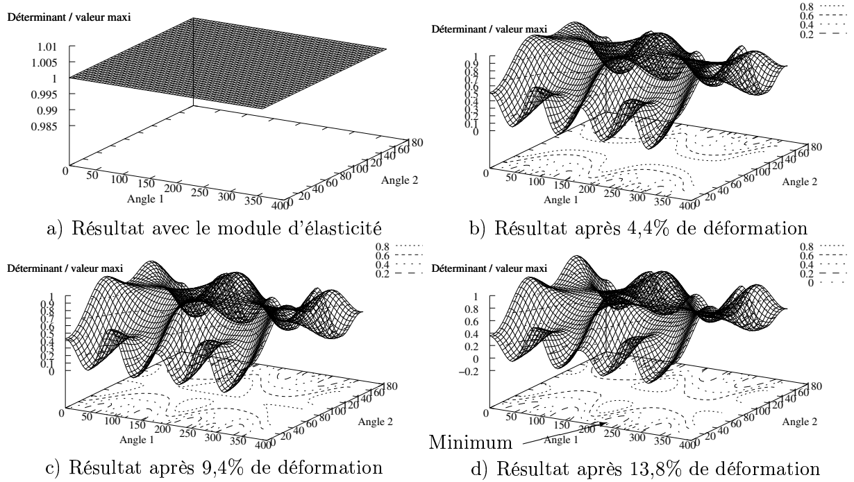
FIG. 3.18 – Evolution du déterminant normalisé au cours de la déformation en fonction de l'orientation de la normale lors d'un essai de traction uniaxiale pour un polycristal de 100 grains
