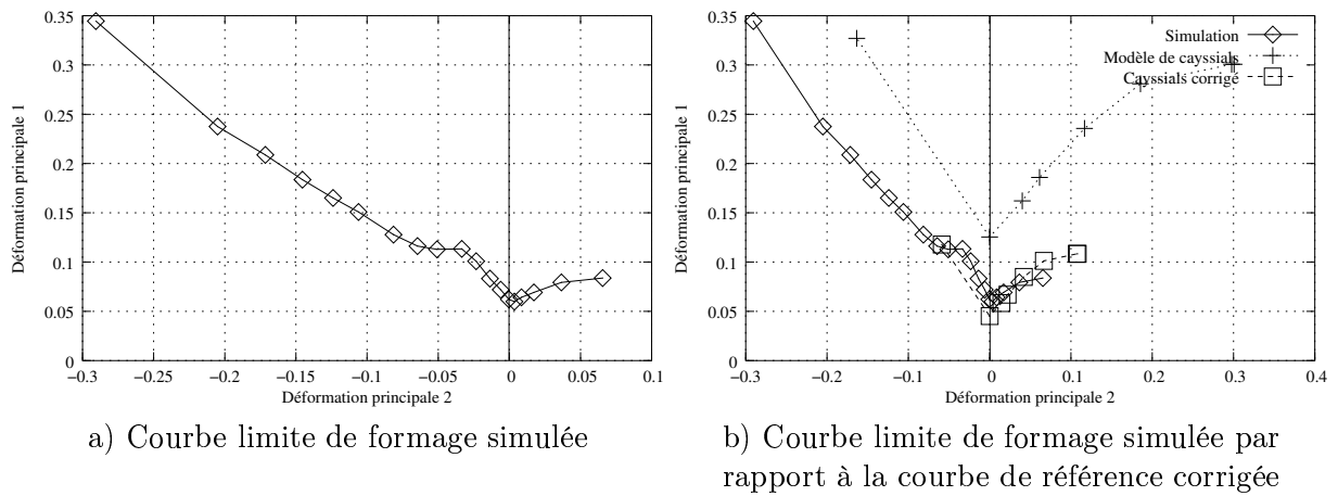
FIG. 3.30 – Courbes limite de formage simulée et corrigée d'après Cayssiàls [Cay00] de l'acier D1957
