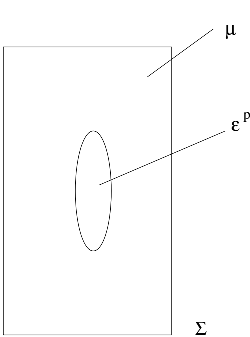
FIG. 2.1 – Modélisation d'Eshelby
