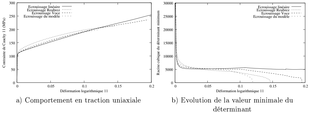
FIG. 3.16 – Influence de la matrice d'écroissage sur le comportement du monocristal
