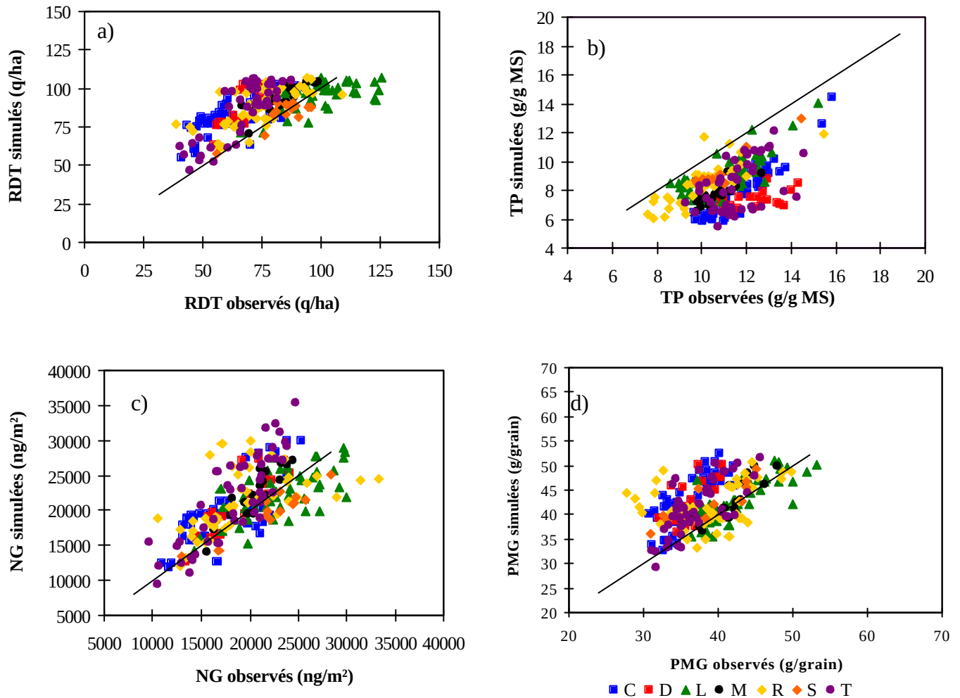
Figure 38 : Comparaison des valeurs observées et simulées pour le rendement (a), la teneur en protéines (b), le nombre de grains par m² et le poids de mille grains (d), en fonction de la station d'essai. (C=Clermont-Ferrand, D=Dijon, L= Le Moulon, M = Mons, R = Rennes, S = Serasem, T = Toulouse).
