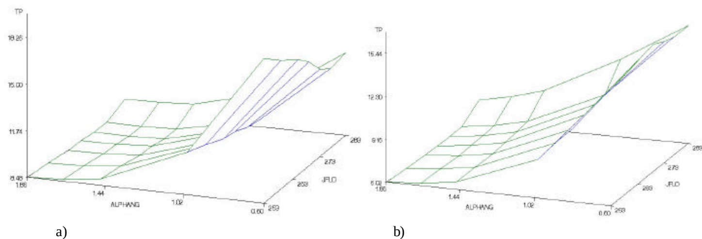
Figure 35 : Variation de la teneur en protéines en fonction des facteurs Alphaning et J_{FLO} pour les environnements LMNR (a) et SRNR (b).
