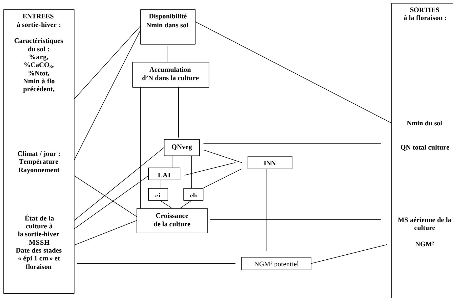
Figure 8 : Représentation schématique du fonctionnement d'Azodyn pour la période sortie-hiver à floraison.
