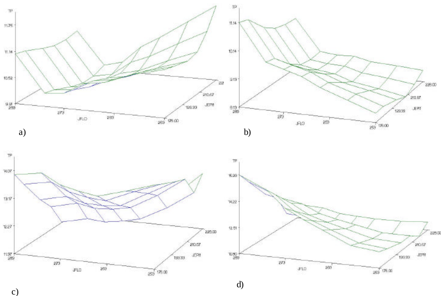
Figure 36 : Variation de la teneur en protéines en fonction des facteurs JFLO et JE1C sur les environnements CLIN (a), CLNR (b), SRIN (c) et SRNR (d).
