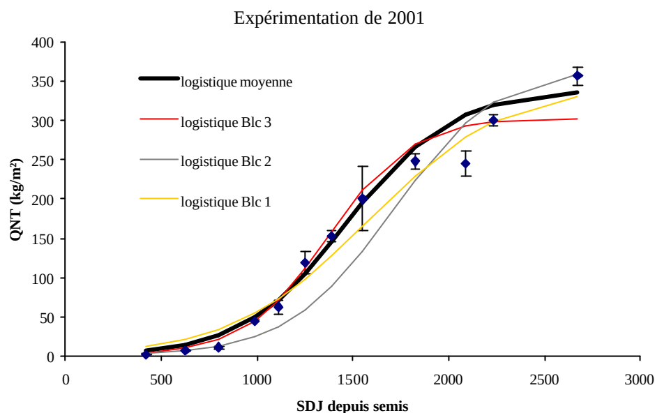
Figure 19 : Ajustement de la courbe logistique aux données expérimentales pour chacune des répétitions et en moyenne pour le géotype Arche expérimenté en 2001, valeurs moyennes et écart-types pour chaque date de prélèvement.
