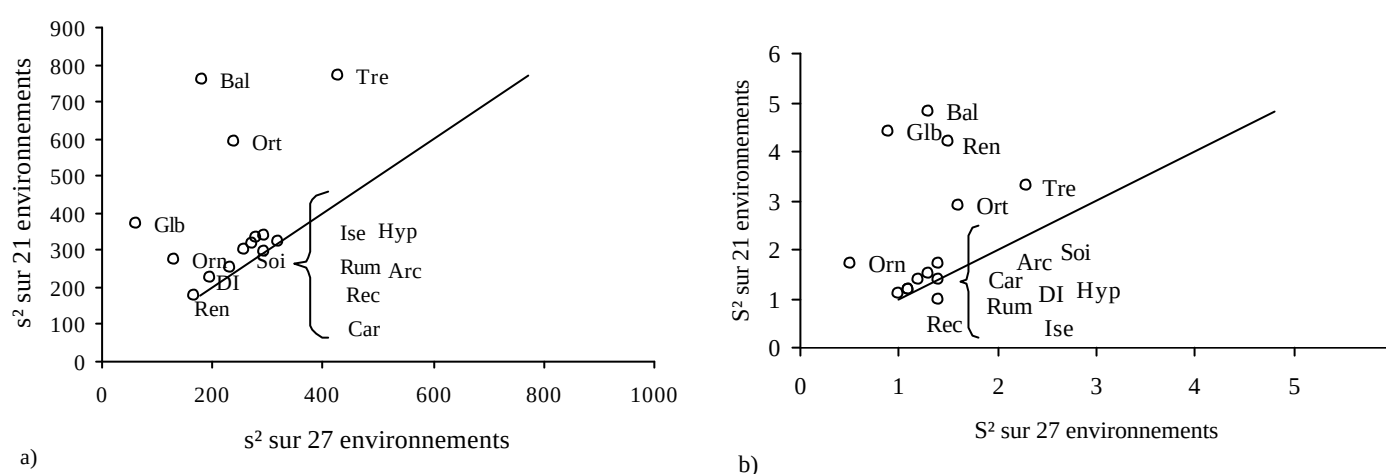
Figure 18 : Comparaison des variances environnementales estimées sur l'ensemble des 27 environnements du réseau d'essais ou pour le sous-ensemble de 21 environnements pour le rendement (a) et la teneur en protéines des grains (b)
