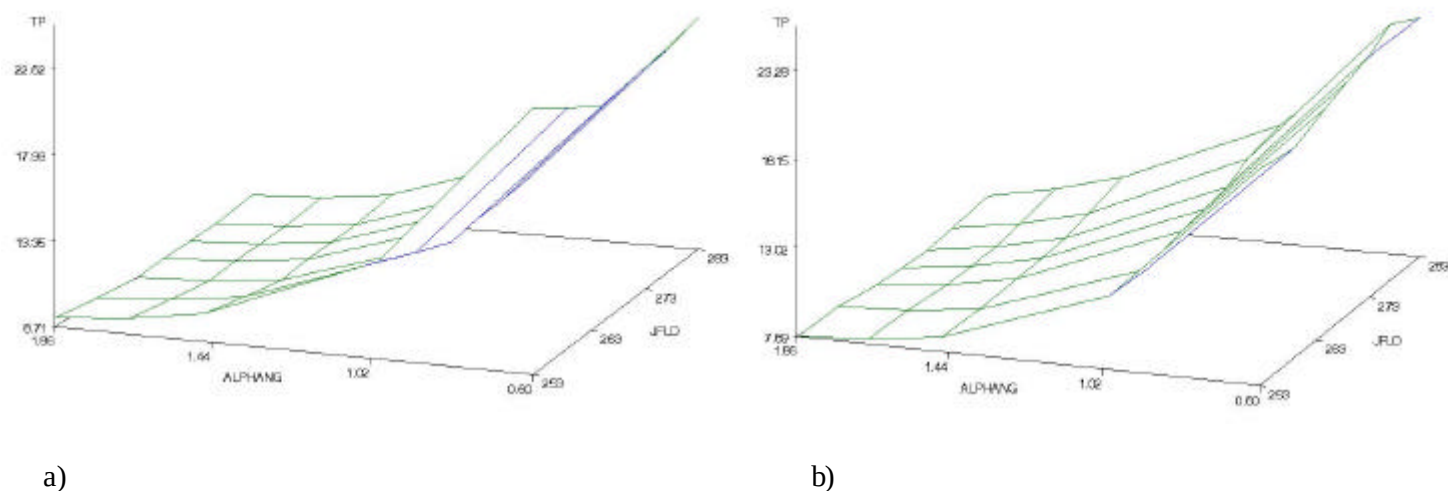
Figure 34 : Variation de la teneur en protéines en fonction des facteurs Alphaning et J_{FLO} pour les environnements CLIN (a) et CLNR (b).
