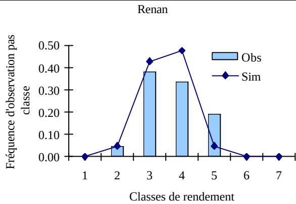
Figure 43 : Distribution des rendements observés et simulés pour les génotypes Renans, Rumba, Soissons, Baltimor, Galibier, Ornicar et Trémie sur l'ensemble des environnements considérés.
