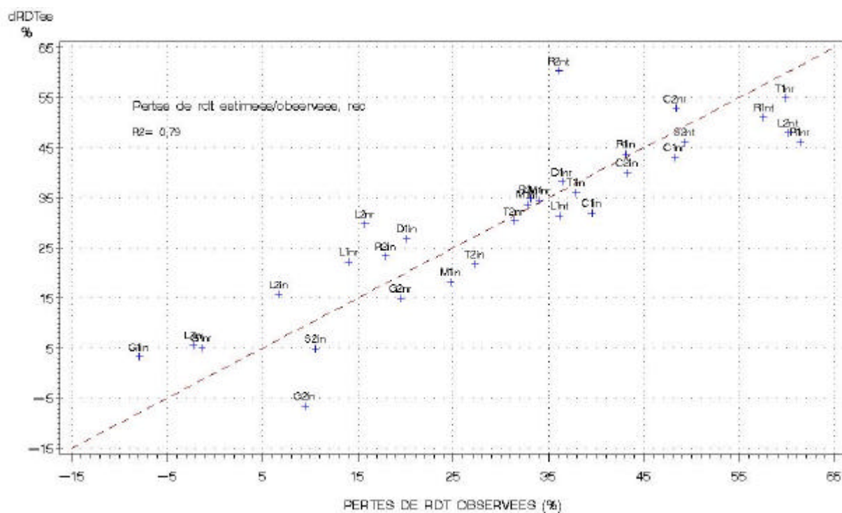
Figure 16 : Comparaison des pertes de rendement observées et estimées (dRDTes) à partir de la régression multiple effectuée sur l'ensemble des environnements (31) pour la variété Récital.
