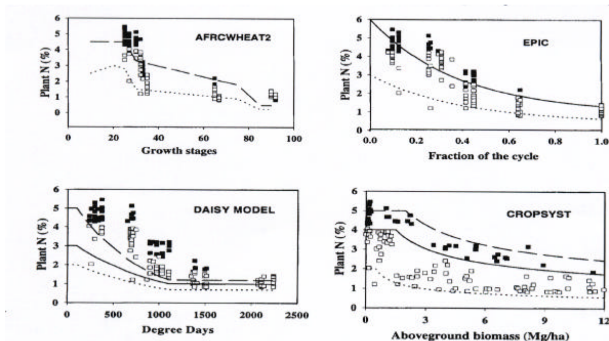
Figure 5 : Comparaison de quatre modèles et de leurs courbes d'évolution de la teneur en azote en fonction des différentes variables qui permettent de les estimer. Les différents modèles sont comparés avec des données expérimentales issues d'essais limitants (carrés vides) et non limitants en azote (carrés pleins). D'après Stöckle et Debaeke (1997).
