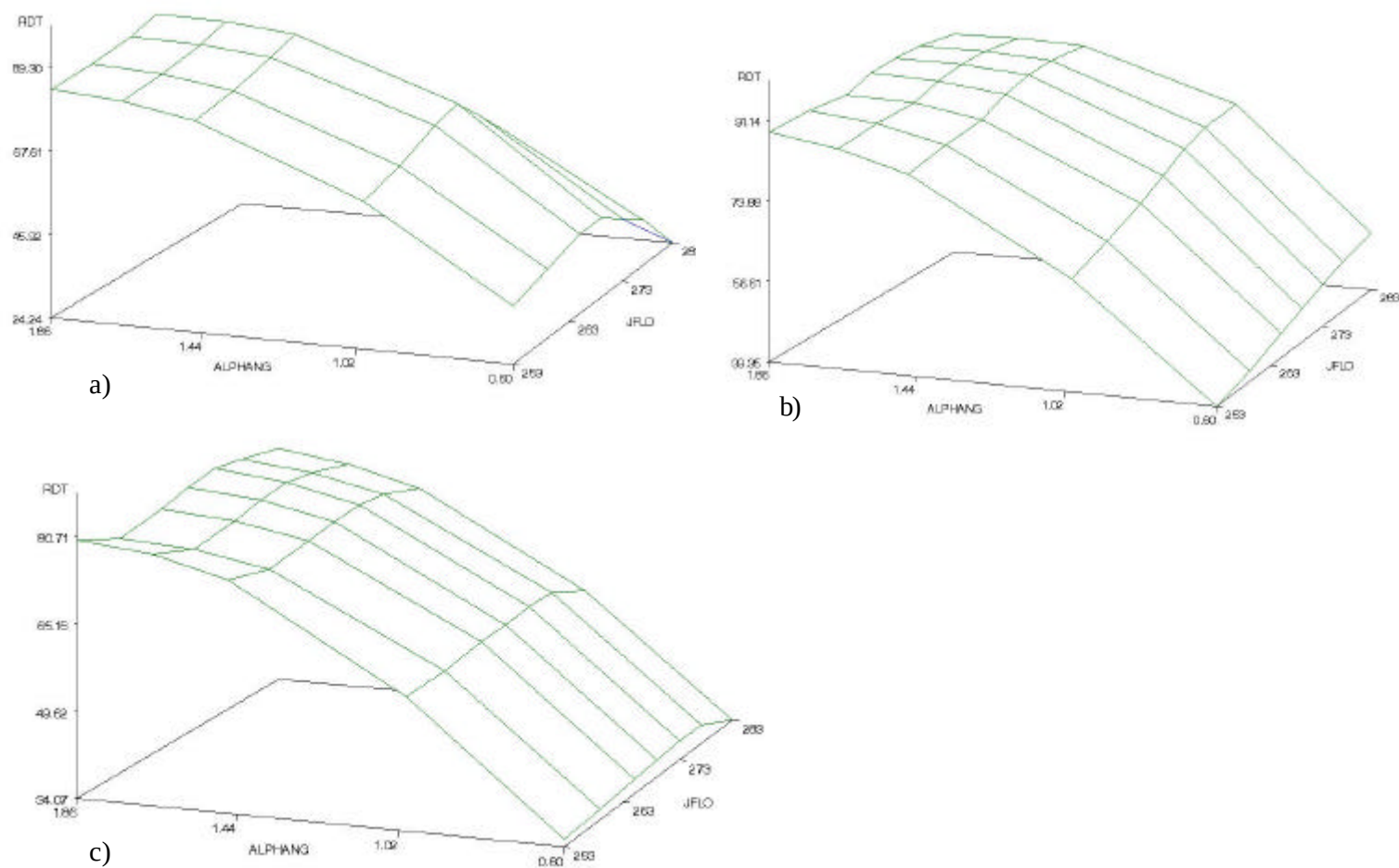
Figure 28 : Influence des facteurs Alphan et J_{FLO} sur le rendement pour les environnements CLIN (a), LMIN (b) et SRIN (c).
