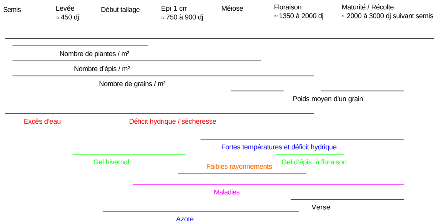
Figure 13 : Cycle schématique de l'élaboration du rendement chez le blé tendre et éléments de croissance et de développement nécessaires par phase d'après Meynard (1987) et Lecomte (com. Pers.).
