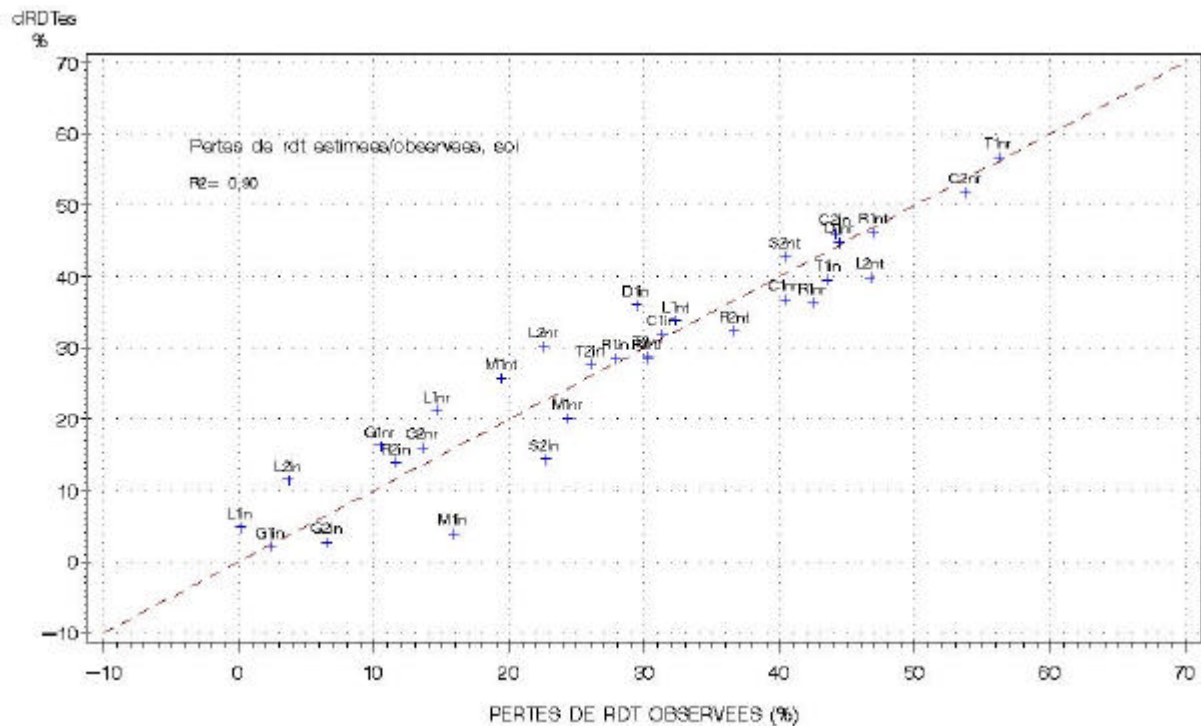
Figure 14 : Comparaison des pertes de rendement observées et estimées (dRDTe) à partir de la régression multiple effectuée sur l'ensemble des environnements (31) pour la variété Soissons
