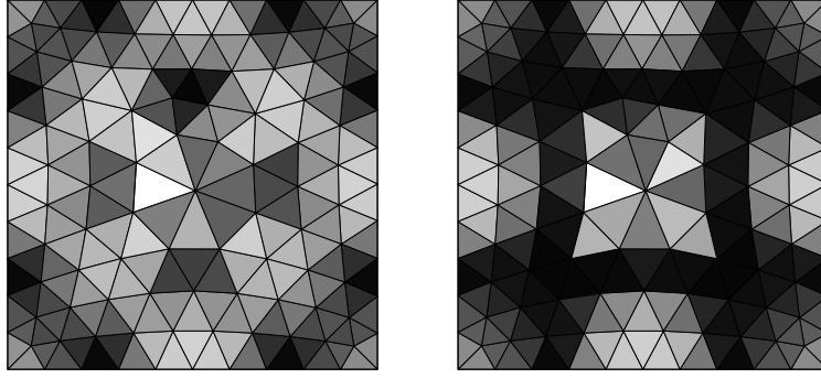
FIG. 2.7: Localisation de l'erreur réelle (gauche) et de l'estimateur d'erreur par résidu \eta_1(u_h) (droite) pour la triangulation quasi-uniforme de taille h = \frac{h_0}{2}
