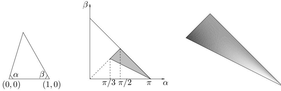
FIG. 2.4: Gauche : triangle T d'angles \alpha et \beta ; centre : domaine D (triangle ombré) pour les couples (\alpha, \beta) ; droite : fonction (\alpha, \beta) \in D \mapsto \gamma_T (dans la table des couleurs, les valeurs noires correspondent à 0.4 et les valeurs blanches à 0.75)
