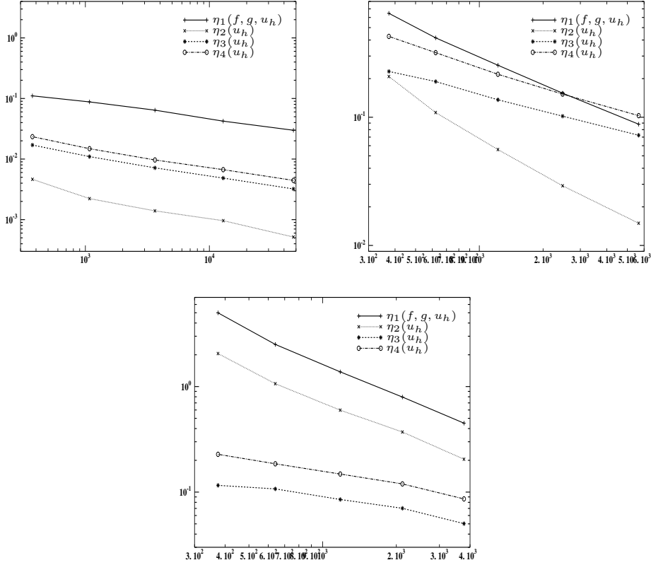
FIG. 4.6: Estimateurs d'erreur a posteriori par résidu sur les triangulations générées de façon adaptative avec \eta_{1,T}(f, g, u_h) en fonction du nombre d'arêtes. En haut à gauche : \epsilon = 1 ; en haut à droite : \epsilon = 10^{-2} ; en bas : \epsilon = 10^{-4}
