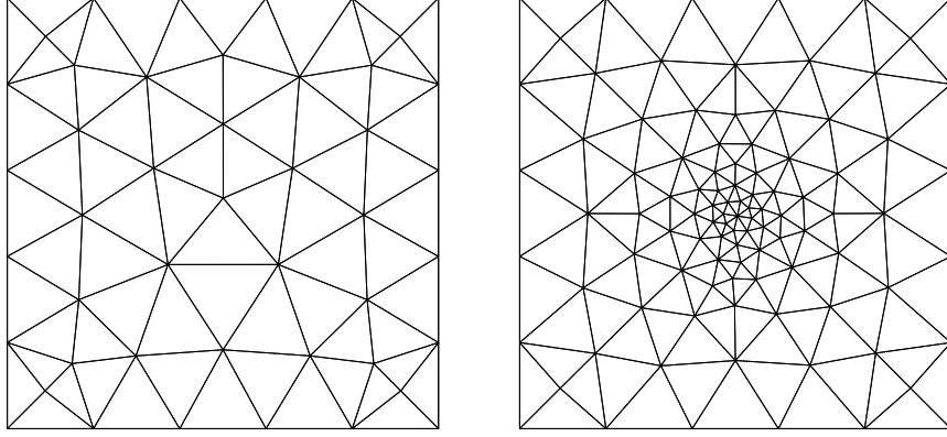
FIG. 2.5: A gauche : triangulation quasi-uniforme de taille h_0 ; à droite : triangulation non-uniforme de taille h_0
