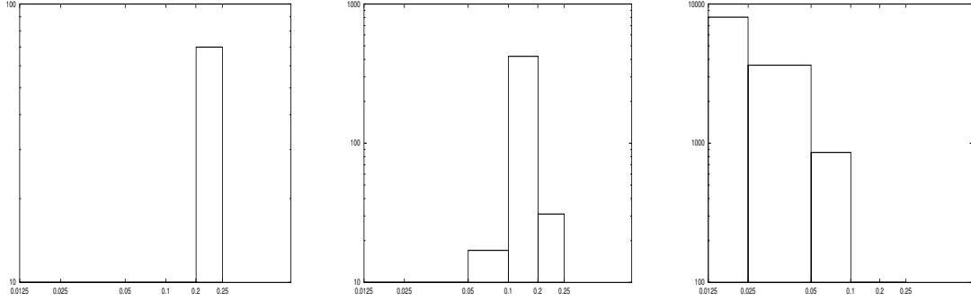
FIG. 2.12: Répartition des triangles par leur taille sur des triangulations générées de façon adaptative en utilisant \eta_{1,T}(u_h) comme indicateur d'erreur. A gauche : sur la triangulation initiale ; au centre : sur la triangulation générée de façon adaptative après 3 itérations ; à droite : sur la triangulation générée de façon adaptative après 6 itérations
