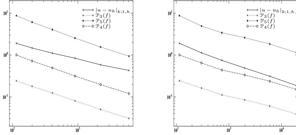
FIG. 2.16: Erreur réelle et estimateurs d'erreur par résidu en fonction de nombre de faces du maillage sur les triangulations raffinées de façon adaptative en utilisant \mathcal{P}_{3,T}(f) (à gauche) ; \eta_{1,T}(u_h) (à droite)
