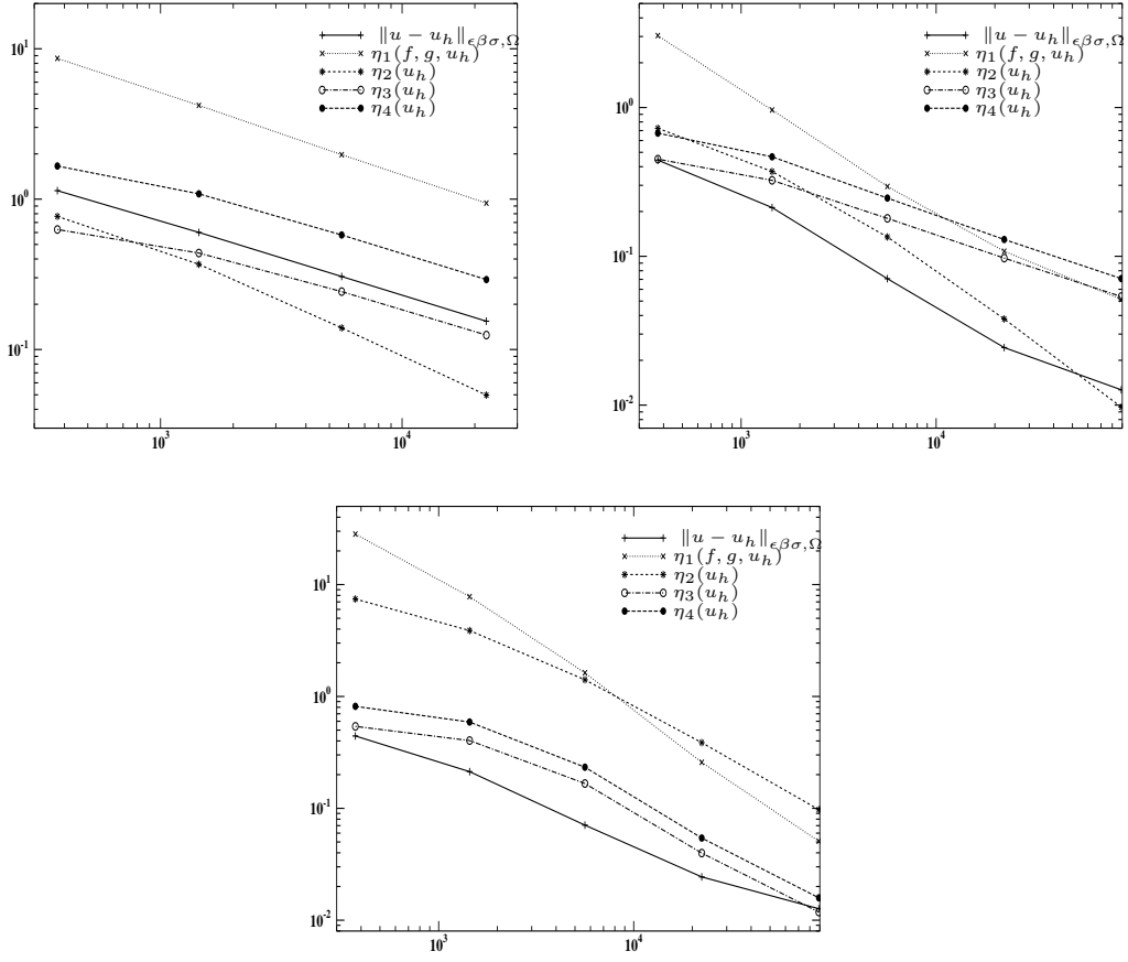
FIG. 4.1: Erreur réelle et estimateurs d'erreur a posteriori en fonction du nombre de faces de la triangulation. Gauche : \epsilon = 1 ; centre : \epsilon = 10^{-2} ; droite : \epsilon = 10^{-4}
