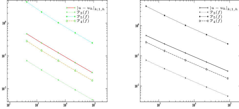
FIG. 2.11: Erreur exacte et estimateurs d'erreur hiérarchiques en fonction du nombre de faces du maillage. Gauche : \varrho_\Omega(k) = 10^3 ; droite : \varrho_\Omega(k) = 10^6
