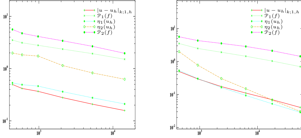
FIG. 2.18: Erreur exacte et estimateurs d'erreur par résidu en fonction de nombre de faces du maillage lorsque \varrho_\Omega(k) = 10^3 sur les triangulations raffinées de façon adaptative en utilisant \mathcal{P}_{3,T}(f) (à gauche) ou \eta_{1,T}(u_h) (à droite)
