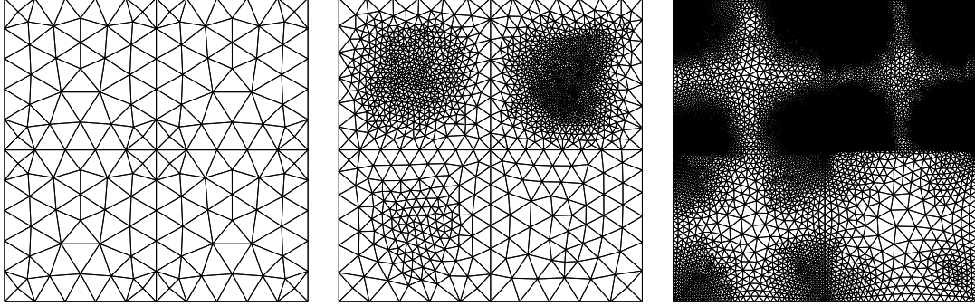
FIG. 2.17: Gauche : triangulation initiale (440 faces) ; centre : triangulation raffinée de façon adaptative en utilisant \mathcal{P}_{3,T}(f) (14395 faces) ; droite : triangulation raffinée de façon adaptative en utilisant \eta_{1,T}(u_h) (54738 faces)
