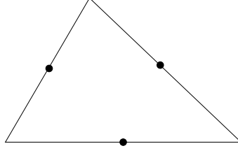
FIG. A.1: Degrés de liberté de l'élément fini de Crouzeix–Raviart
