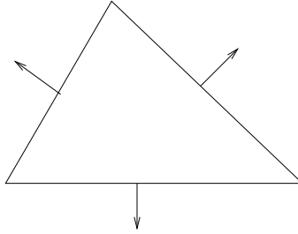
FIG. A.2: Degrés de liberté de l'élément fini de Raviart–Thomas
