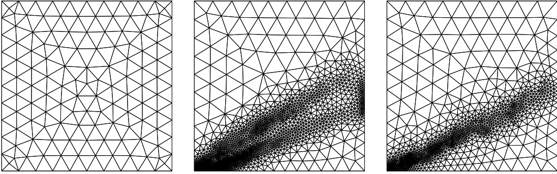
FIG. 4.5: Raffinement de maillage adaptatif en utilisant l’indicateur d’erreur \eta_{1,T}(f, g, u_h) . A gauche : maillage initial ; au centre : maillage adapté après 5 itérations pour \epsilon = 10^{-2} ; à droite : maillage adapté après 5 itérations pour \epsilon = 10^{-4}
