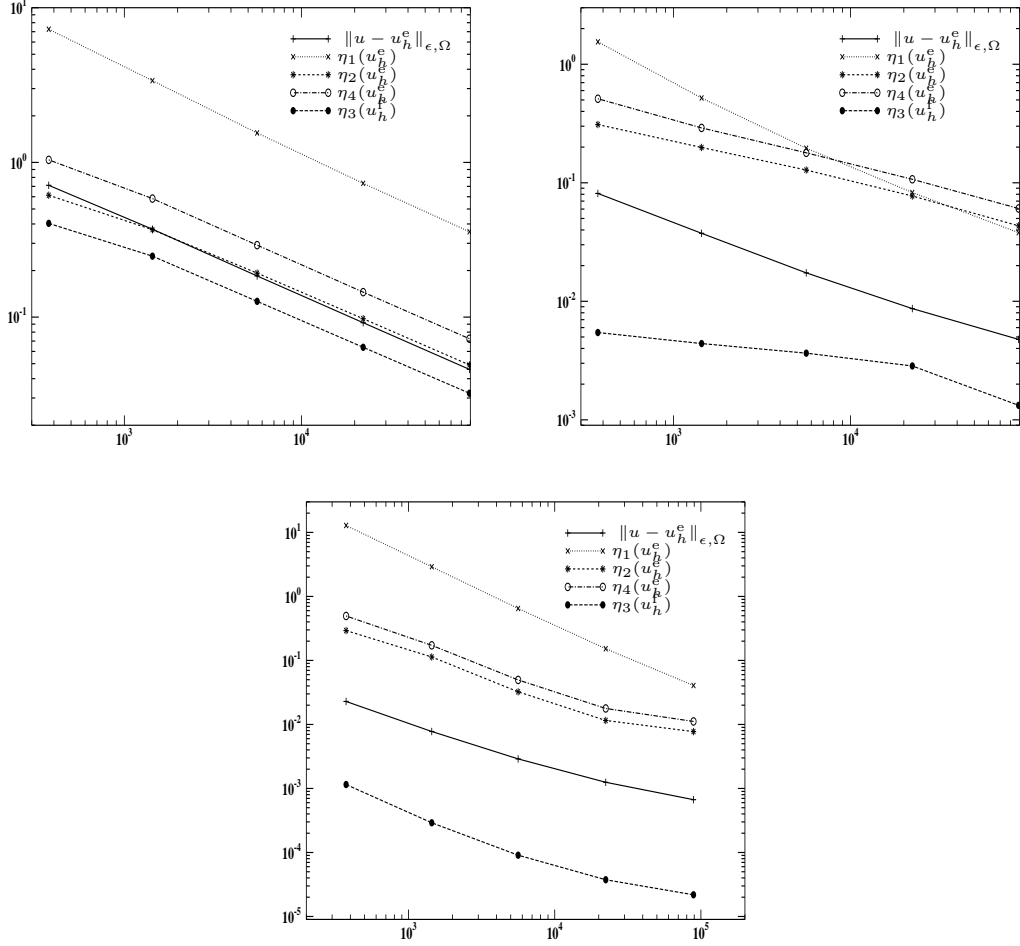
FIG. 3.2: Erreur réelle et estimateurs d'erreur a posteriori en fonction du nombre de faces de la triangulation. En haut à gauche : \epsilon = 1 , en haut à droite : \epsilon = 10^{-2} et en bas : \epsilon = 10^{-4}
