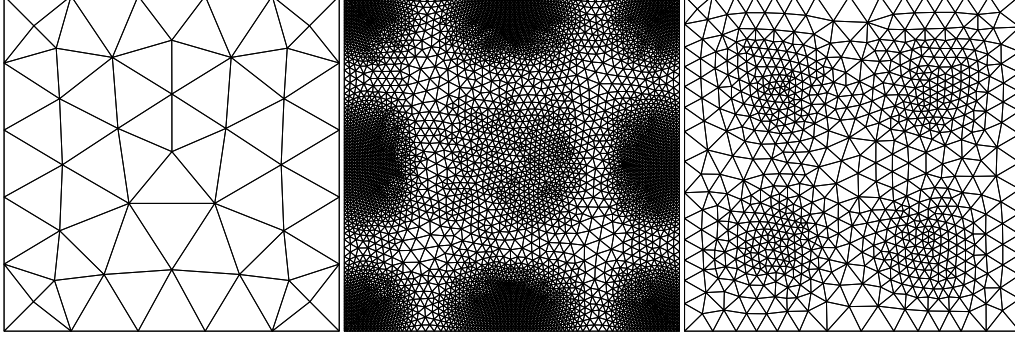
FIG. 2.14: A gauche : triangulation initiale de taille h_0 ; au centre : triangulation générée de façon adaptative après 6 itérations en utilisant \eta_{1,T}(u_h) comme indicateur d'erreur ; à droite : triangulation générée de façon adaptative après 6 itérations en utilisant \mathcal{P}_{3,T}(f) comme indicateur d'erreur
