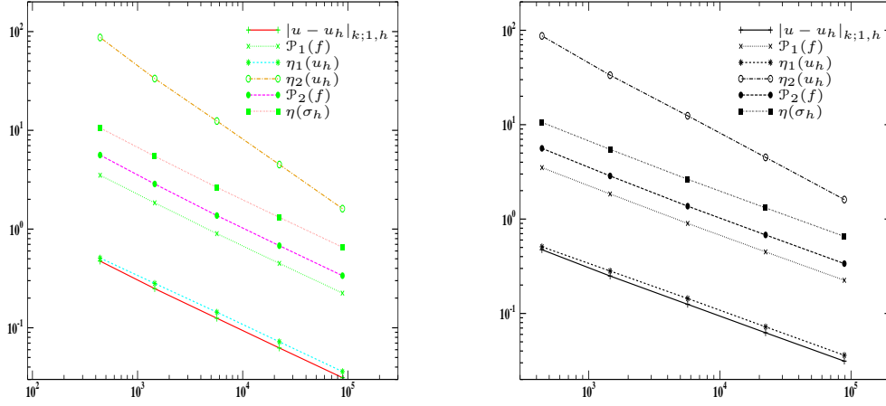
FIG. 2.9: Erreur exacte et estimateurs d'erreur par résidu en fonction de nombre de faces du maillage. Gauche : \varrho_{\Omega}(k) = 10^3 ; droite : \varrho_{\Omega}(k) = 10^6
