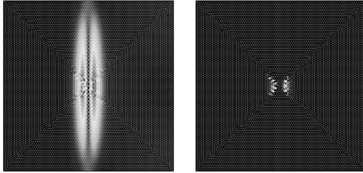
FIG. 3.4: Localisation de l'erreur réelle en norme \|\cdot\|_{\epsilon,\Omega} (à gauche) et de l'estimateur d'erreur a posteriori \eta_{1,T}(f, u_h^e) (à droite) lorsque \epsilon = 10^{-4} sur la triangulation de taille h_3
