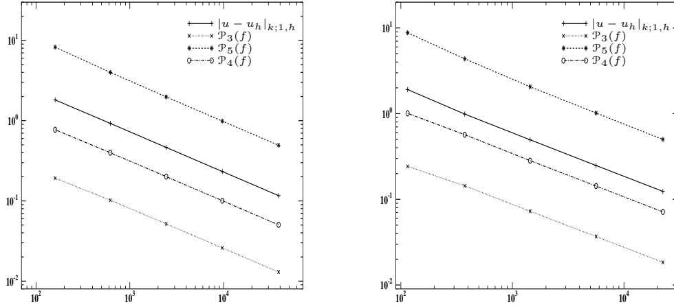
FIG. 2.8: Erreur réelle et estimateurs d'erreur hiérarchiques en fonction du nombre de faces de la triangulation. Gauche : triangulations quasi-uniformes ; droite : triangulations non-uniformes
