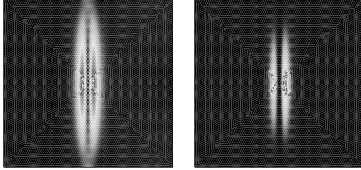
FIG. 3.3: Localisation de l'erreur réelle en norme \|\cdot\|_{\epsilon,\Omega} (à gauche) et de l'estimateur d'erreur a posteriori \eta_{1,T}(f, u_h^e) (à droite) lorsque \epsilon = 1 sur la triangulation de taille h_3
