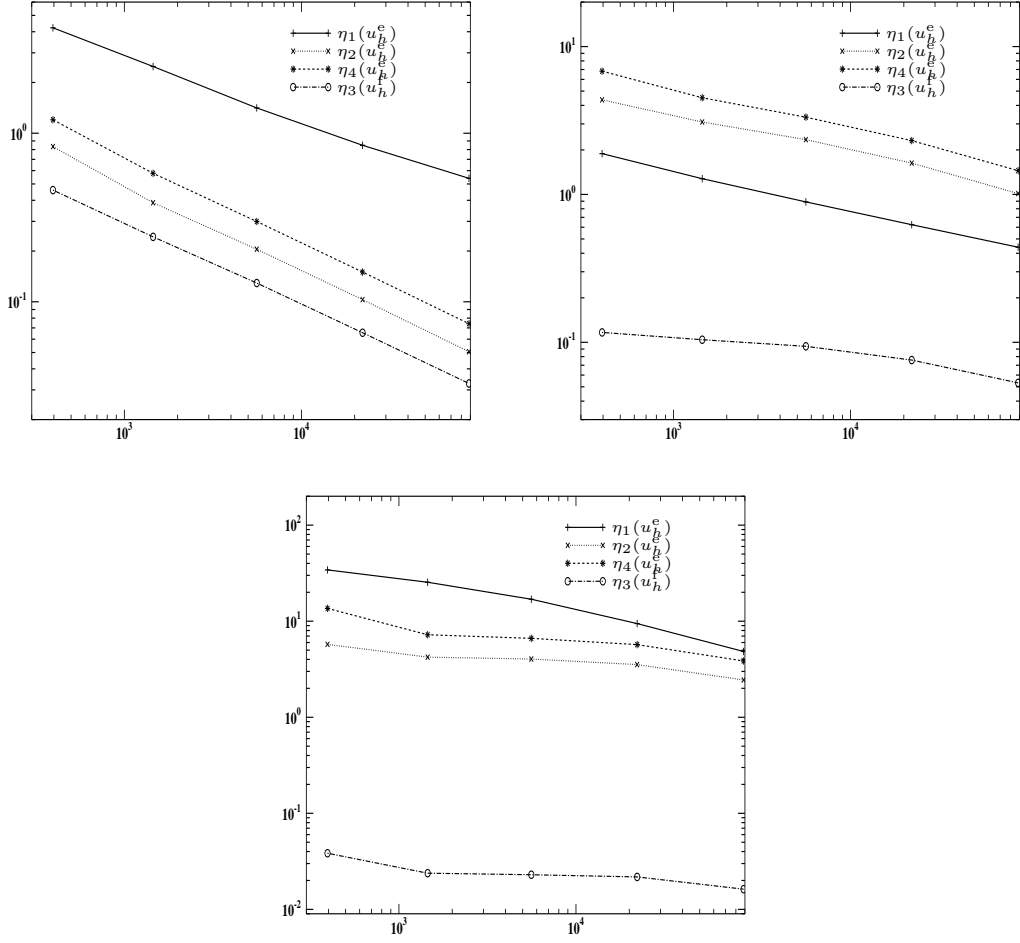
FIG. 3.9: Erreur réelle en norme \|\cdot\|_{\epsilon, \Omega} et estimateurs d'erreur a posteriori en fonction du nombre de faces de la triangulation générée de façon adaptative avec \eta_{1,T}(f, u_h^e) . En haut à gauche : \epsilon = 1 ; en haut à droite : \epsilon = 10^{-2} ; en bas : \epsilon = 10^{-4}
