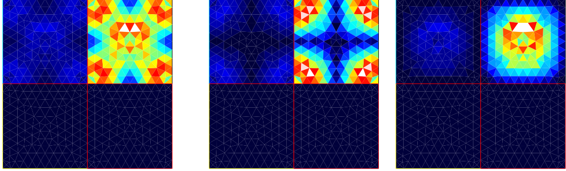
FIG. 2.10: Localisation de l'erreur réelle (gauche), localisation de l'estimateur d'erreur par résidu \eta_1(u_h) (centre) et localisation de l'estimateur d'erreur hiérarchique \mathcal{P}_3(f) (droite) pour une triangulation de taille h = \frac{h_0}{2} et \varrho_\Omega(k) = 10^6
