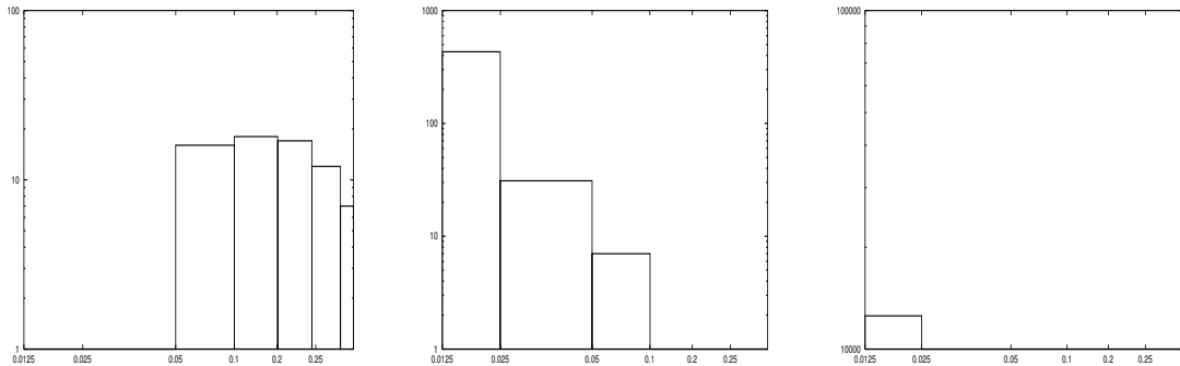
FIG. 2.13: Répartition des erreurs en pression sur des triangulations générées de façon adaptative en utilisant \eta_{1,T}(u_h) comme indicateur d'erreur. A gauche : sur la triangulation initiale ; au centre : sur la triangulation générée de façon adaptative après 3 itérations ; à droite : sur la triangulation générée de façon adaptative après 6 itérations
