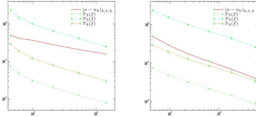
FIG. 2.19: Erreur exacte et estimateurs d'erreur par résidu en fonction du nombre de faces du maillage lorsque \varrho_\Omega(k) = 10^3 sur les triangulations raffinées de façon adaptative en utilisant \mathcal{P}_{3,T}(f) (à gauche) ou \eta_{1,T}(u_h) (à droite)
