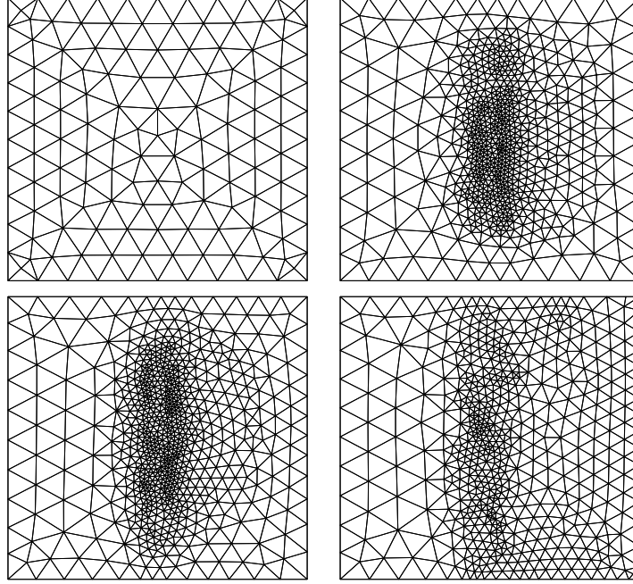
FIG. 3.5: Raffinement de maillage adaptatif en utilisant l'indicateur d'erreur \eta_{1,T}(f, u_h) . En haut à gauche : maillage initial (374 faces) ; en haut à droite : maillage adapté après 5 itérations pour \epsilon = 1 ; en bas à gauche : maillage adapté après 5 itérations pour \epsilon = 10^{-2} (2202 faces) ; en bas à droite : maillage adapté après 5 itérations pour \epsilon = 10^{-4} (1657 faces)
