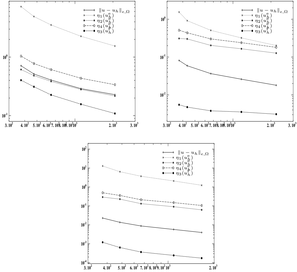
FIG. 3.6: Erreur réelle en norme \|\cdot\|_{\epsilon,\Omega} et estimateurs d'erreur a posteriori en fonction du nombre de faces de la triangulation générée de façon adaptative avec \eta_{1,T}(f, u_h^e) . En haut à gauche : \epsilon = 1 ; en haut à droite : \epsilon = 10^{-2} ; en bas : \epsilon = 10^{-4}
