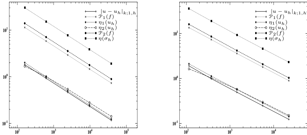
FIG. 2.6: Erreur réelle et estimateurs d'erreur par résidu en fonction du nombre de faces de la triangulation. Gauche : triangulations quasi-uniformes ; droite : triangulations non-uniformes
