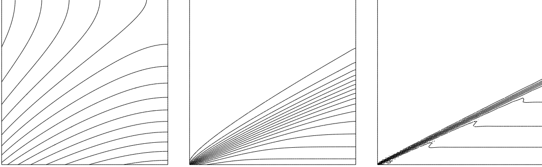
FIG. 4.3: Isovaleurs de la solution approchée, \epsilon = 1 (à gauche); \epsilon = 10^{-2} (au centre); \epsilon = 10^{-4} (à droite) sur la triangulation de taille h_3 .
