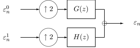
Figure 7.2: Additivité de la distorsion. Sur une étape de décomposition orthogonale, on a \sum_n \varepsilon_n^2 = \sum_n (\varepsilon_n^0)^2 + \sum_n (\varepsilon_n^1)^2 , où \varepsilon_n , \varepsilon_n^0 , et \varepsilon_n^1 désignent les erreurs commises par quantification avant et après décomposition.
