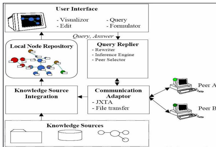
Figure 2.5 : Architecture d'un nœud SWAP [Ehrig et al. , 2003]
