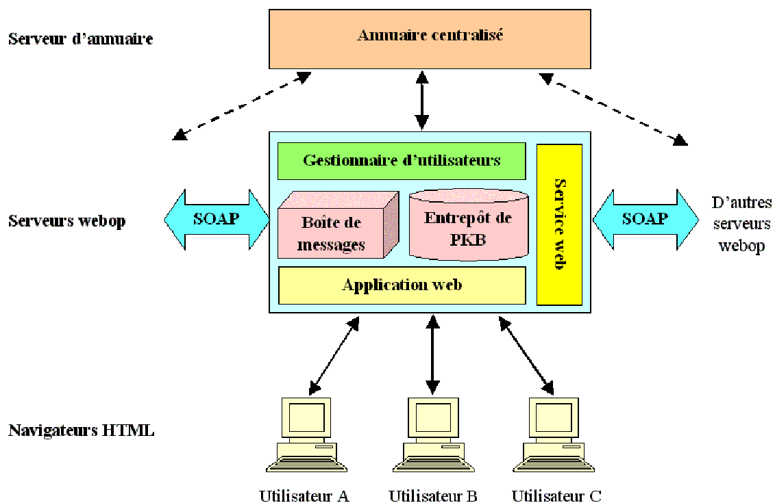
Figure 4.1 : Architecture logicielle du prototype
