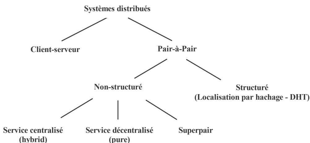
Figure 2.2 : Taxonomie des modèles distribués
