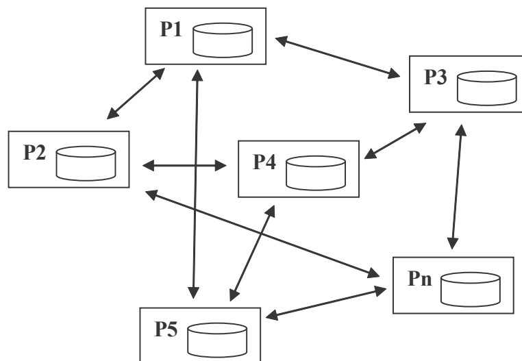
Figure 2.10 : Architecture de médiation de pairs
