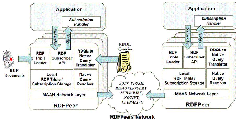
Figure 2.9 : Architecture du réseau RDFPeers [Cai et Frank, 2004]
