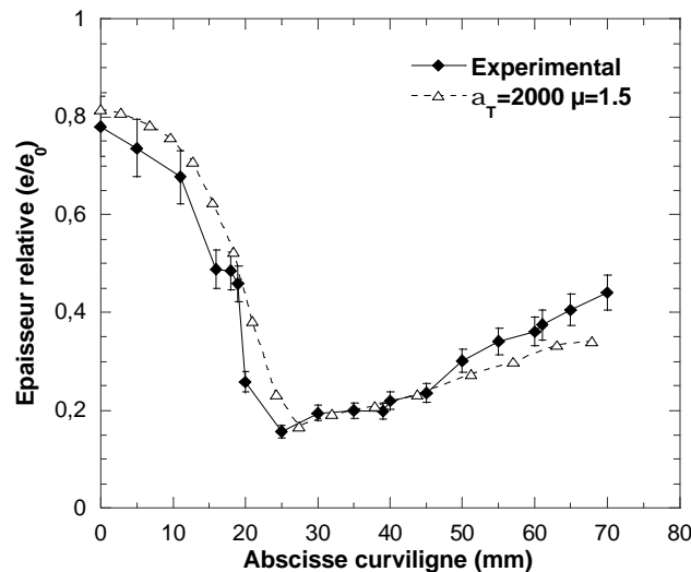
figure VI-17 : Répartitions d'épaisseur en fin de poinçonnage expérimentales et simulées d'une feuille à 147°C avec un poinçon feutre à 20 °C pour un coefficient de frottement de 1.5 ( a_T=2000 W.K^{-1}.m^{-2} ).
