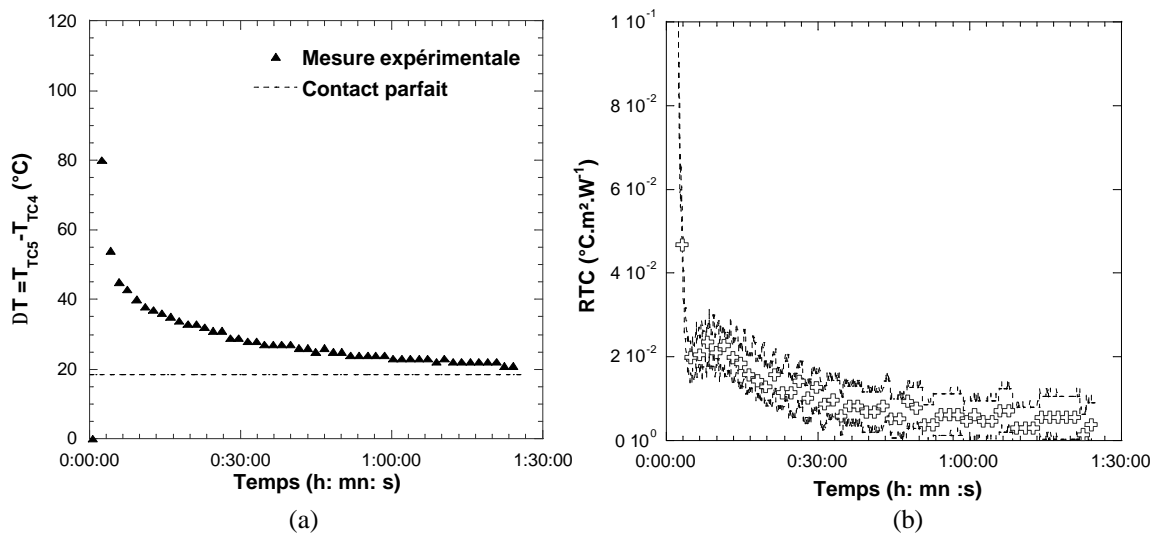
figure IV-5 : Détermination de la RTC aluminium/polystyrène : Evolution de l'écart de température DT entre les thermocouples les plus proches de la surface en fonction du temps (a) ; Evolution de la résistance thermique de contact en fonction du temps avec son enveloppe d'incertitude (b).
