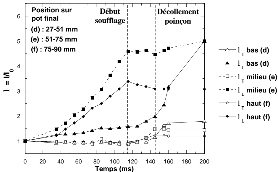
figure III-31 : Taux d'étréage longitudinaux et transverses du bas (d), du milieu (e) et haut (f) du flanc (pour le thermoformage « standard » d'une feuille de température initiale de 145\text{ }^\circ\text{C} avec un poinçon aluminium thermostaté à 120\text{ }^\circ\text{C} ).
