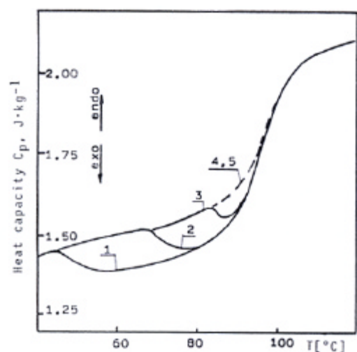
figure II-16 : Analyse DSC à 20\text{ }^{\circ}C \cdot \text{min}^{-1} d'un polystyrène déformé à 13 % par compression uniaxiale (vitesse de sollicitation de 0,001\text{ s}^{-1} ) à différentes températures T_{\text{def}} d'après [36] : (1) : T_{\text{def}} = 25\text{ }^{\circ}C ; (2) : T_{\text{def}} = 65\text{ }^{\circ}C ; (3) : T_{\text{def}} = 80\text{ }^{\circ}C ; (4) : second passage en DSC des échantillons (1), (2) et (3) ; (5) : échantillon non déformé.
