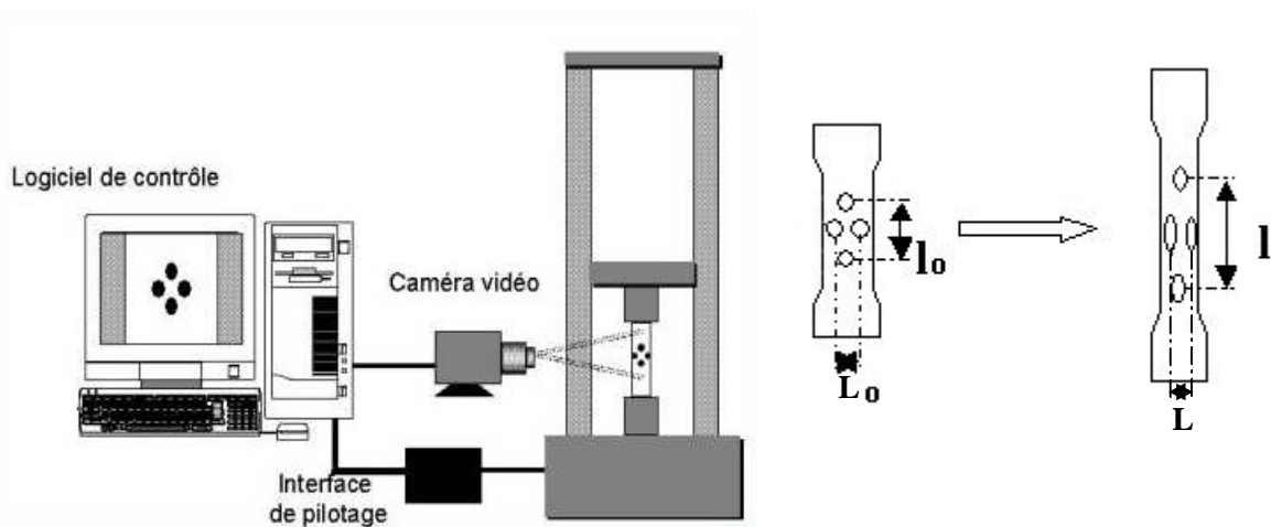
figure IV-4 : Dispositif de pilotage de traction à vitesse de déformation constante via le système Vidéotraction.
