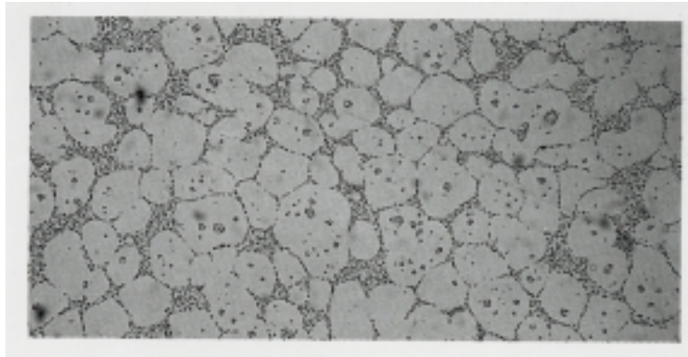
FIG. 3.12 – Microstructure d'un lopin d'A356 avant injection
