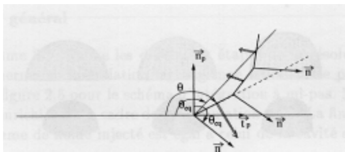
FIG. 4.6 – Situation de non mouillage
