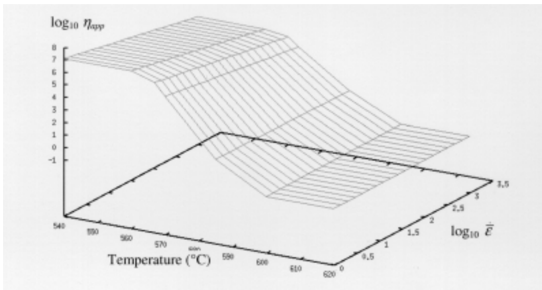
FIG. 3.29 – Evolution de la viscosité apparente identifiée en fonction de la température et de la vitesse de déformation
