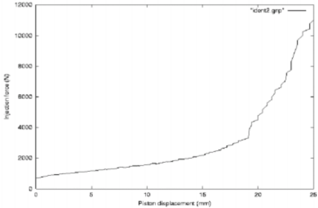
FIG. 3.22 – Courbe typique d'évolution de la force en fonction du déplacement du piston
