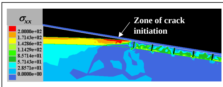
Figure VI-25: Same simulation as Figure VI-24: reduction 45%. The crack initiation zone does not extend. Results are identical to those obtained with a reduction of 35%. Même simulation que Figure VI-24: réduction 45%. Zone de fissuration pas plus étendue. Résultats identiques obtenus avec une réduction de 35%.
