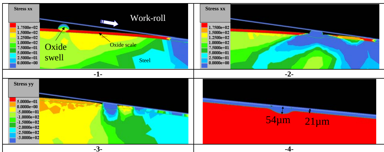
Figure VI-29: Oxide swell evolution in a F2 stand. Surépaisseur d'oxyde dans une cage F2.
