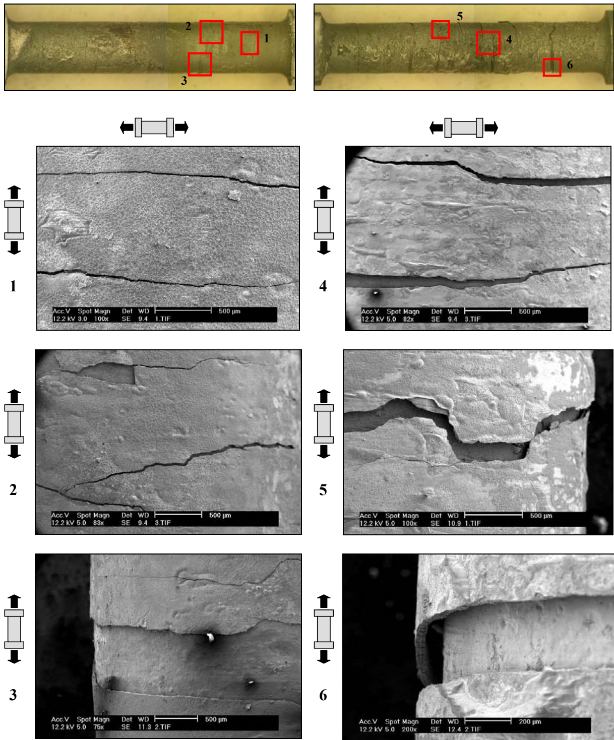
Figure V-13: HTT performed at 800°C and 8 mm.s -1 – Left : elongation=1 mm. Right : elongation=2 mm. TTC réalisés à 800°C et 8 mm.s -1 – Gauche : élongation=1 mm. Droite : élongation=2 mm.
