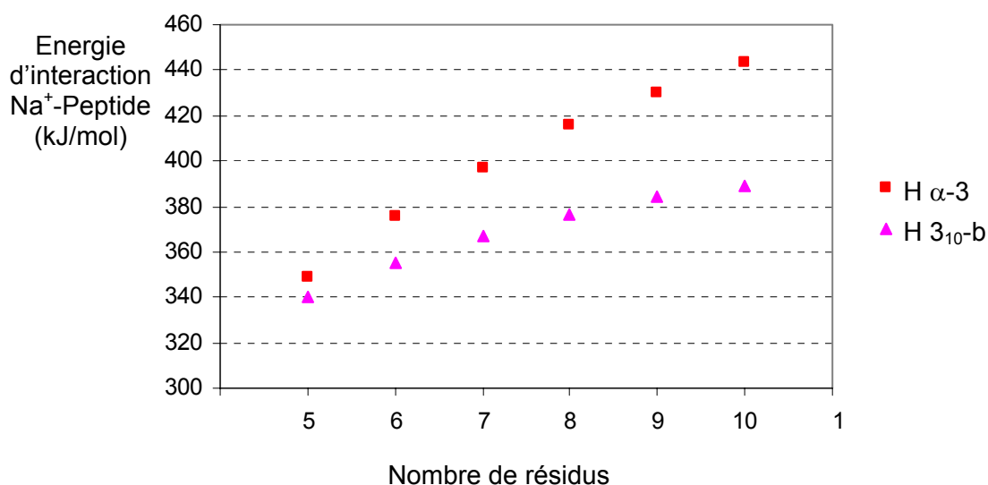
Figure VI-4 : Energies d'interaction métal-peptide pour les structures H α-3 et H 3 10 -b, calculées au niveau ri-BLYP/GB2//ri-BLYP/PB2 en fonction du nombre de résidus n de Gly n -Na + .
