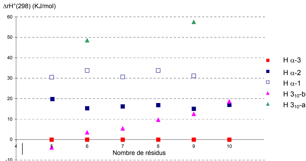
Figure VI-3 : Enthalpies standards de conformation à 298 K des différentes hélices relatives à celle de la structure hélice H α-3, calculées au niveau ri-BLYP/GB2//ri-BLYP/PB2, en fonction du nombre de résidus n de Gly n -Na + .
