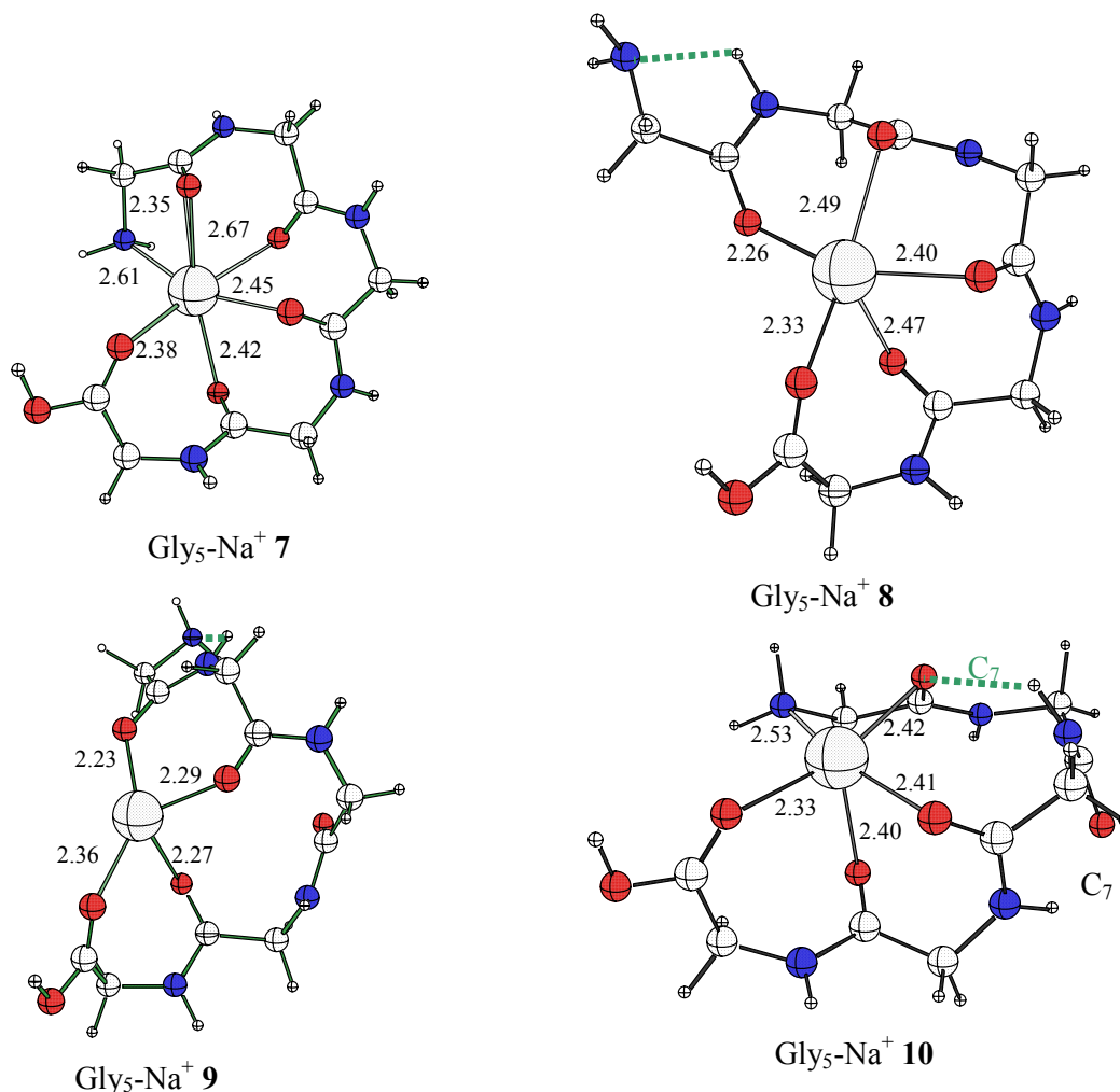
Suite Figure VI-7 : Conformères de plus basse énergie de Gly 5 -Na + .
