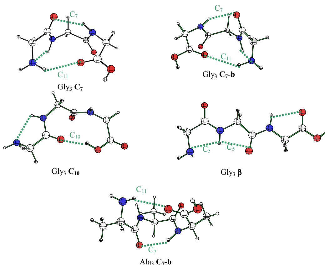
Figure V-13 : Structures de Gly 3 les plus basses en énergie et structure de Ala 3 la plus basse en énergie.
