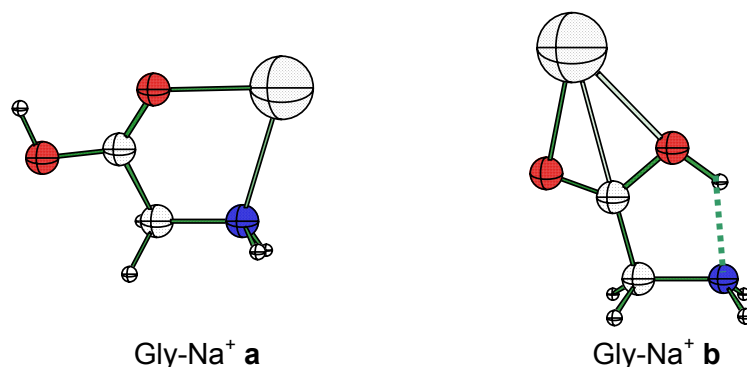
Figure III-7 : Structures des isomères Gly-Na + a et b
