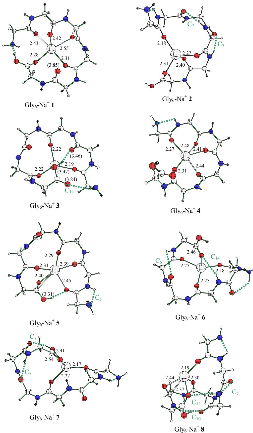
Figure VI-8 : Conformères de plus basse énergie de Gly 6 -Na + .
