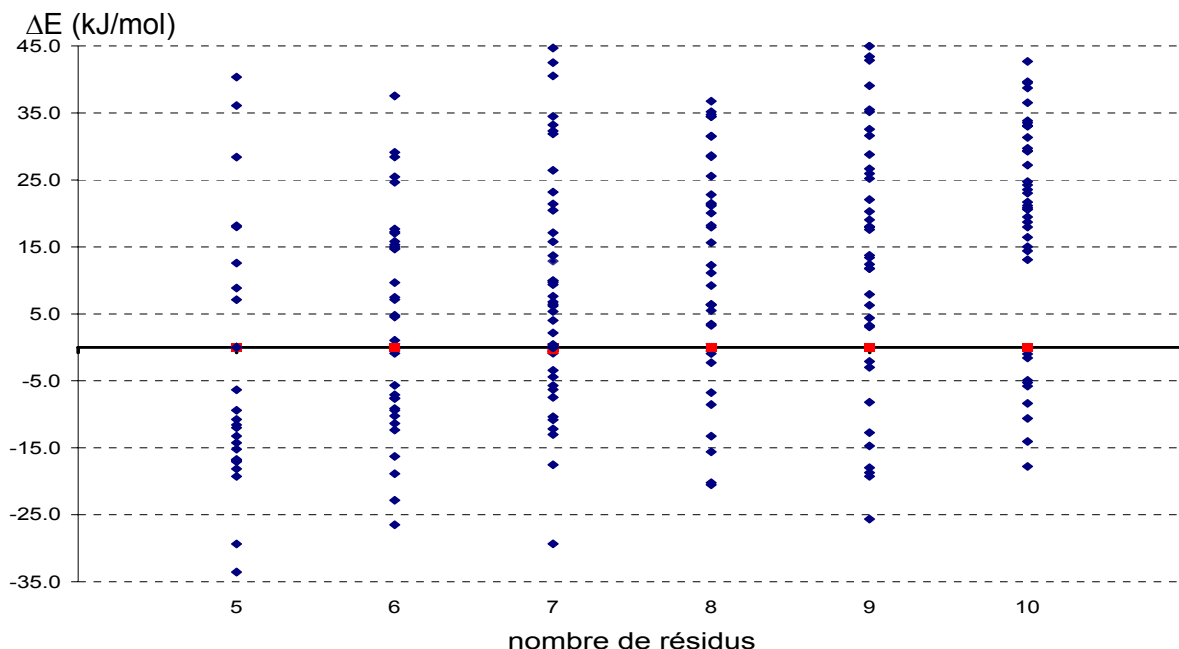
Figure VI-5 : Energies des conformères globulaires relatives à celle de la structure en hélice H α-3, calculées au niveau ri-BLYP/GB2//ri-BLYP/PB2 en fonction du nombre n de résidus de Gly n -Na + .
