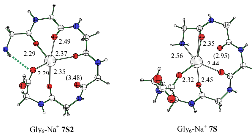
Figure VI-13 : Structures des conformères complémentaires de Gly 6 -Na + .
