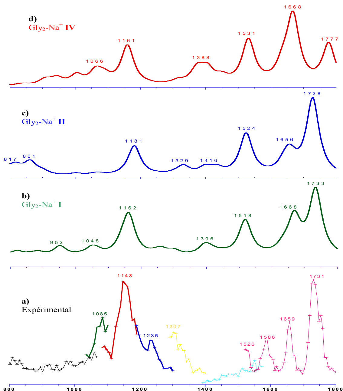
Figure V-8 : (a) Spectre IRMPD de Gly 2 -Na + , (b-d) spectres IR des conformères de plus basse énergie calculés au niveau B3LYP/6-31G*.
