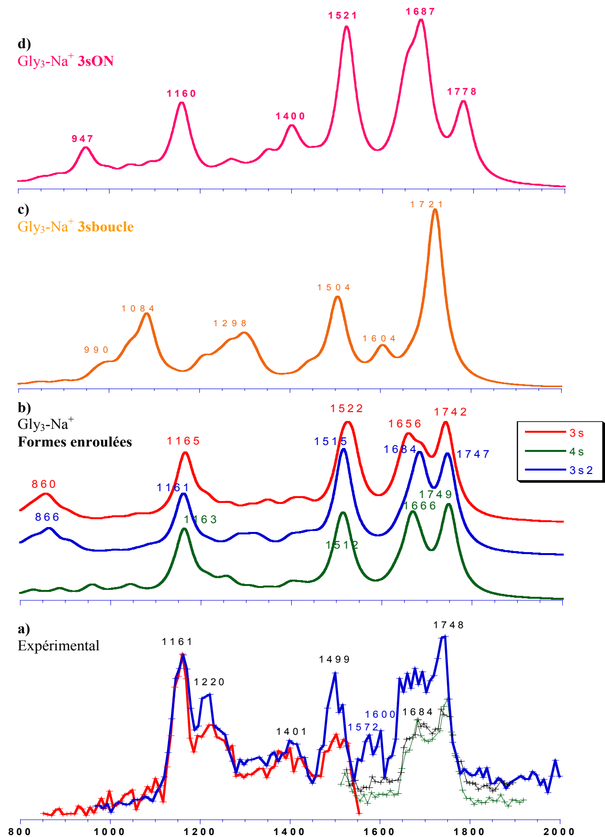
Figure V-9 : (a) Spectre IRMPD de Gly 3 -Na + , (b-d) spectres IR des conformères de plus basse énergie calculés au niveau B3LYP/6-31G*.
