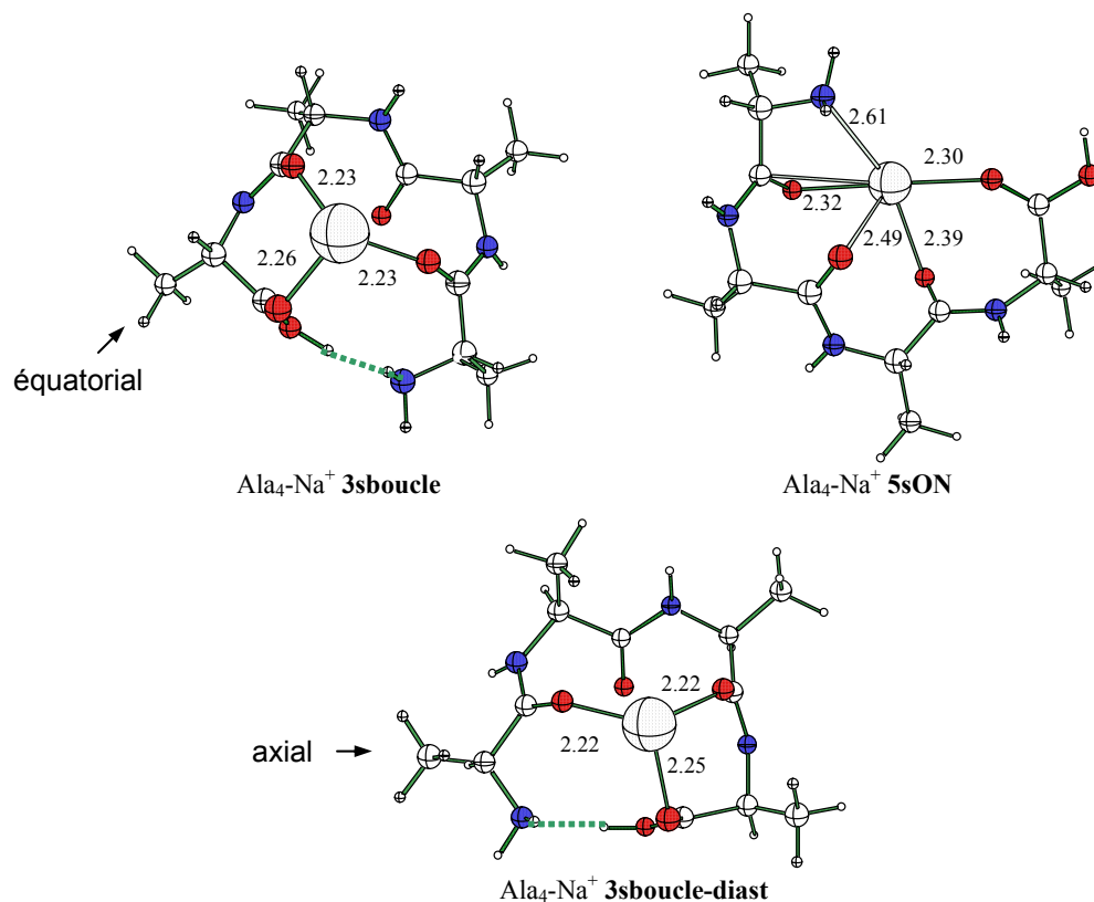
Figure V-6 : Structures des diastéréoisomères les plus bas en énergie de Ala 4 -Na + .
