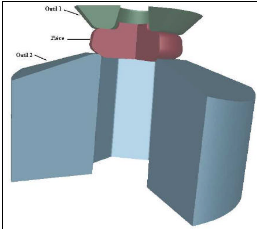
Figure 31 : Vue en coupe du cas du Trinity Colleague
