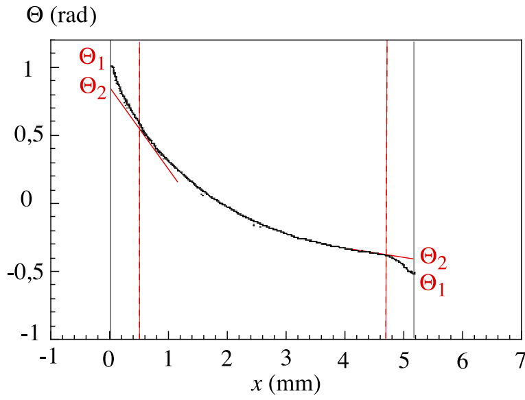
FIG. 3.7 – On voit ici la différence entre les mesures obtenues en utilisant la méthode laser ( \Theta_1 ) et la méthode des cercles ( \Theta_2 ). A l'avant comme à l'arrière de la goutte on note que \Theta_1 \geq \Theta_2
