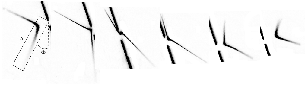
FIG. 2.4 – Différentes figures de réfraction observées lors du passage de la goutte dans le plan laser.
