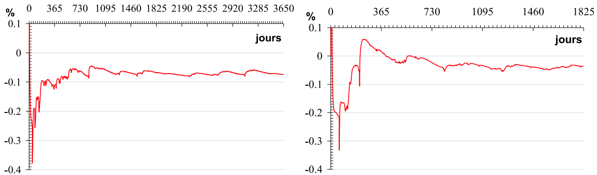
FIG. 7.7: Erreur relative en % calculée sur les cumulés. A gauche résultats du calage, à droite résultats de la validation.
