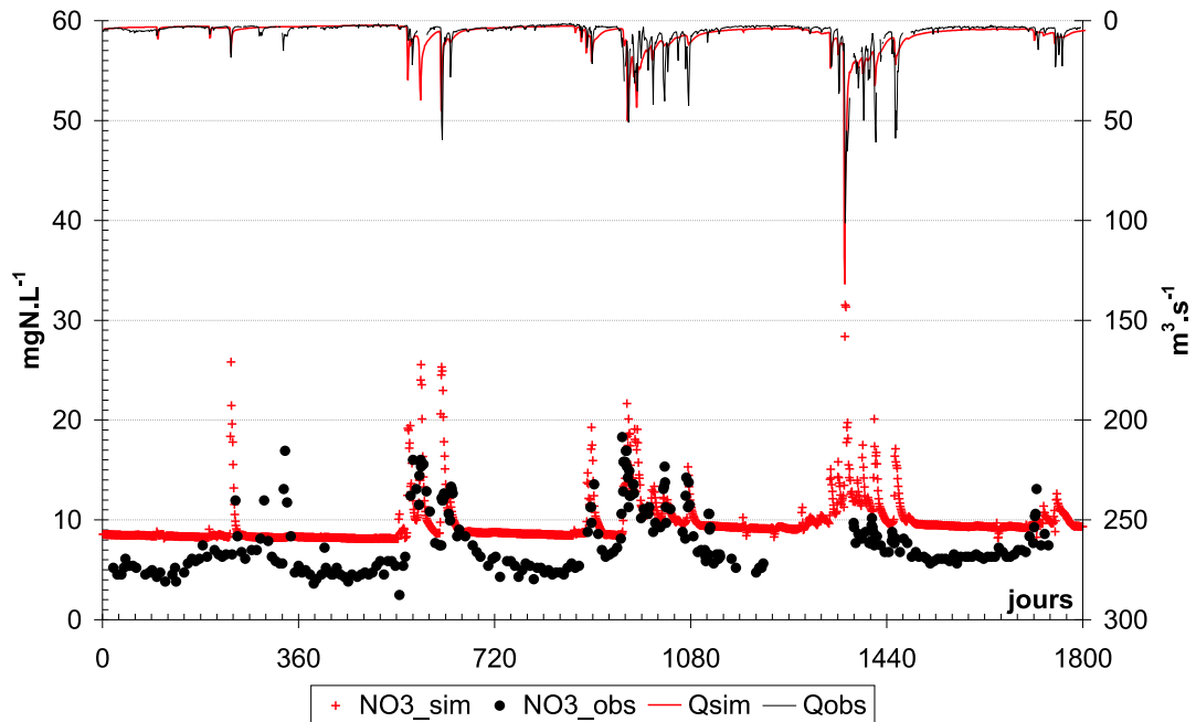
FIG. 12.4: Concentrations simulées et observées à Villiers (1 150 km 2 ). 1 er mai 1991 - 5 avril 1996.
