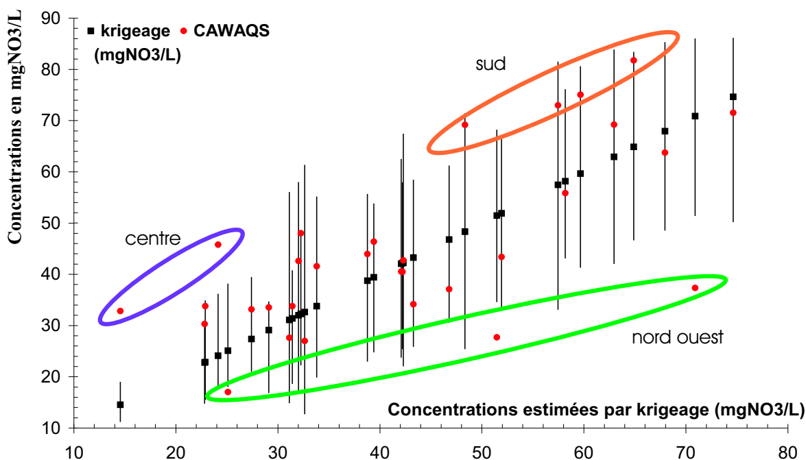
FIG. 10.5: Ecarts, aux points de contrôle, entre CAWAQS et le krigage pour l'Eocène en 1988. Les barres noires représentent l'intervalle de confiance à 95 % estimé par krigage.
