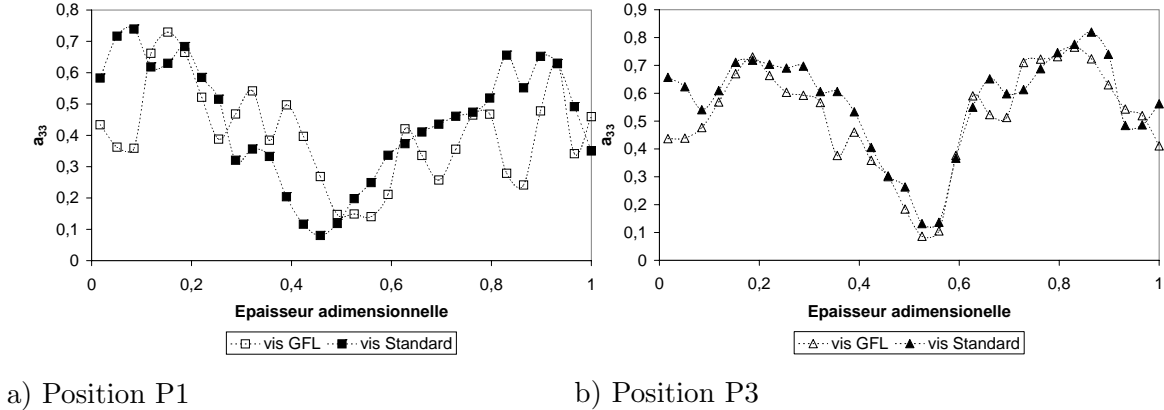
FIG. 1.41 – Influence de la vis d'injection sur l'orientation moyenne 3D des fibres pour les composantes a_{33} du tenseur \mathbf{a}_2 -pp30%fv12 injecté avec une vis standard et une vis GFL-
