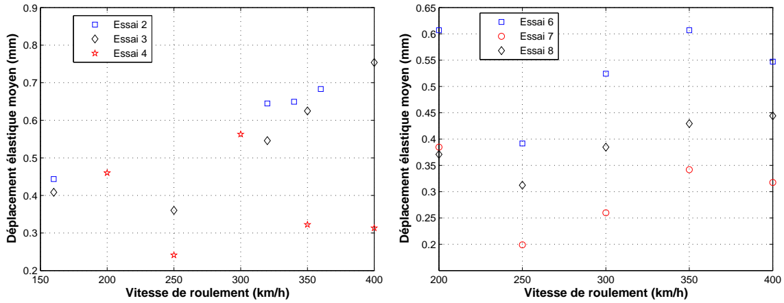
FIGURE 2.27. Déplacement élastique en fonction de la vitesse de roulement (Essais avec une plate-forme raide)
