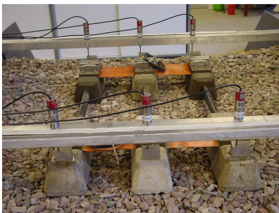
FIGURE 3.32. Mise en place des capteurs de déplacement (LVDT) sur les blochets
