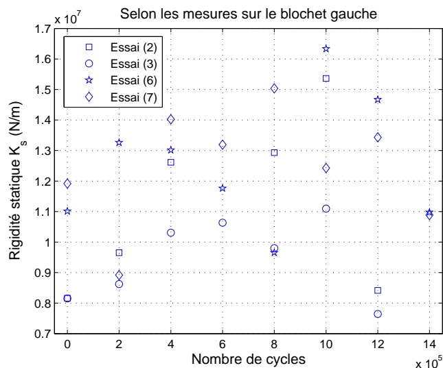
FIGURE 4.8. Rigidité statique du système complet
