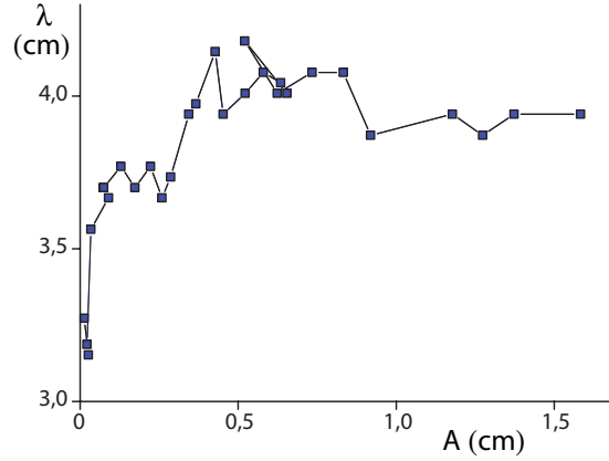
FIG. 5.43 – Longueur d'onde \lambda en fonction de l'amplitude A (air, d = 300\mu m , \theta = 35^\circ ).
