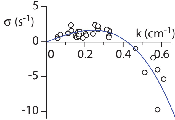
FIG. 5.52 – Taux de croissance temporel \sigma en fonction du nombre d'onde k (air, d = 300 \mu\text{m} , \theta = 35^\circ ). La courbe continue est le meilleur ajustement de la forme \sigma = \sigma_m |k| \lambda_0 (1 - (k \lambda_0)^2 / 3) , avec un taux de croissance maximum \sigma_m \approx 2,5 \text{ s}^{-1} pour \lambda_0 \approx 4 \text{ cm} .
