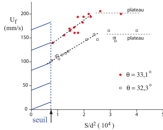
FIG. 5.18 – Vitesse des ondes en terme de volume linéique de grains piégés représentée pour deux angles distincts ( \theta = 32,3^\circ , \theta = 33,1^\circ ).
