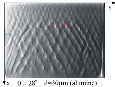
FIG. 6.4 – Ecoulement perturbé par la présence de défauts (points rouges).
