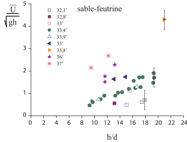
FIG. 4.14 – Mesure de la vitesse moyenne des écoulements stationnaires uniformes en fonction de l'épaisseur h et de l'angle d'inclinaison \theta pour le sable de Fontainebleau sur de la feutrine. La vitesse est adimensionnée par \sqrt{gh} en fonction de h/d
